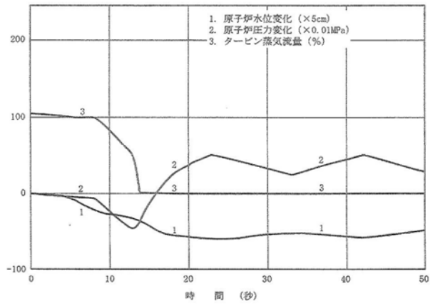
図2 (参考) 給水流量の全喪失時の過渡変化解析結果 (A型/B型の比較)
