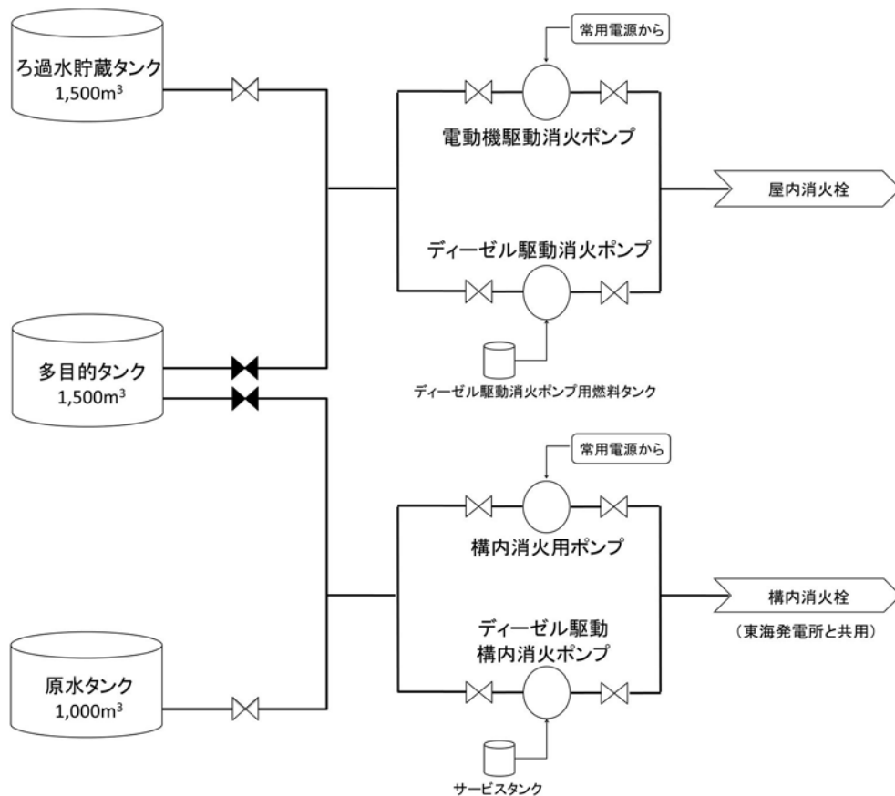
第1-22図 屋内及び構内(屋外)消火用水供給系の概要
