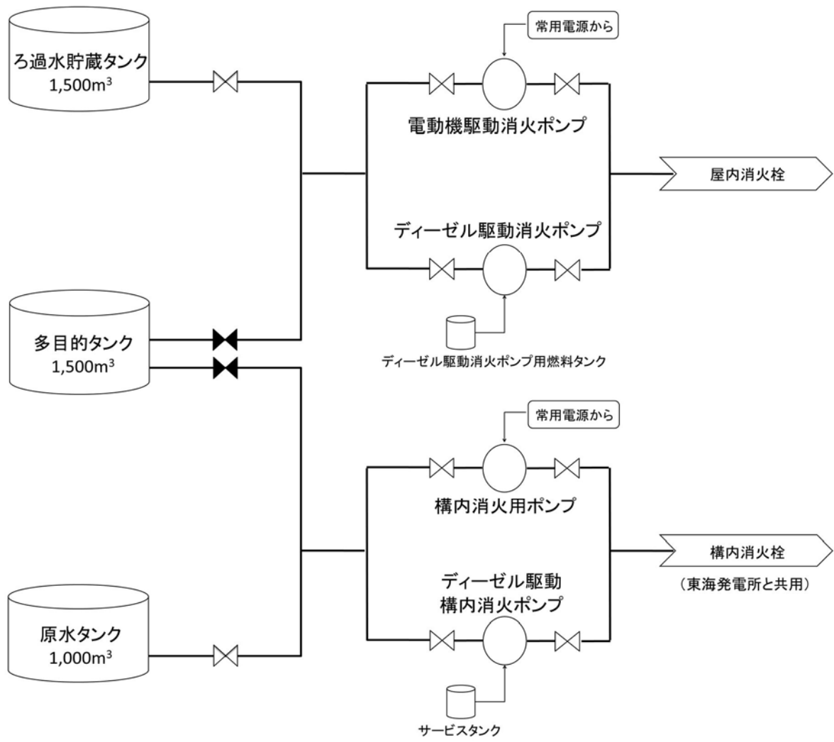
第 10.5-2 図 屋内及び構内消火栓設備の系統構成
