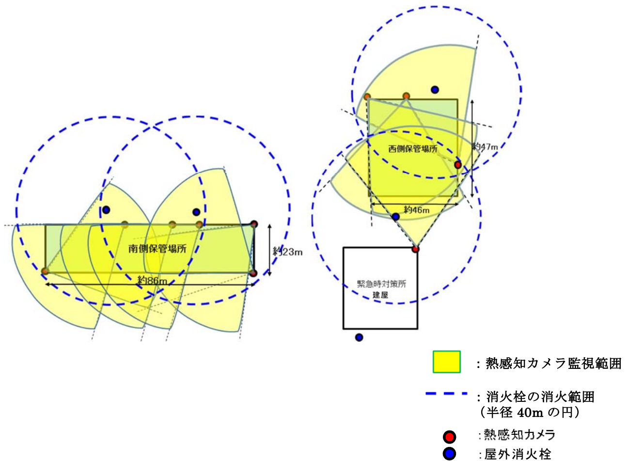
第 1-45 図 屋外の可搬型重大事故等対処設備保管場所の感知設備， 消火設備
