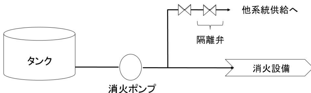
第1-29 消火用水供給系の優先供給の概略図
