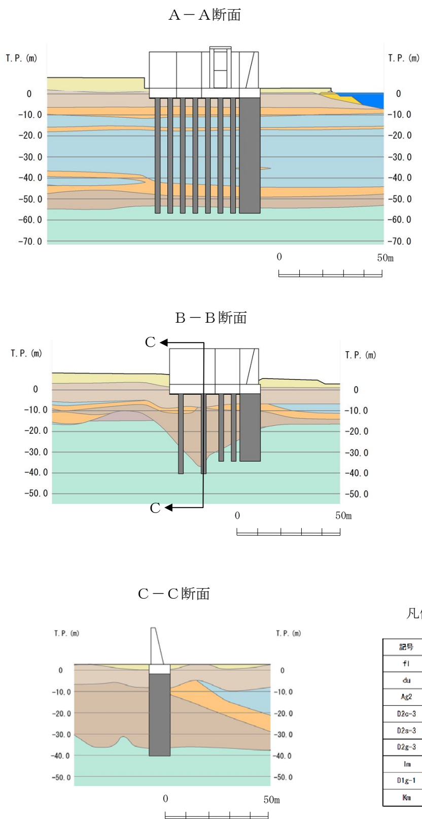
第3-7図 側方流動の評価範囲 (2/2)
