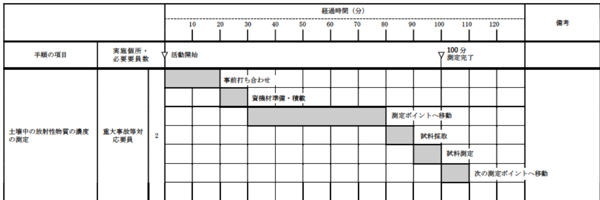
第1.17-9図 土壌中の放射性物質の濃度の測定のタイムチャート
