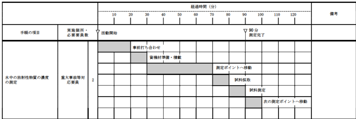
第1.17-8図 水中の放射性物質の濃度の測定のタイムチャート
