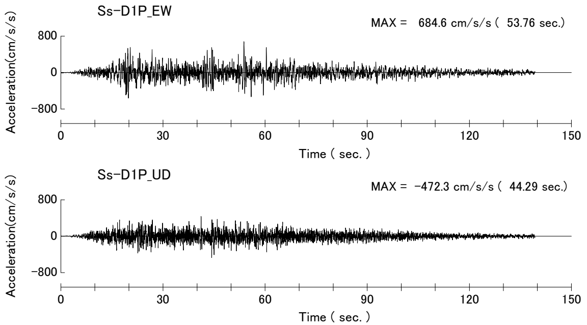
図 4-3 入力地震動の加速度時刻歴波形 (S s -D1) (地盤物性のばらつきを考慮 (+1σ))
