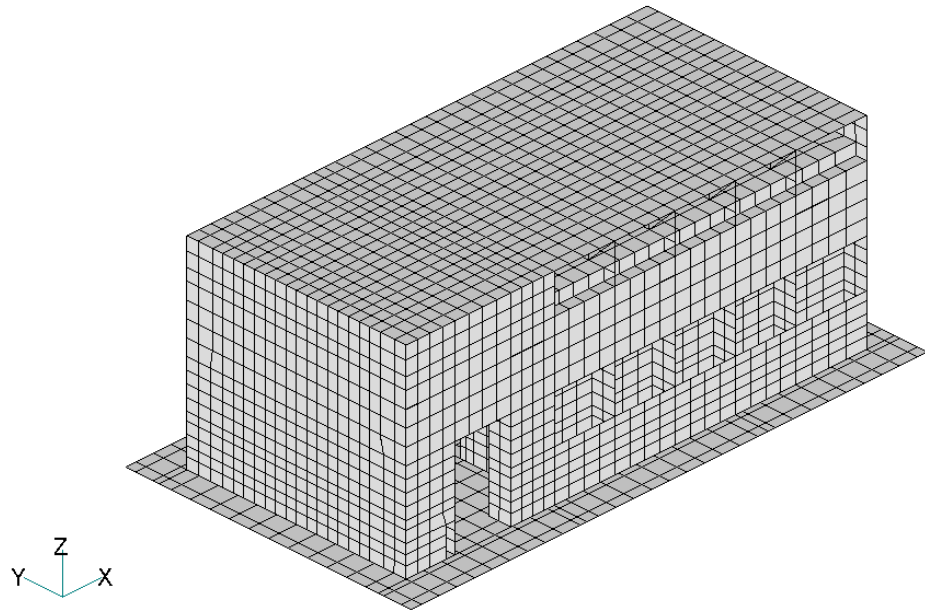
(シェル要素)
