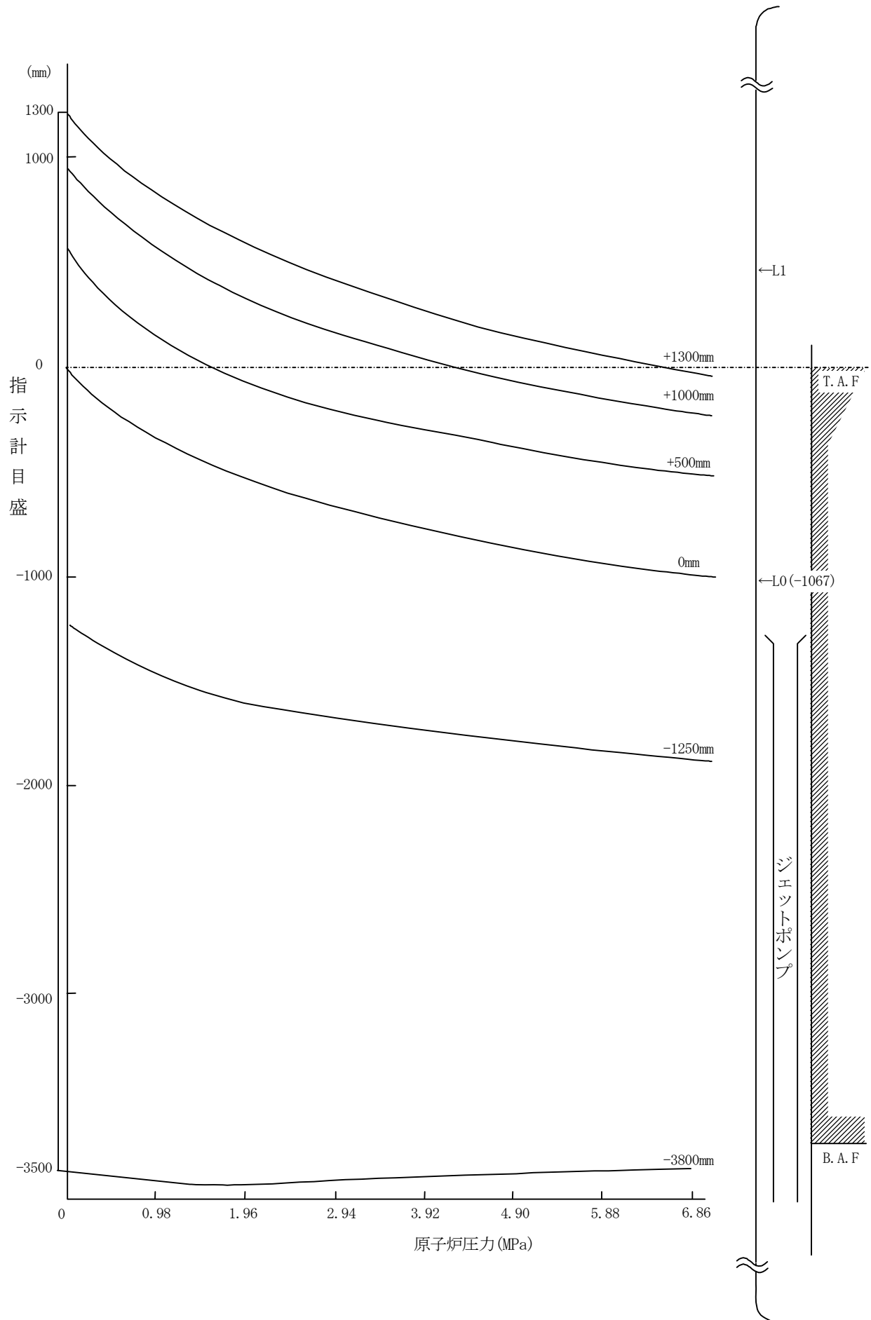
図3 燃料域計補正曲線 (原子炉圧力変化)
