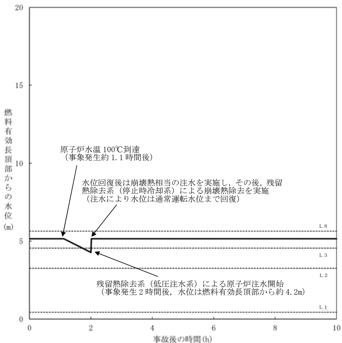
第7.4.1-4図 原子炉水位の推移
