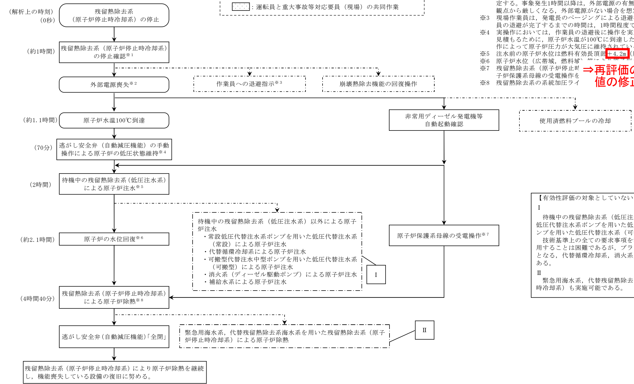
第 7. 4. 1-2 図 崩壊熱除去機能喪失時の対応手順の概要
