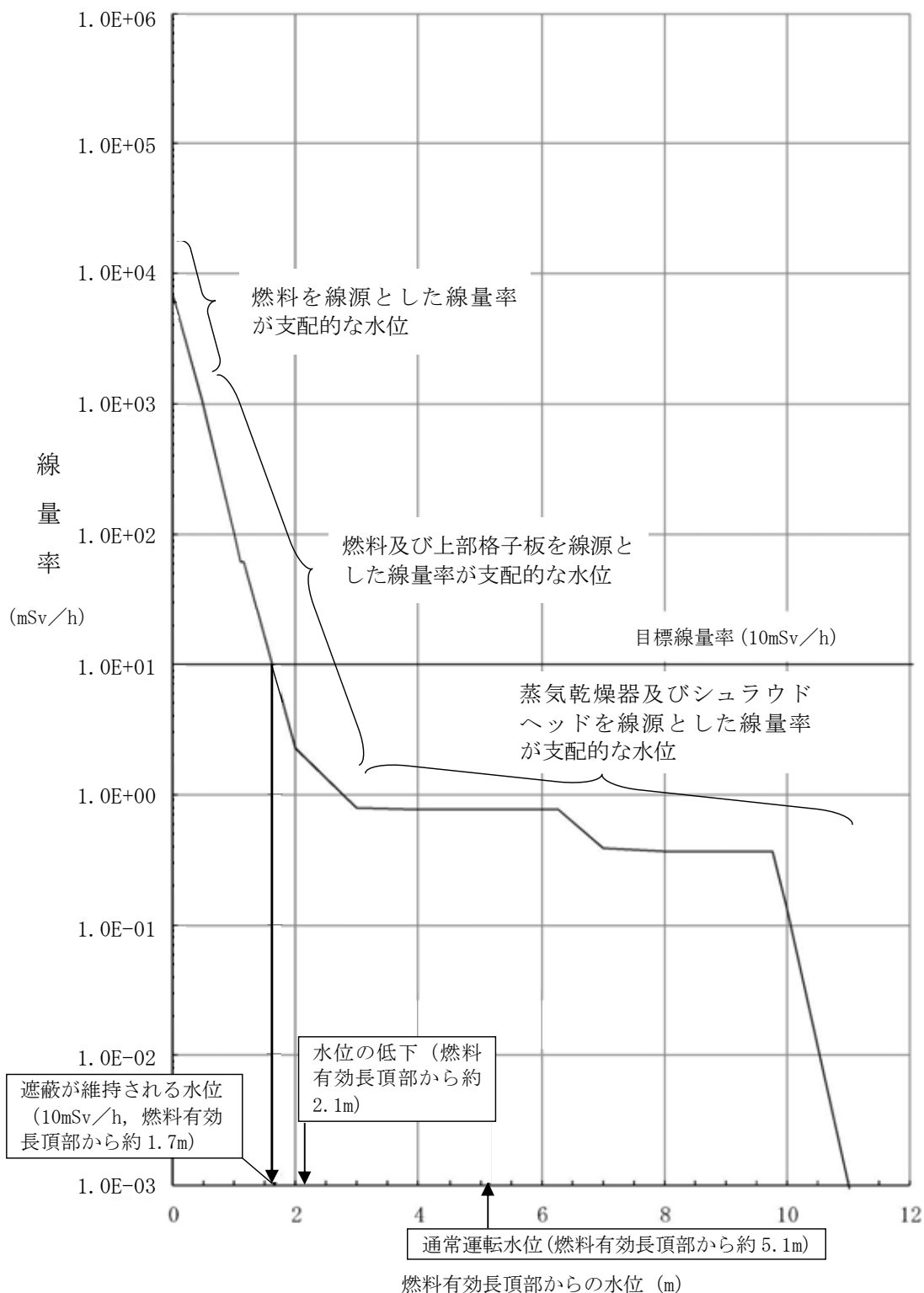
第7.4.3-5図 原子炉水位と線量率
