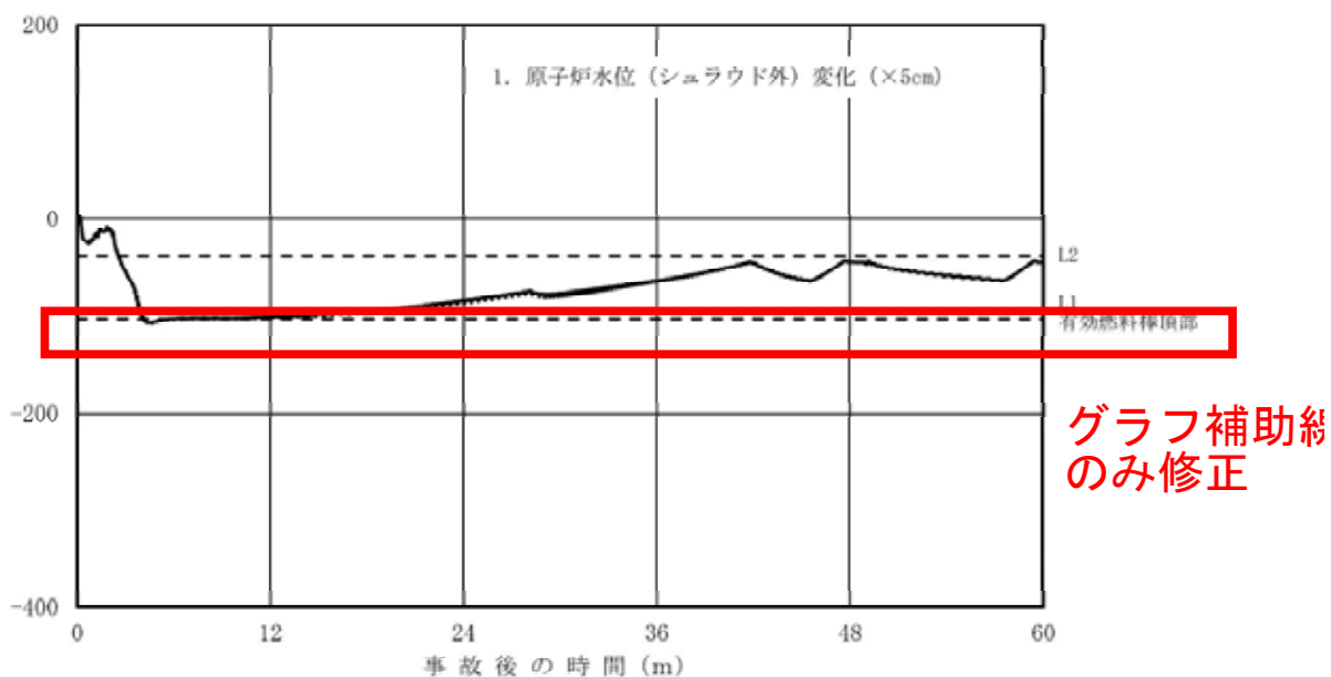
第 4 図 原子炉水位の水位 (60 分まで)
