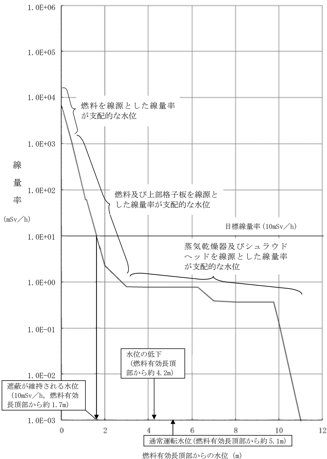
第7.4.1-5図 原子炉水位と線量率
