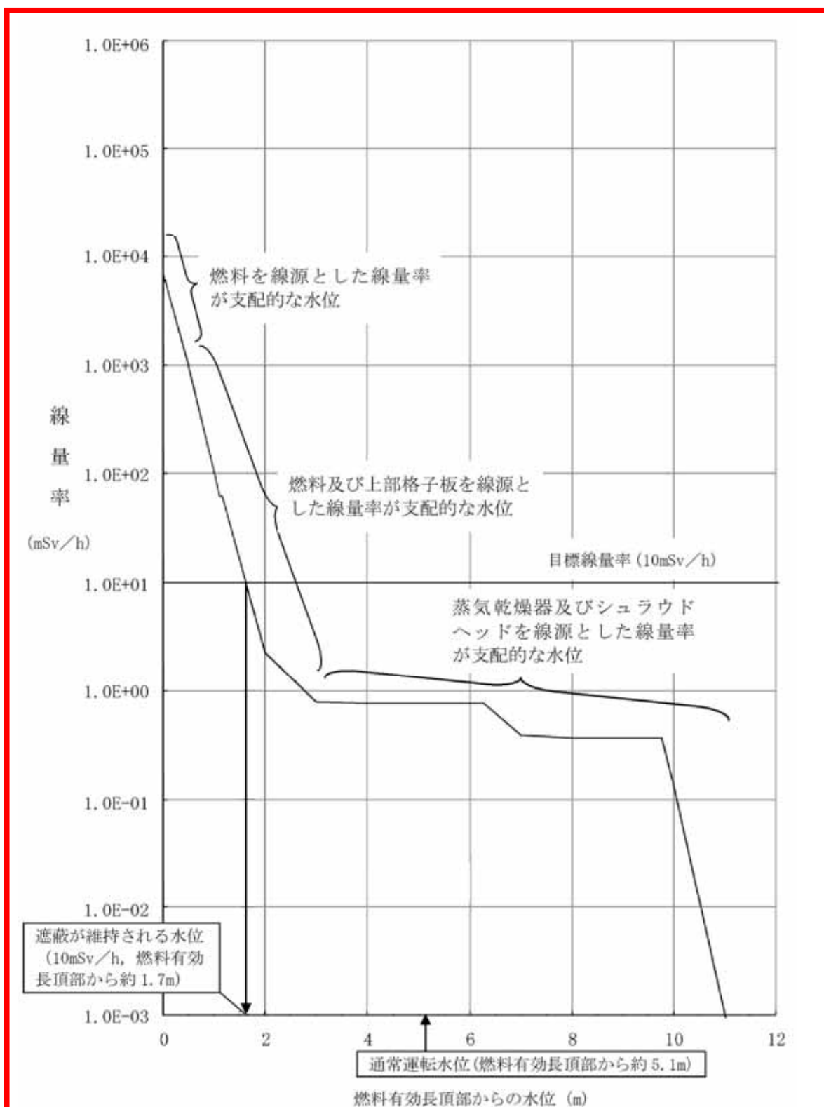
第 7. 4. 2-5 図 原子炉水位と線量率
