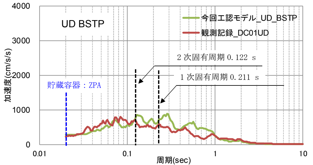
図1 (3/3) 床応答スペクトルの比較 (上下方向, h=5%)
