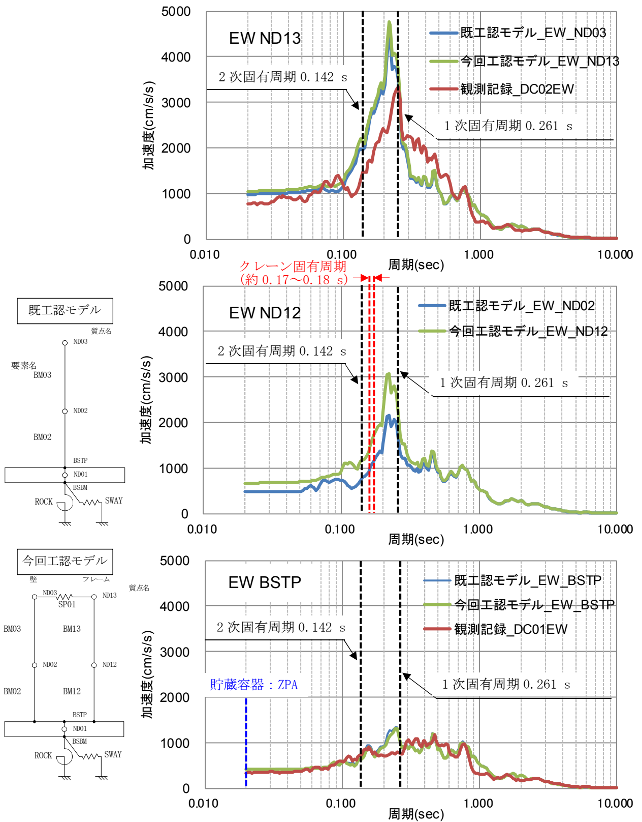
図 1 (2/3) 床応答スペクトルの比較 (EW方向, h=5%)
