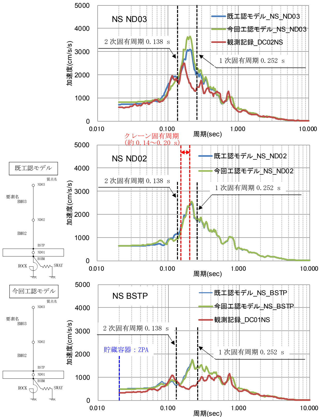
図1 (1/3) 床応答スペクトルの比較 (NS方向, h=5%)
