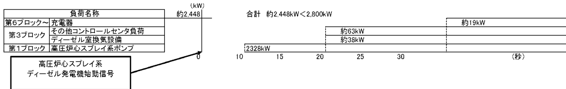
第 2.3.1.2-3 図 高圧炉心スプレイ系ディーゼル発電機の負荷の始動順位 (外部電源喪失及び原子炉冷却材喪失時)
