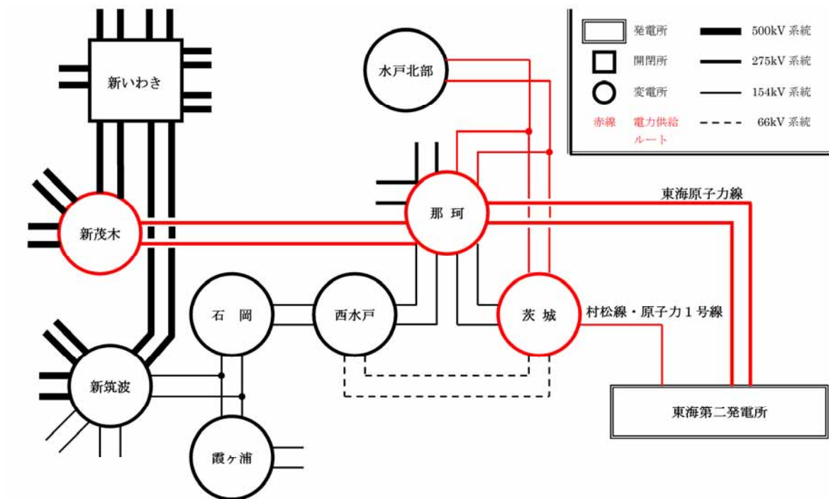
第 2.2.2.1-1 図 送電系統図
