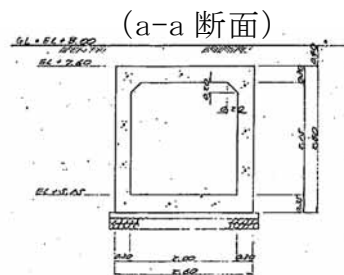
第 2.2.4.4-2 図 275kV 超高圧開閉所から東海第二発電所にかけてのケーブル洞道基礎図
