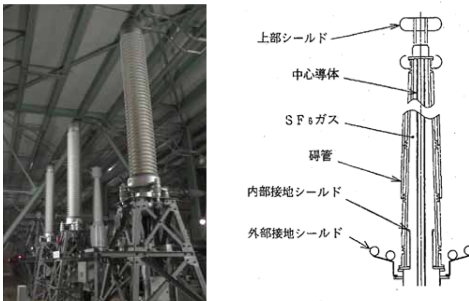
第 3 図 ブッシングの外観及び内部構造部の例
