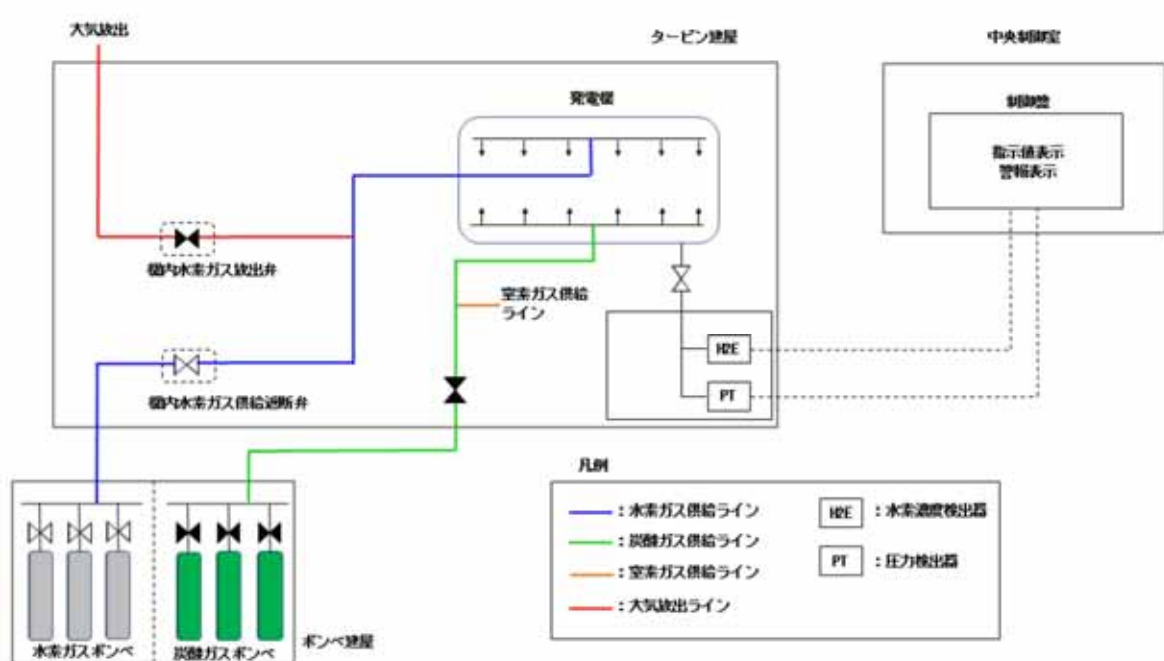
第 1-3 図 発電機水素漏えい防止設備の概要
