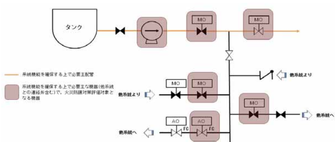
第2-4図 機器の抽出の考え方
