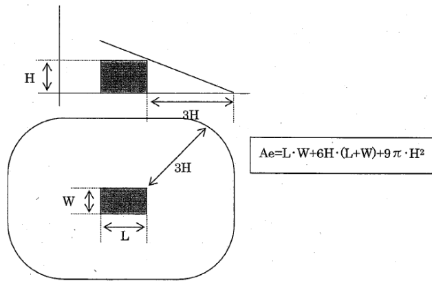
図 要素 Ae (構造物の等価受雷面積)
