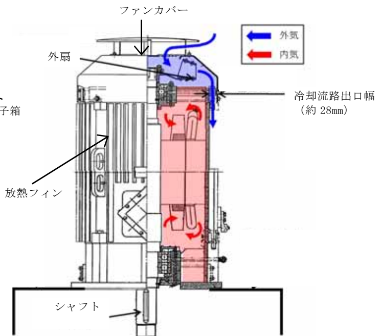
第2.4.2-7図 非常用ディーゼル発電機（高压炉心スプレィ系ディーゼル発電機を含む。）用海水ポンプ電動機 構造図
