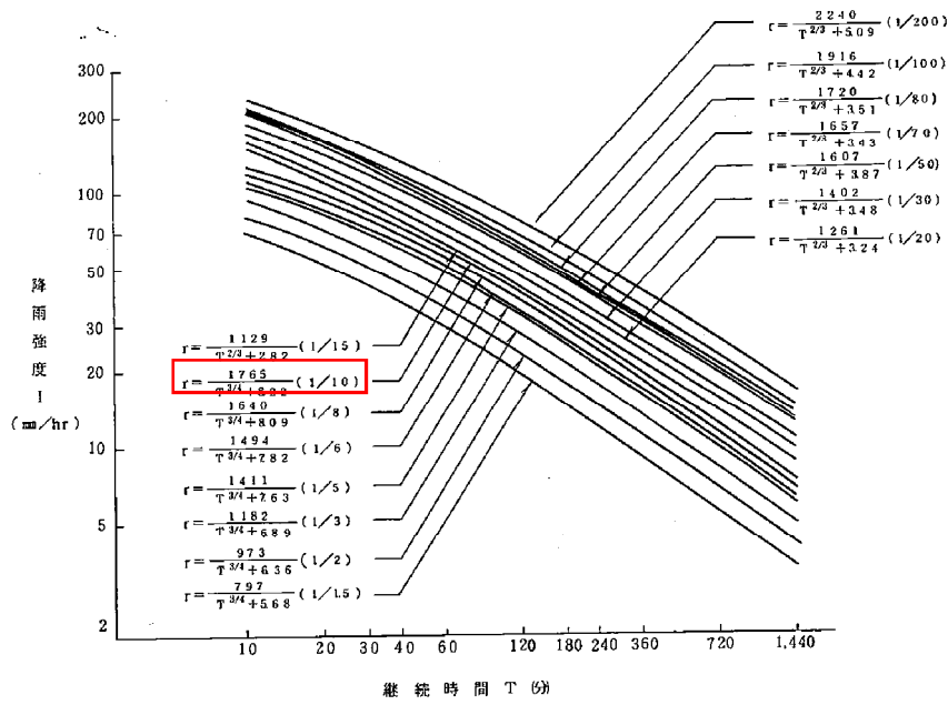
図 水戸降雨強度曲線 (トーマス法)
