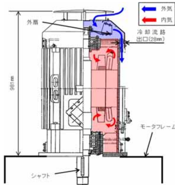
第 8 図 非常用ディーゼル発電機（高压炉心スプレィ系ディーゼル発電機を含む。）用海水ポンプ電動機の冷却方式
