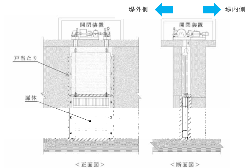
図4 防潮扉の概要図
