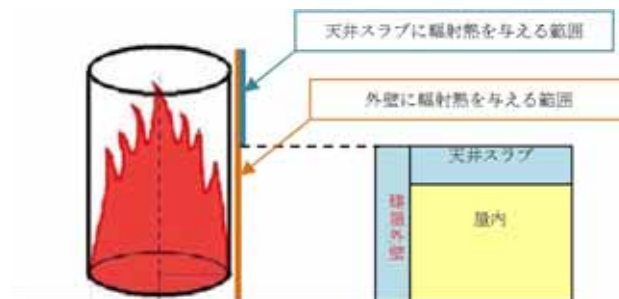
第 4.3.2.1-4 図 天井スラブへの輻射熱の影響概念図
