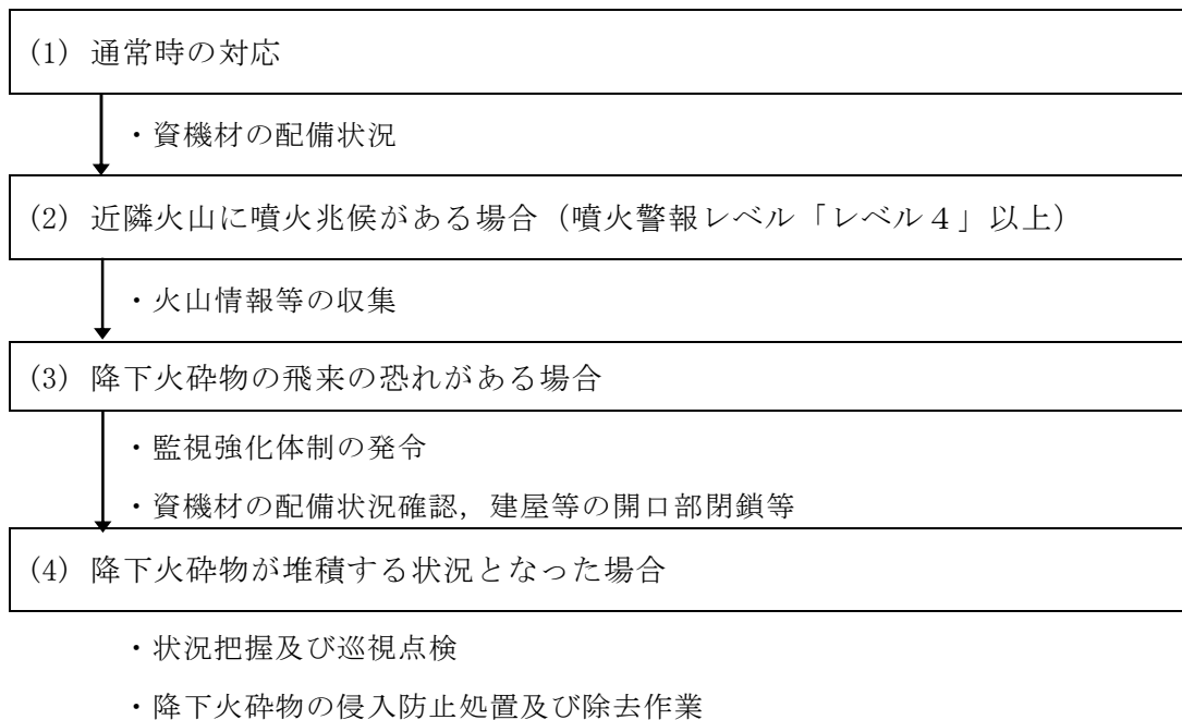
第 3.7.1-1 図 降下火砕物に対応するための運用管理フロー
