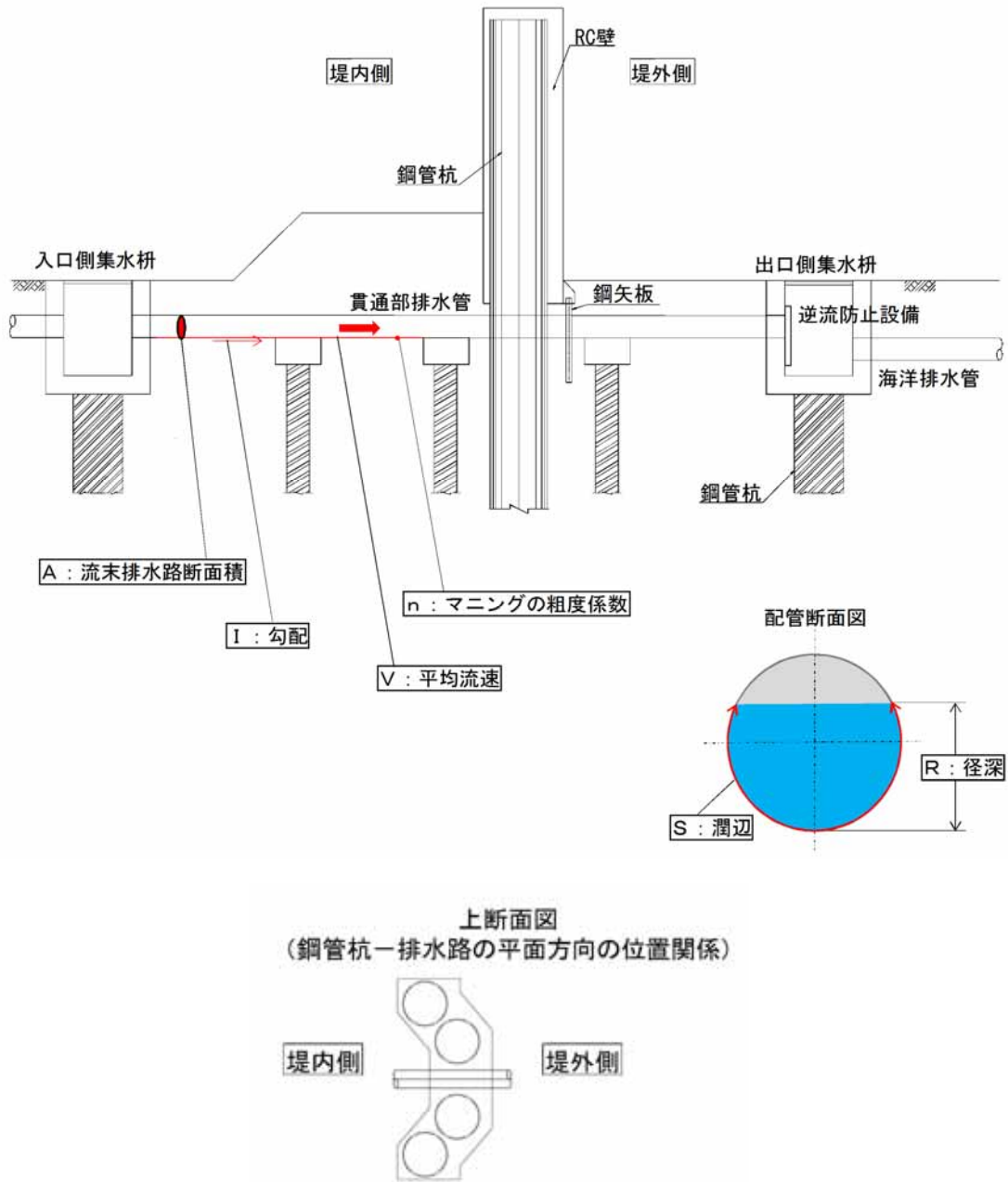
第2図 流末排水路構造 (案)
