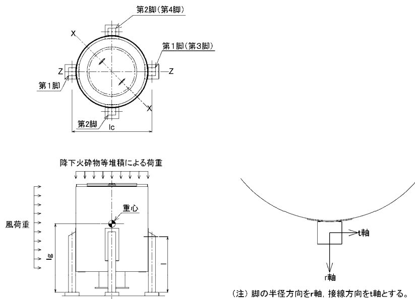
第3図 ディーゼル発電機吸気フィルタ モデル図
