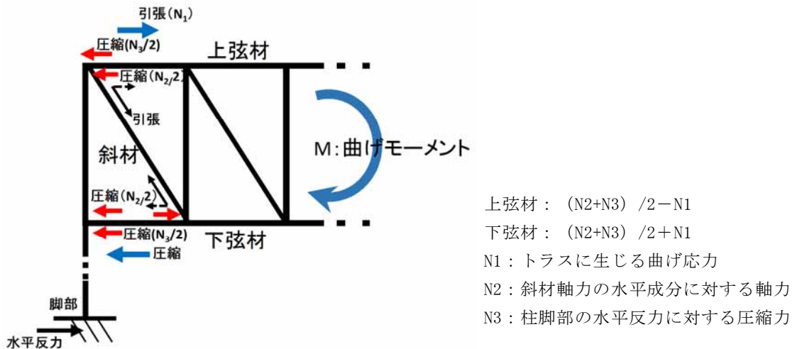
第 4-1 図 発生応力の概略図
