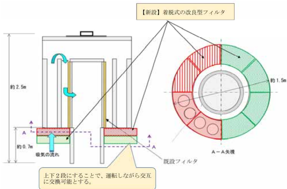
非常用ディーゼル発電機（高圧炉心スプレイ系ディーゼル発電機を含む。）吸気フィルタ（既設）へ着脱式フィルタを取付
