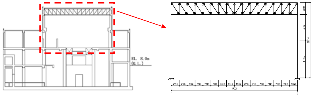
第 3-1 図 タービン建屋断面図（NS 側）及び主トラス検討モデル
