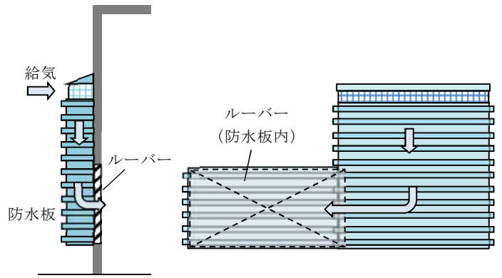
第2図 ディーゼル駆動消火ポンプ室給気口
