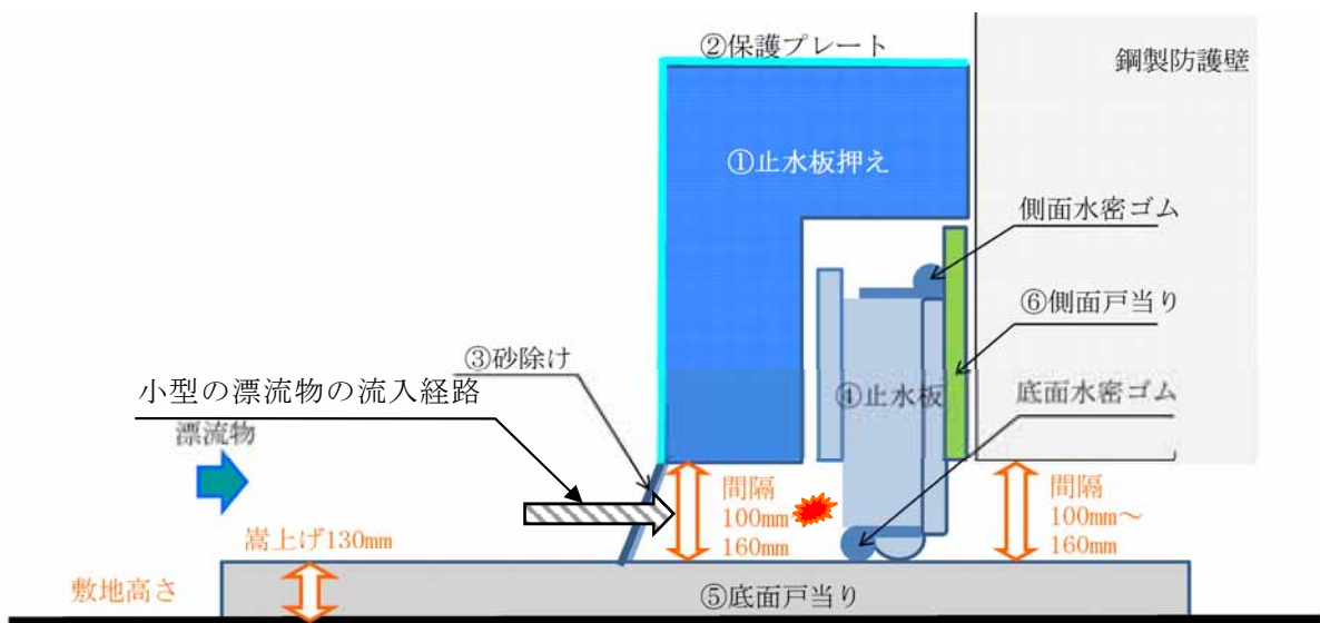
第 1-53 図 小型漂流物の流入経路
