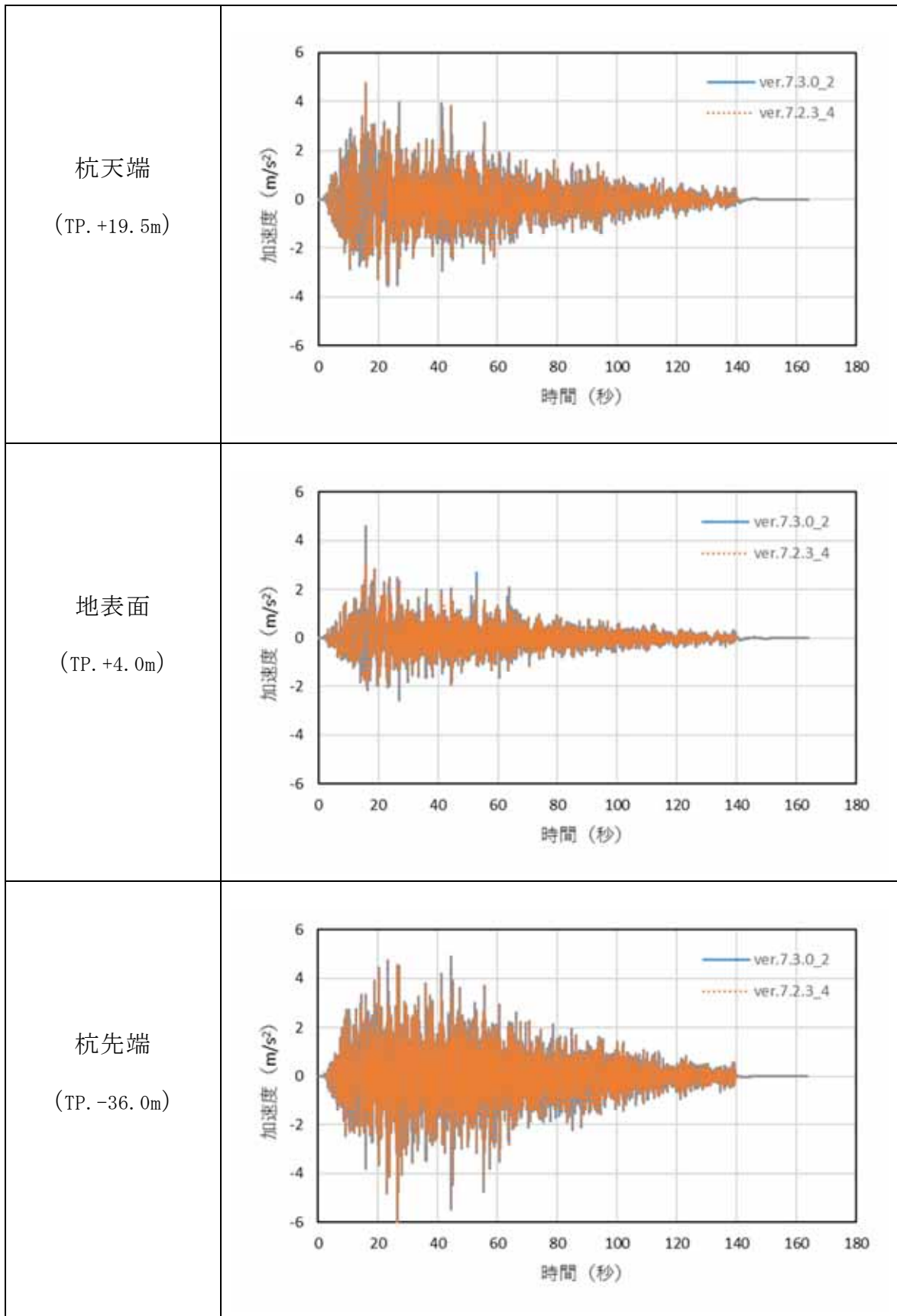
図 2 水平方向加速度 ( \text{m/s}^2 ) (杭軸方向非線形バネを無視した場合)
