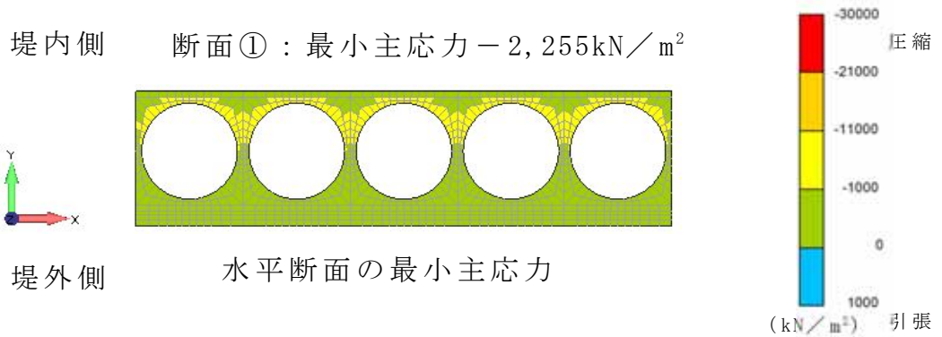
第 3-80 図 津波時+漂流物の解析結果（最小主応力分布）
