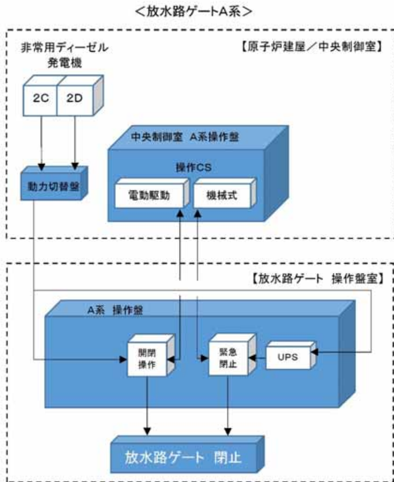
第10図 放水路ゲート電源概念図（A系の例）
