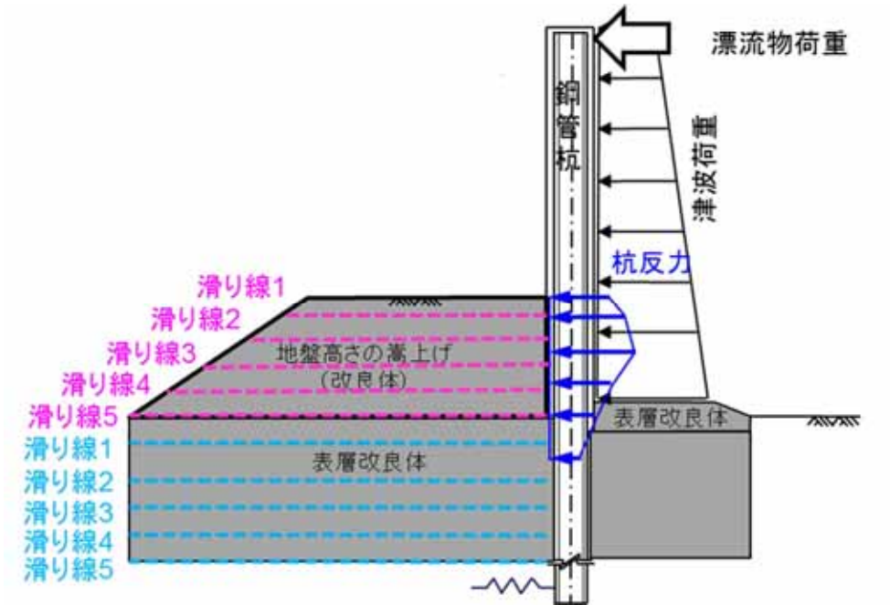
第 3-88 図(1) 滑り線の模式図
