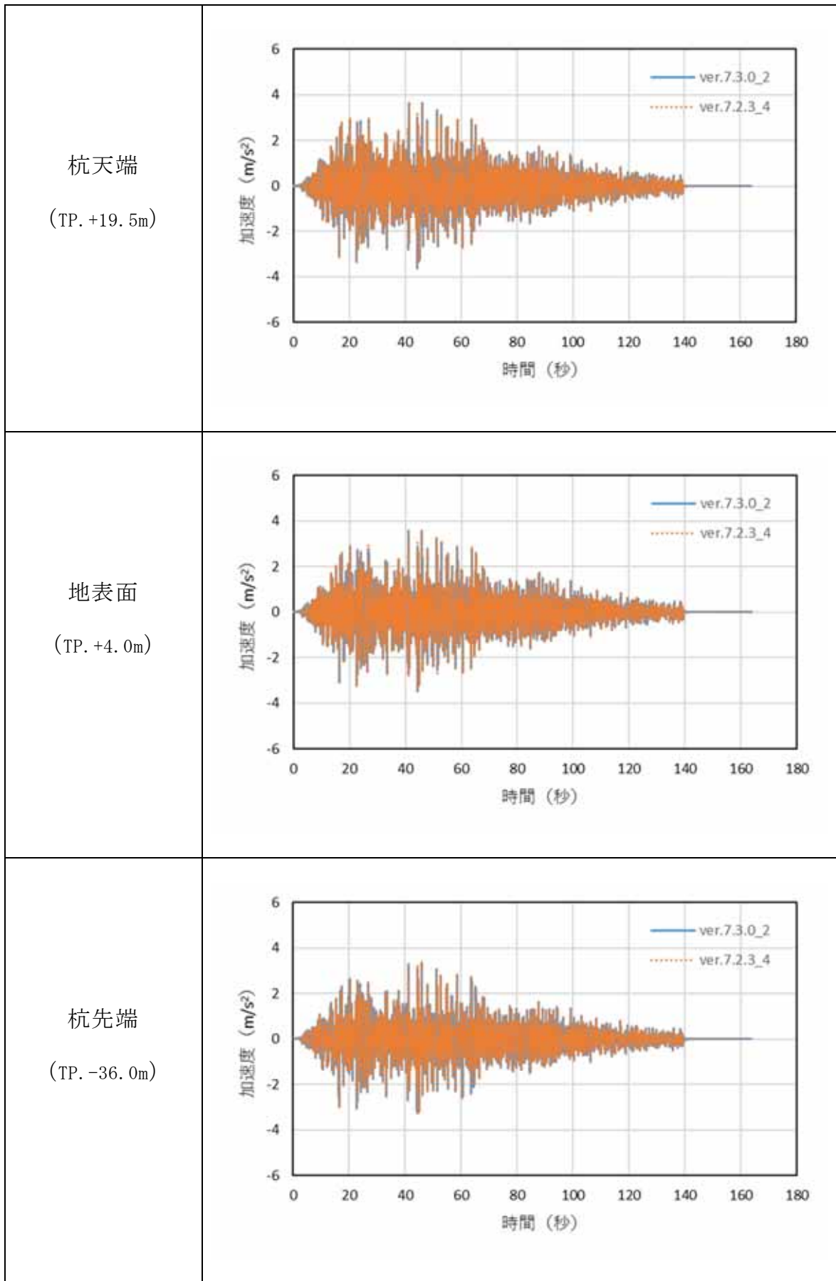
図 5 鉛直方向加速度 ( m/s^2 ) (杭軸方向非線形バネを考慮した場合)
