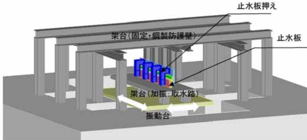
第 1-61 図 試験装置 (参考) ※試験計画の検討により変更の可能性あり
