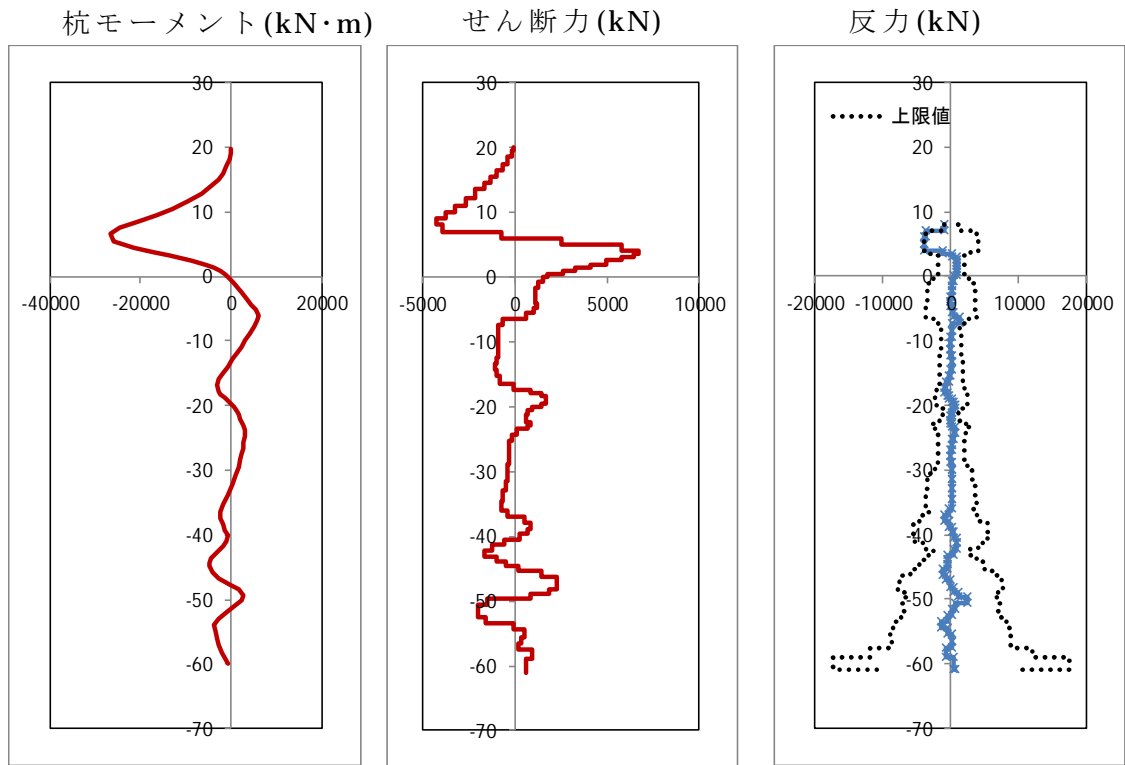
第 3-47 図 曲げモーメント・せん断力及び反力 (基準津波+余震時) (その 1 のバネ)
