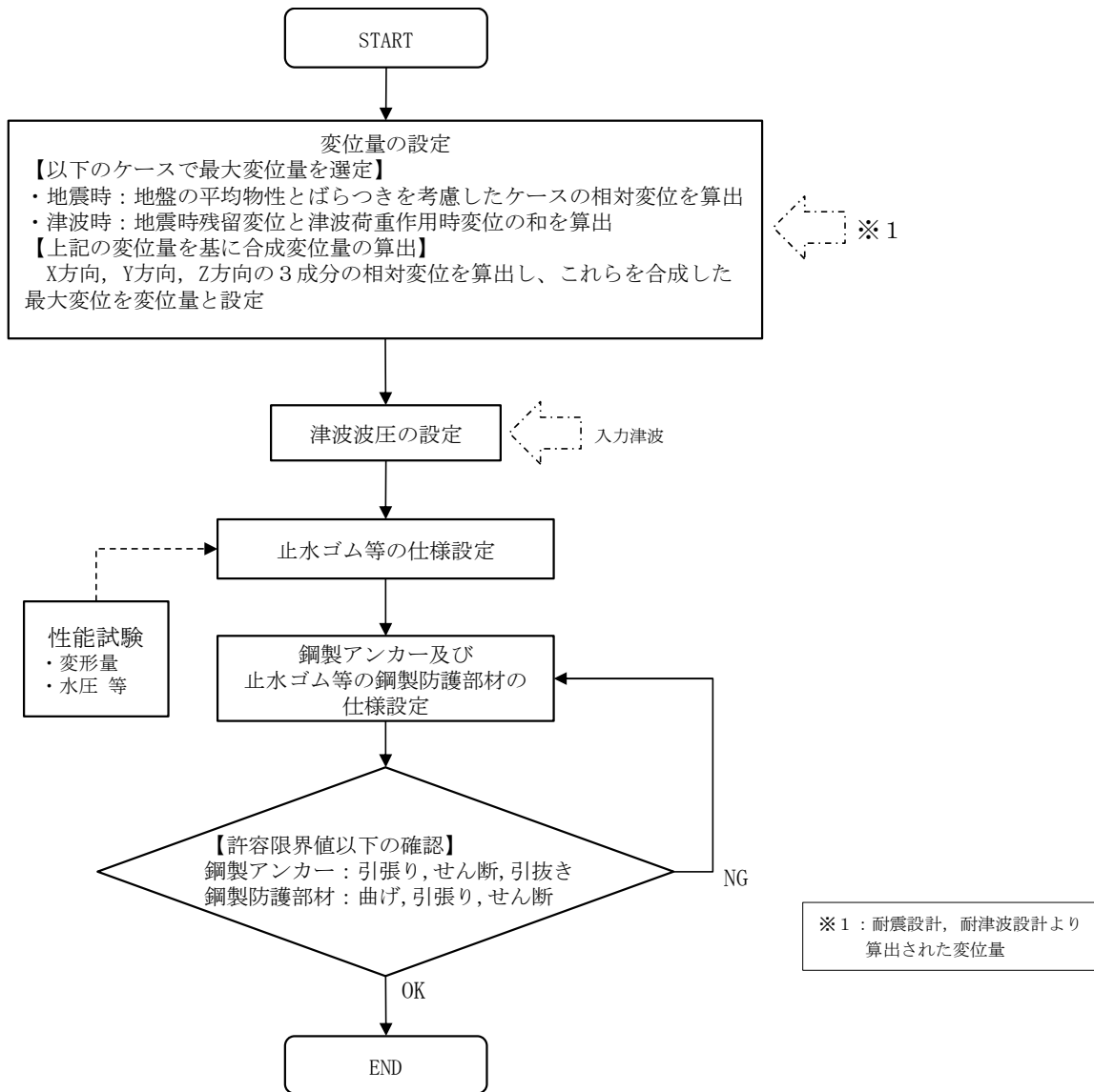
第 1-37 図 止水ジョイント部の設計フロー
