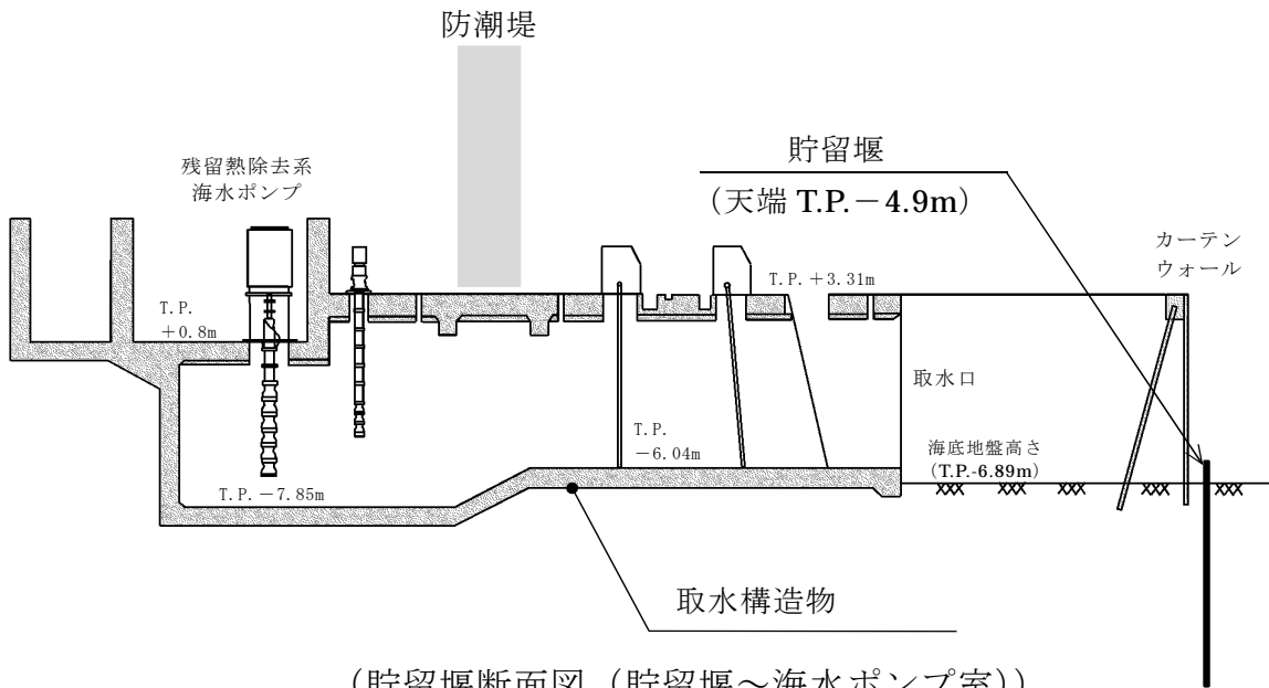
(貯留堰断面図 (貯留堰～海水ポンプ室))
