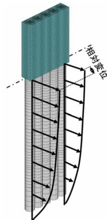
第 1-13 図 三次元 F E M 解析の概念図
