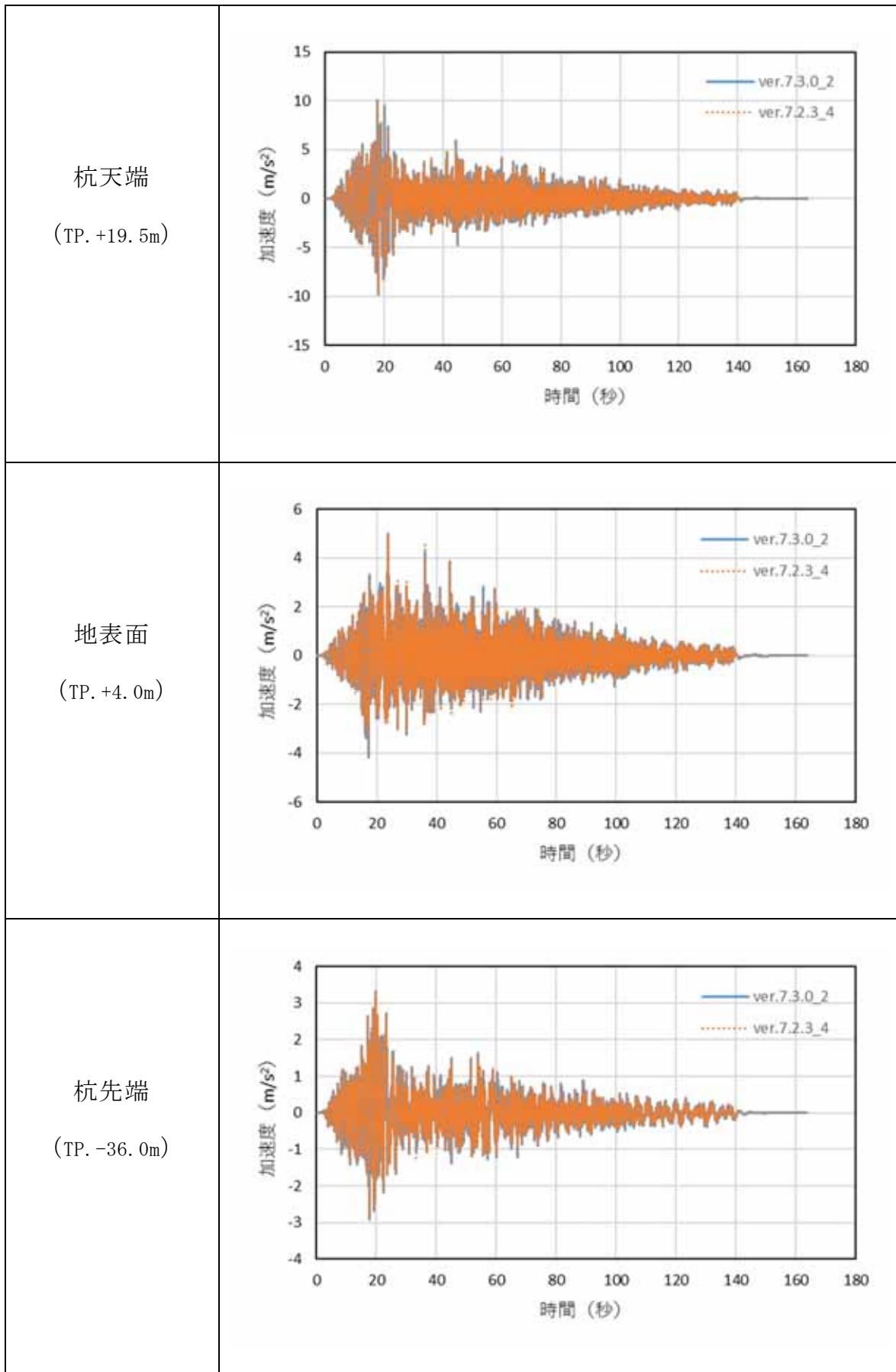
図 4 水平方向加速度 ( m/s^2 ) (杭軸方向非線形バネを考慮した場合)
