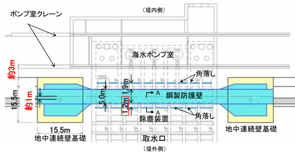
第 1-17 図 取水路周辺の平面図
