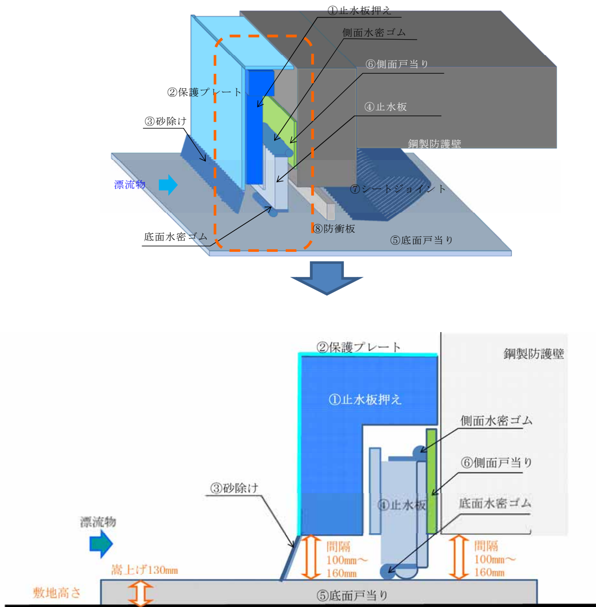
第 1-52 図 止水機構の構成部材の寸法
