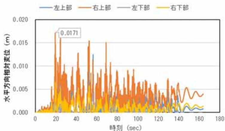
第 3-31 図 (1) ①縦断 (T.P. - 31.36m) 杭長一定ケース 相对変位
