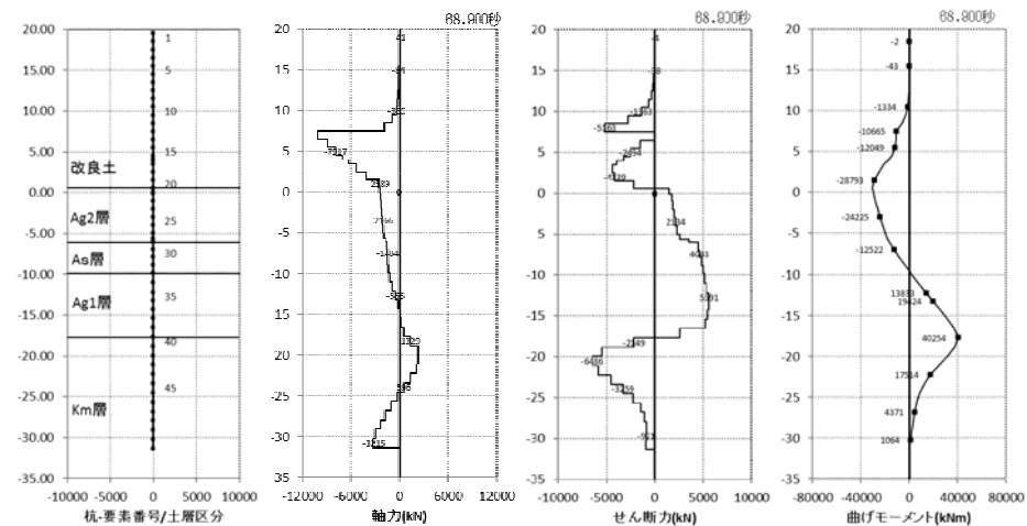
① 縦断（最浅部：杭先端 T.P. - 31.36m）せん断照査時刻時
