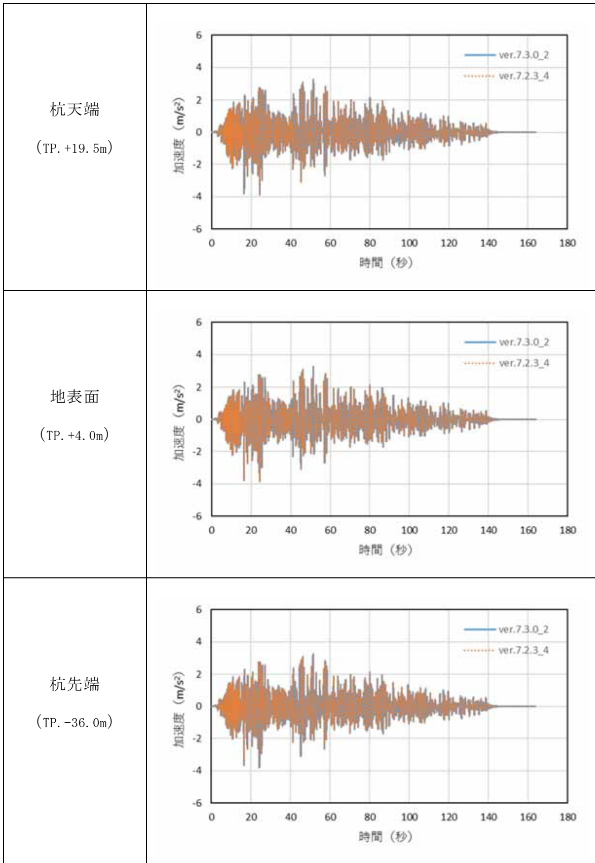
図 3 鉛直方向加速度 ( m/s^2 ) (杭軸方向非線形バネを無視した場合)
