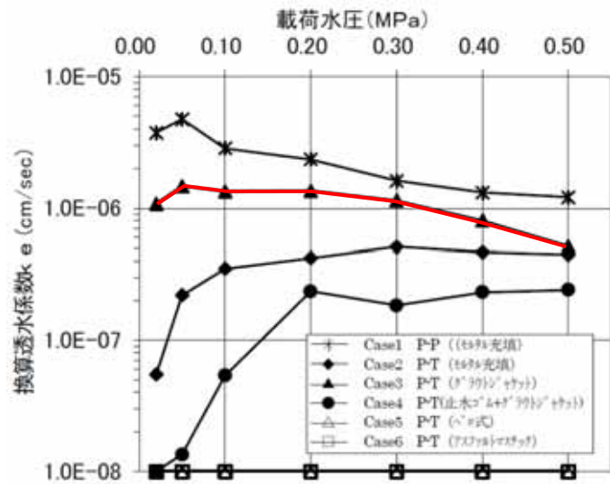
第 2 図 鋼管矢板継手部止水処理形状および遮水性能評価試験結果
