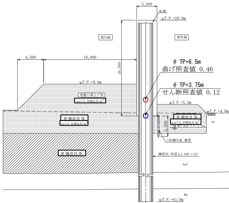
第 3-46 図 曲げ・せん断照査値 (基準津波+余震時) (その 1 のバネ)
