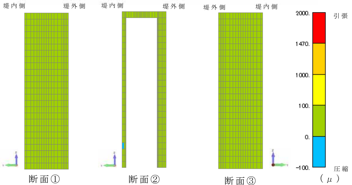
第 3-85 図 地震時（岩盤傾斜モデル）の解析結果 （最大主ひずみ分布）
