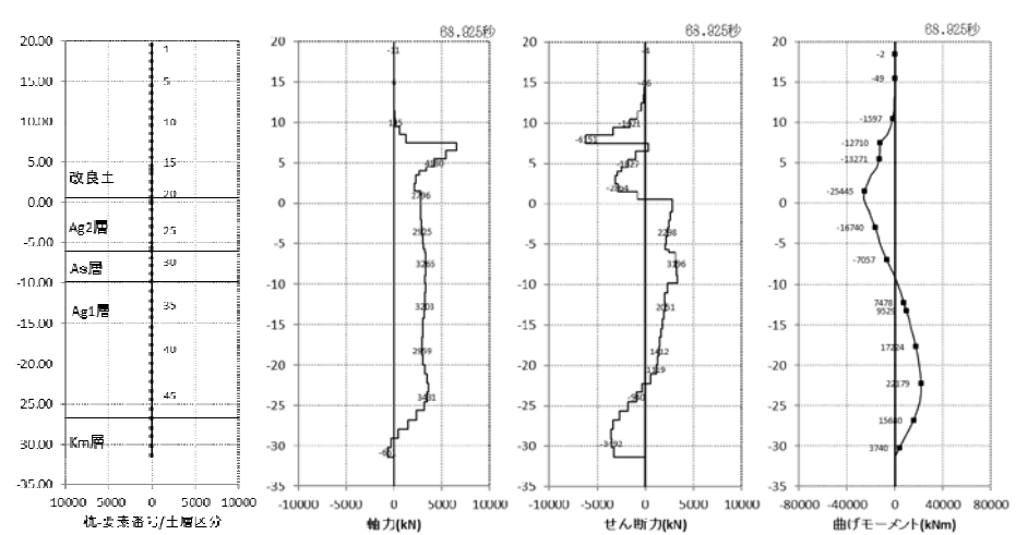
②縦断 1D ケース(最深部:杭先端 T.P.-31.36m)せん断照査時刻時
