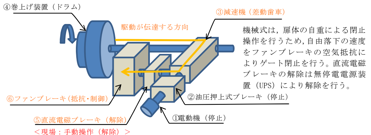
第5図 機械式の構造及び動作原理（閉操作のみ）
