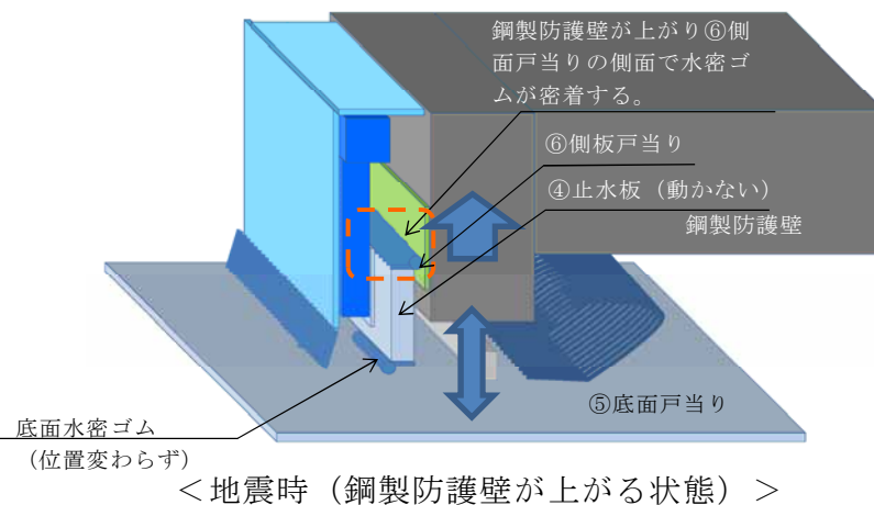
第 1-40 図 1次止水機構の鉛直方向の動作
