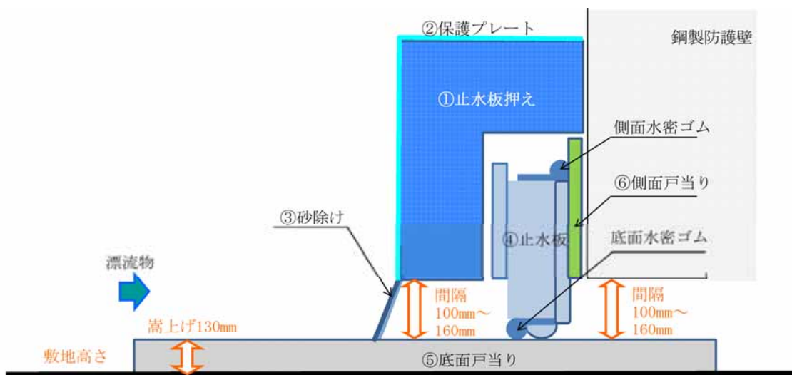
図1-51 鋼製防護壁の概要と各構成部品の概要
