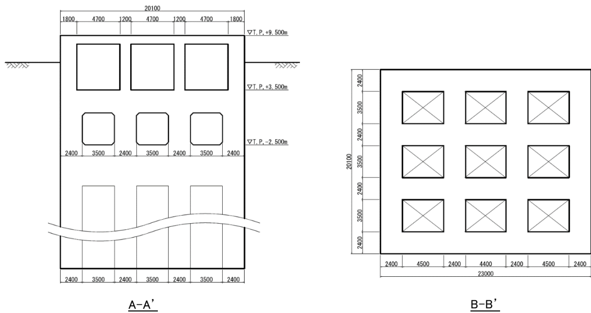
第3図 鉄筋コンクリート防潮壁（放水路エリア）構造図
