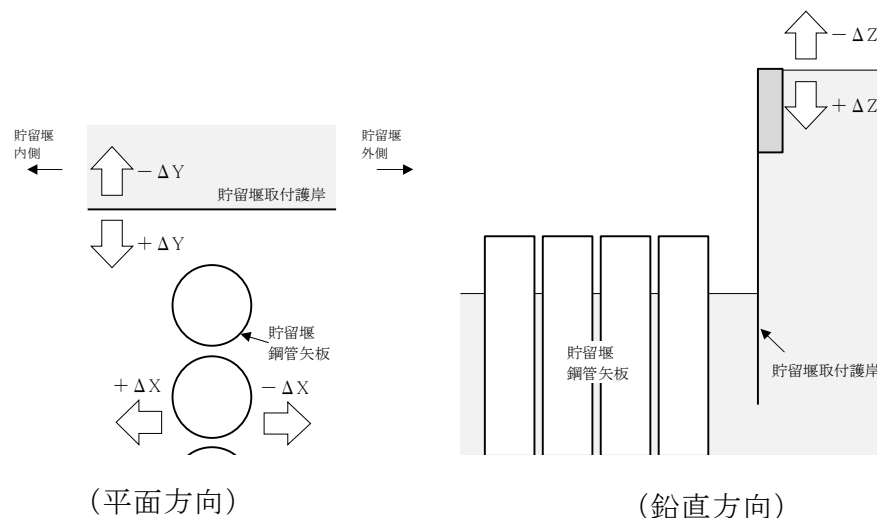
第 2-3 図 貯留堰本体と貯留堰取付護岸との相対変位の考え方
