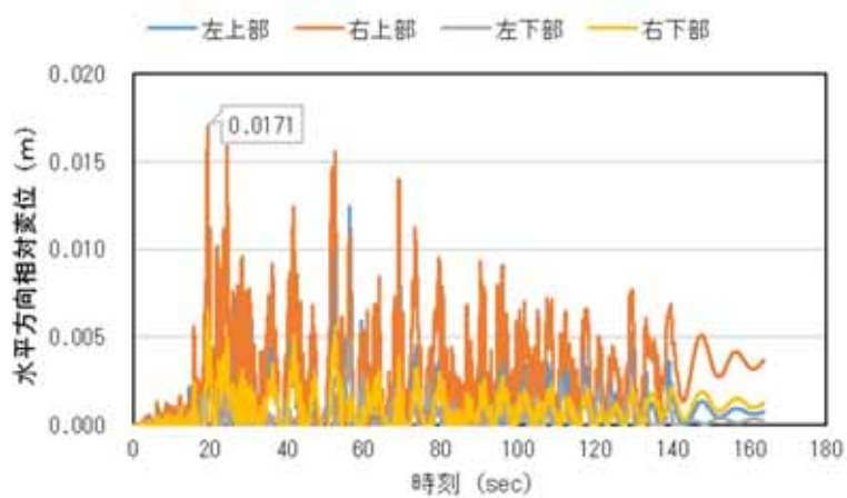
第 3-31 図 (2) ②縦断_1D 根入れケース 相对変位
