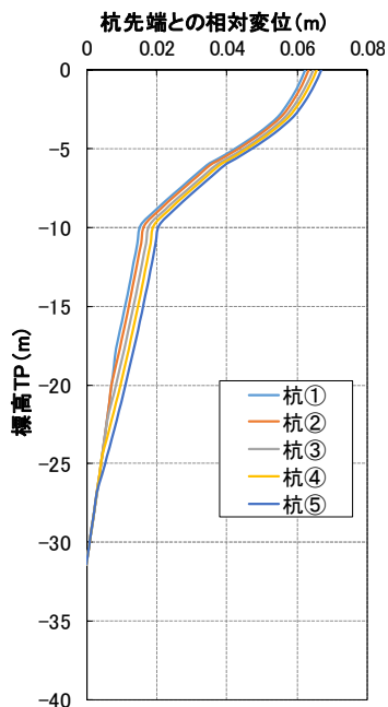
第 3-76 図 地中変位分布及び地表面最大加速度 (地震時・一般部, 地点③)
