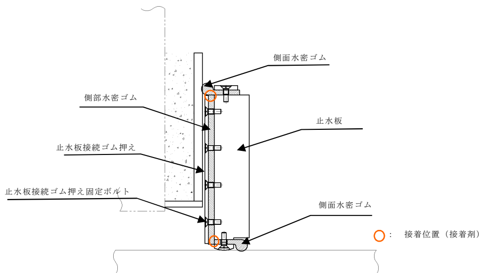
第1-64図 止水板接続ゴムと止水板の固定概要図 (A-A 矢視)
