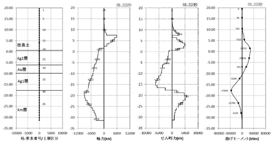
① 縦断（最浅部：杭先端 T.P. - 31.36m）曲げ軸力照査時刻
