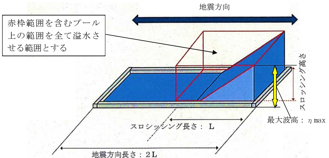
第 9.11-2 図 スロッシング時の溢水量の設定（矩形）
