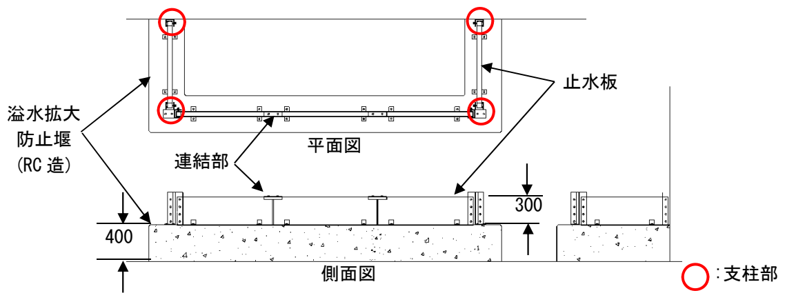
第 9.11-6 図 溢水拡大防止堰への止水板設置概要図
