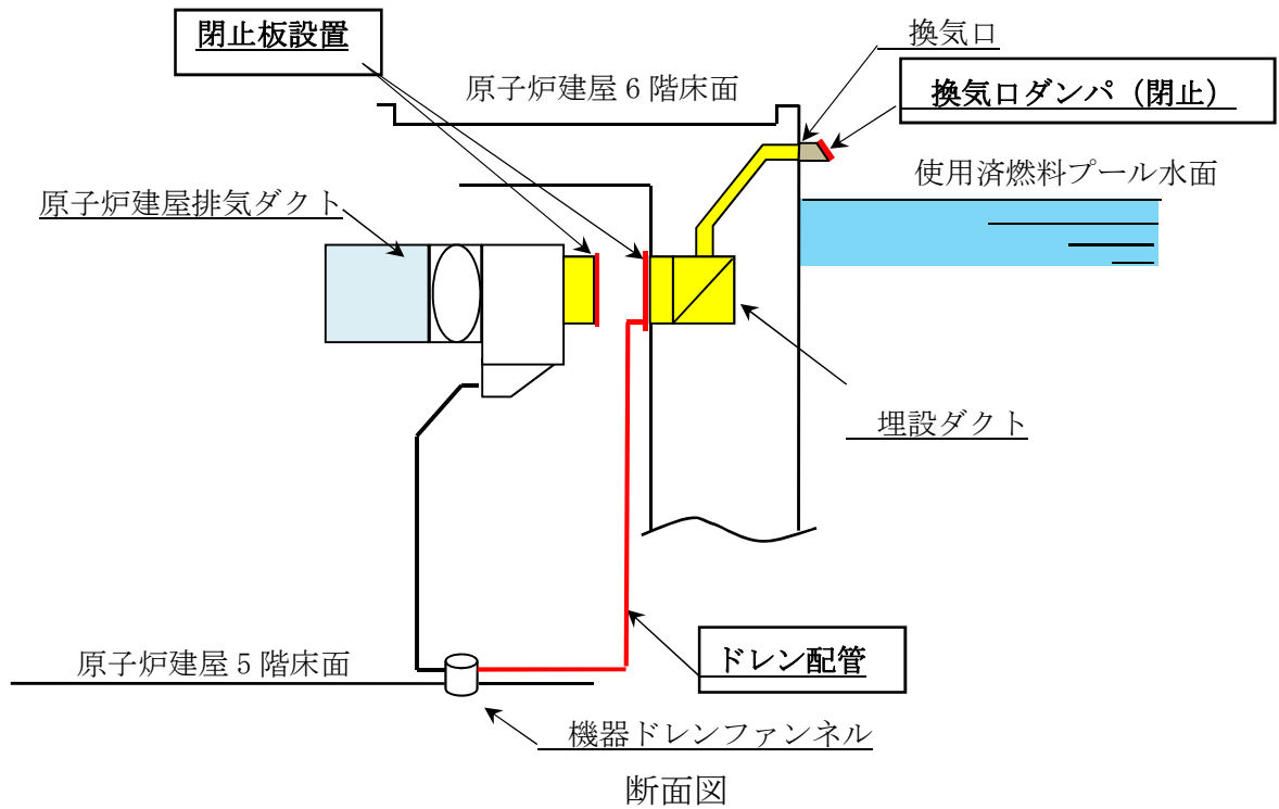
第 9.8-5 図 閉止板設置箇所
