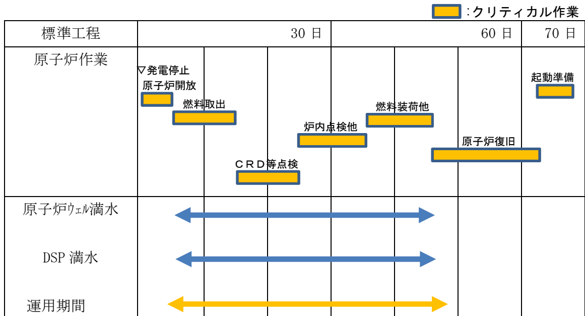
第9.11-10図 施設定期検査工程例
