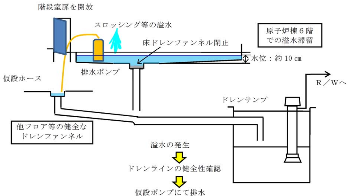
第9.11-9 図 停止時の床ドレンファンネル閉止・堰の排水切欠き閉塞時における排水処理について
