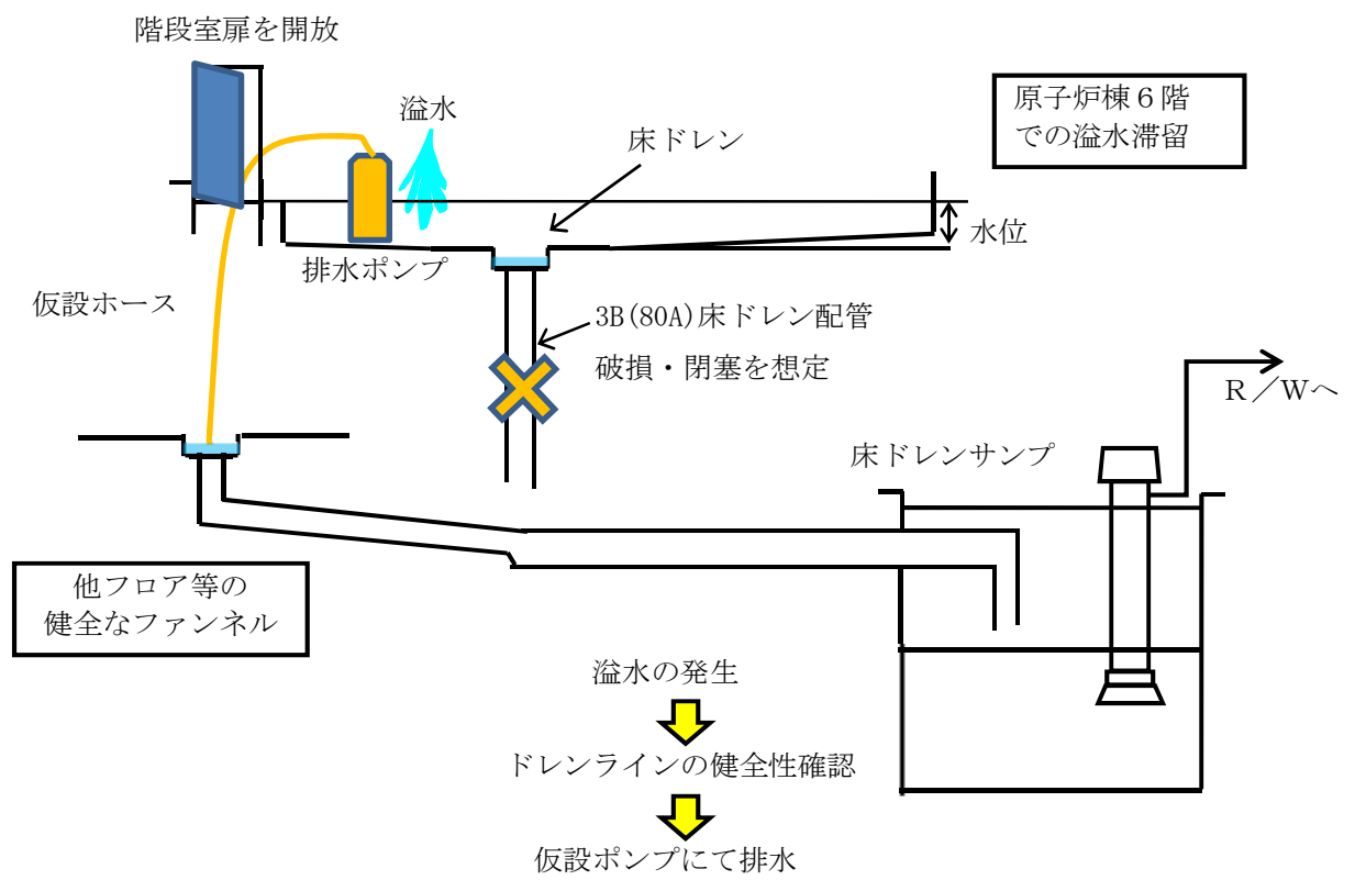
第9.18-2 図 地震時の床ドレンファンネル破損・閉塞時における排水処理について
