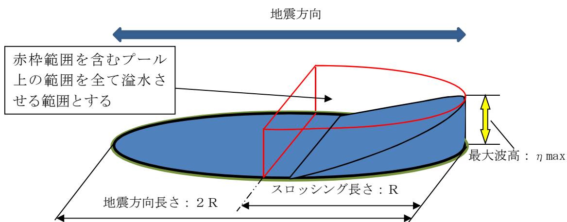
第 9.11-3 図 スロッシング時の溢水量の設定 (円筒形)
