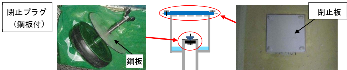
第 9.11-5 図 床ドレンファンネルの閉止例
