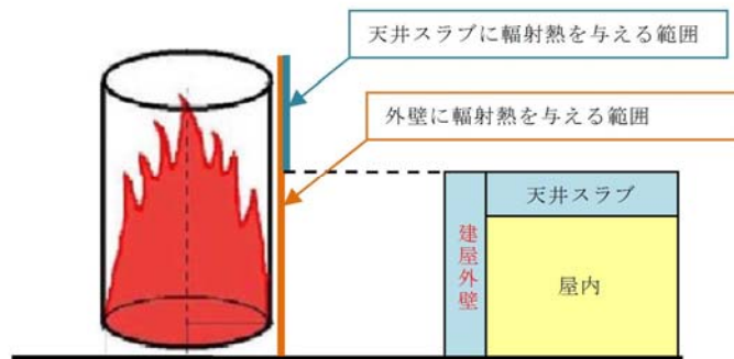
図 2.1.1-3 天井スラブの評価概念図
