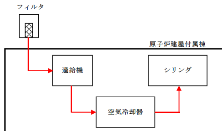
第 3.1-1 図 非常用ディーゼル発電機（高圧炉心スプレイ系ディーゼル発電機を含む。）吸気系統概略図
