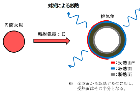
第5.4-2図 排気筒の評価概念図
