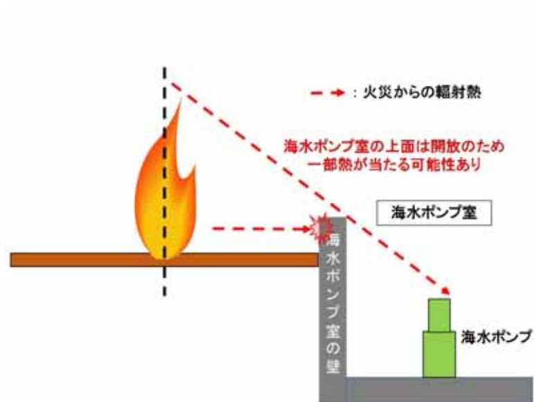
第 2. 2. 4-1 図 火災発生位置と海水ポンプの位置関係
