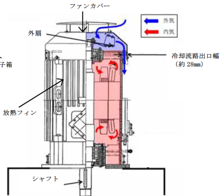
第2.4.2-7図 非常用ディーゼル発電機（高圧炉心スプレイ系ディーゼル発電機を含む。）用海水ポンプ電動機 構造図
