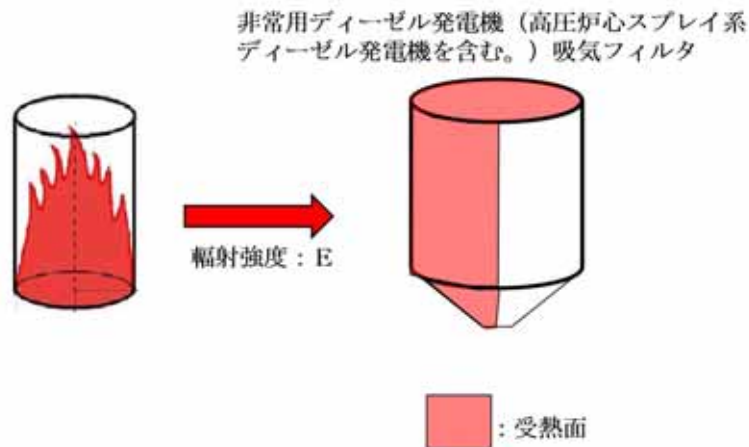
第 4.3.2.4-2 図 非常用ディーゼル発電機（高圧炉心スプレー系ディーゼル発電機を含む。）吸気フィルタの評価概念図
