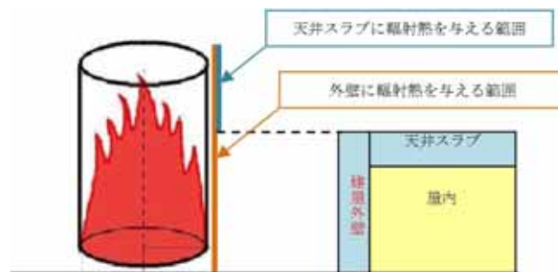
第 4.3.2.1-3 図 天井スラブへの放射熱の影響概念図
