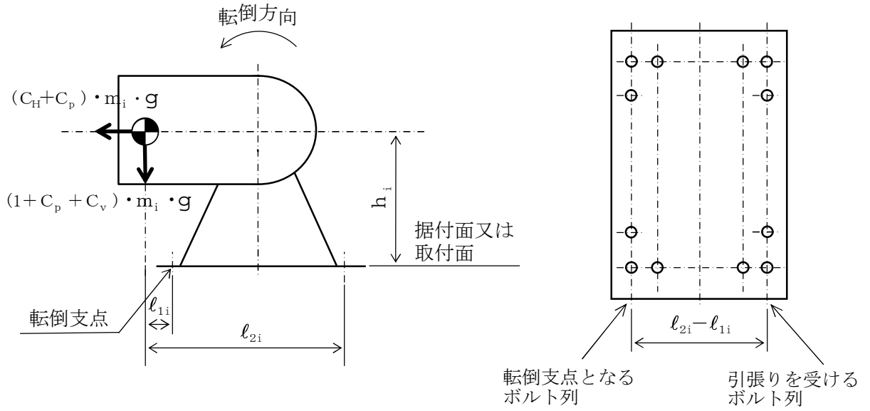
図 4-2 (3) 計算モデル
