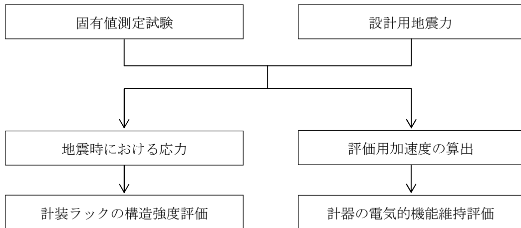
図 2-1 直立形計装ラックの耐震評価フロー
