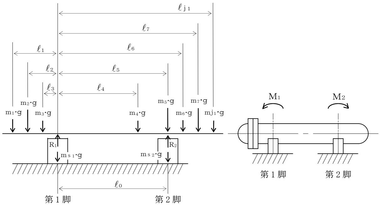
図4-1 荷重状態
