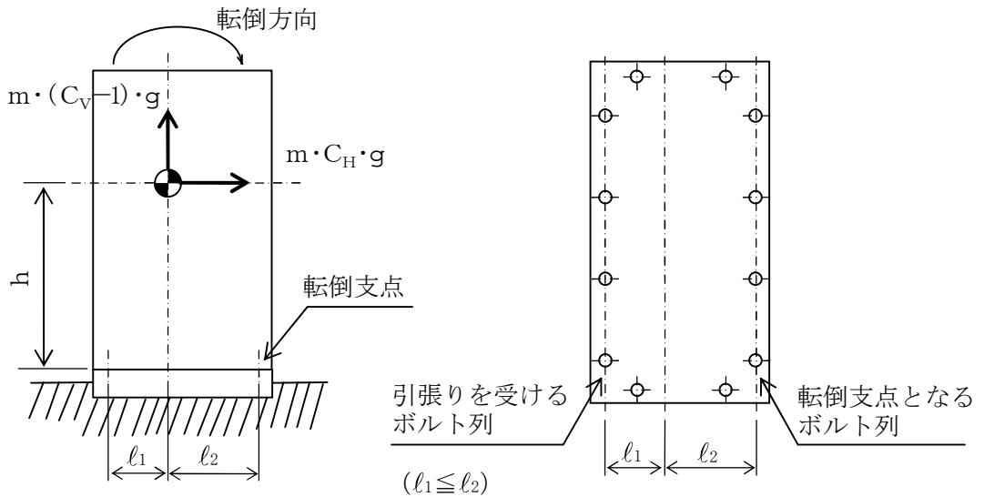
図5-2(2) 計算モデル
