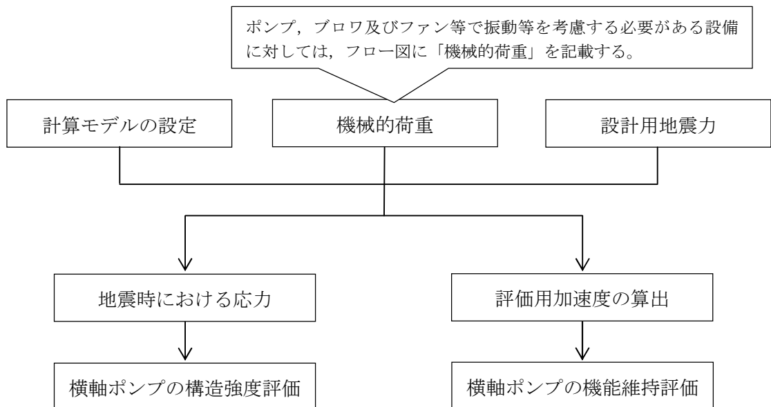
図2-1 横軸ポンプの耐震評価フロー
