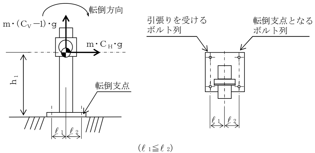
図5-3(2) 計算モデル
