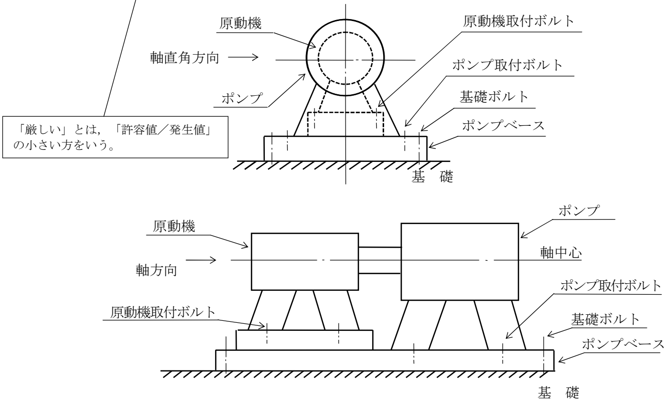
図 4-1 概要図
