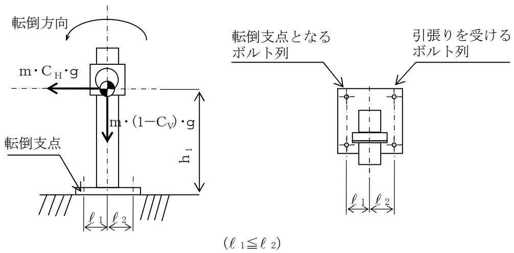
図5-3(1) 計算モデル
