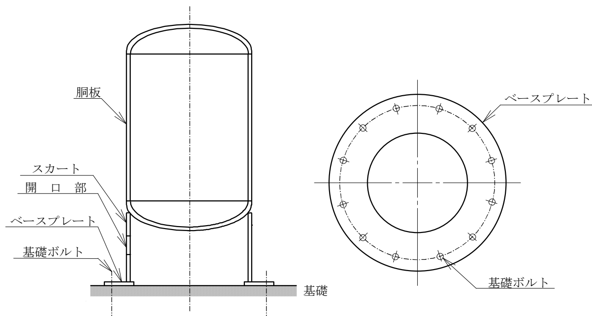
図5-1 概要図
