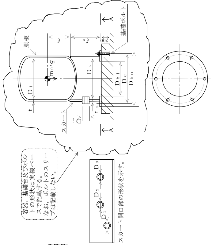
A~A矢視図
