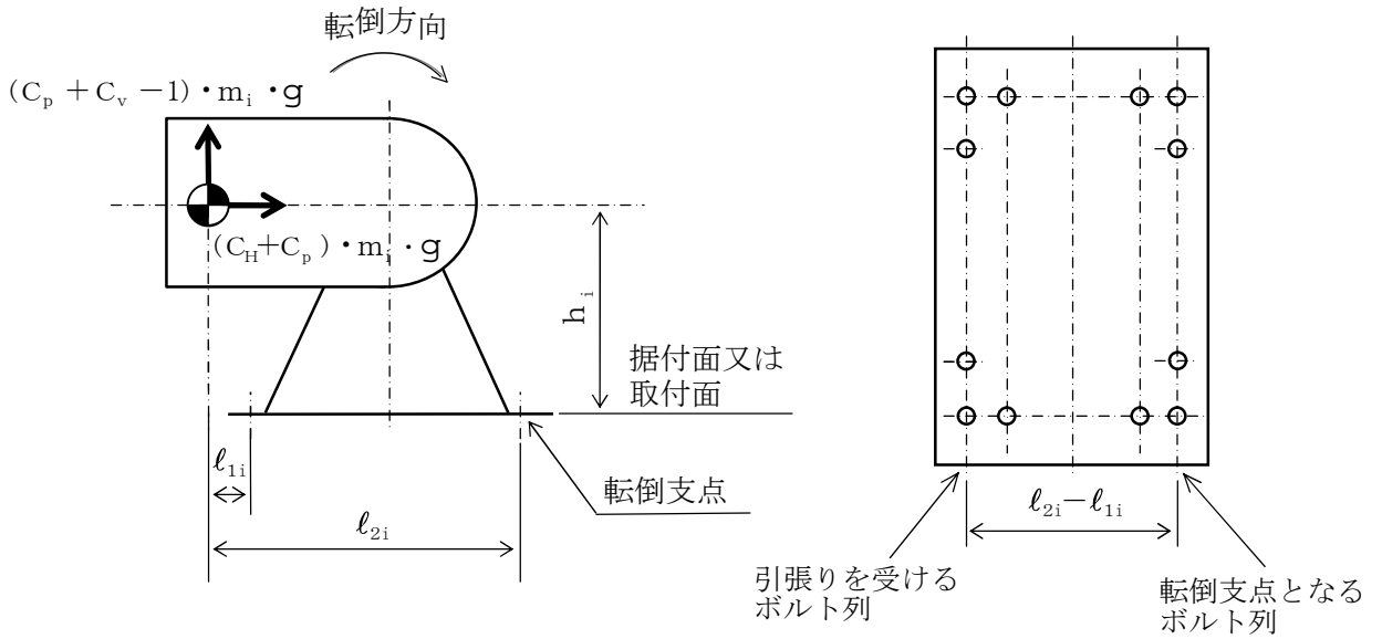
図 4-2 (4) 計算モデル
