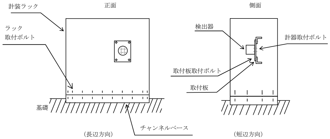
図 5-1 概要図 (直立形)
