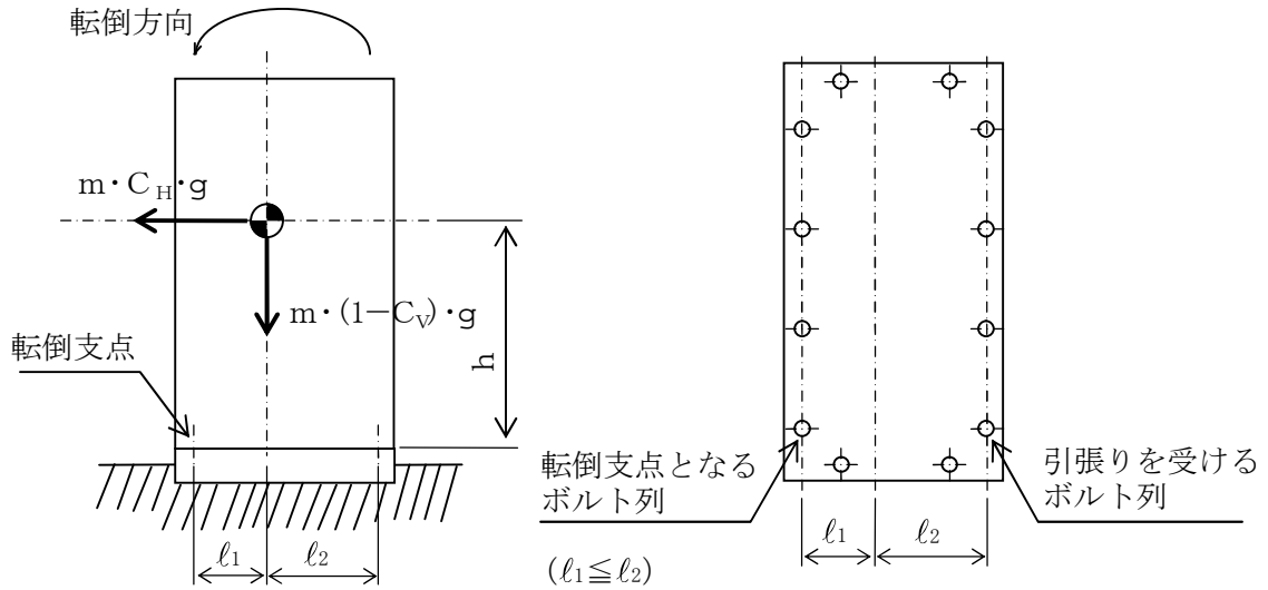
図5-2(1) 計算モデル
