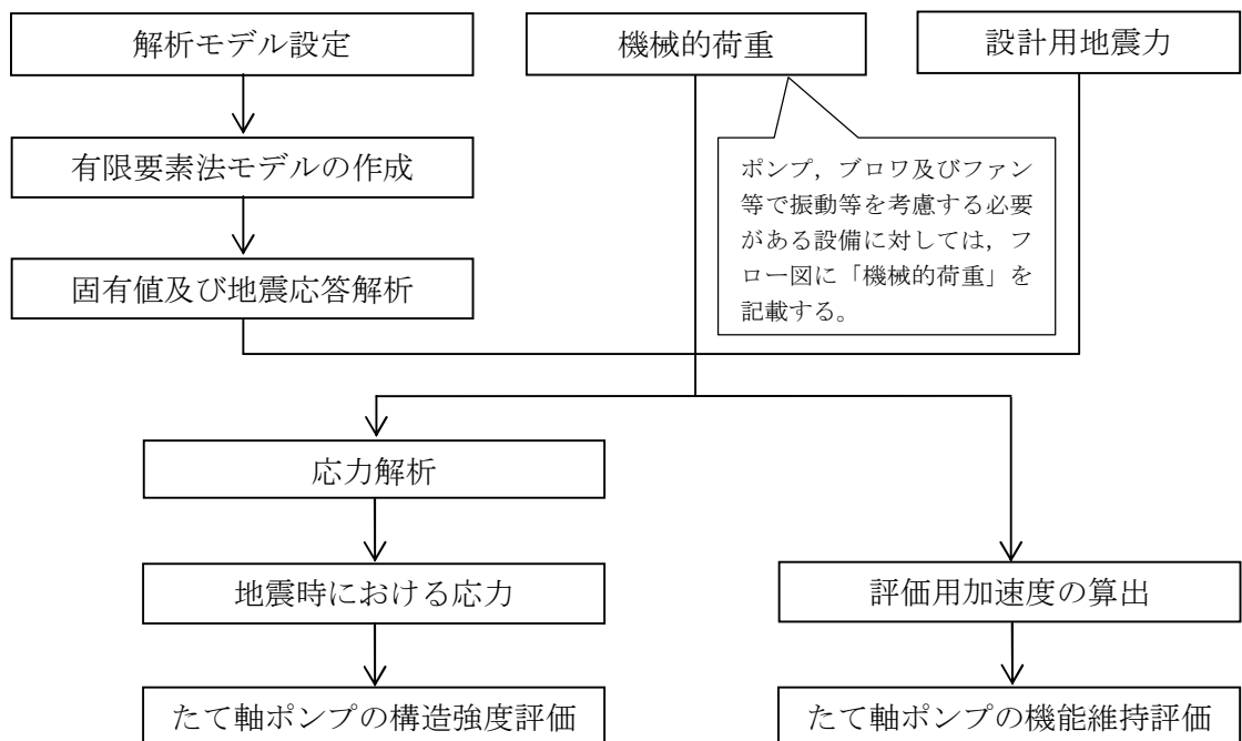
図 2-1 たて軸ポンプの耐震評価フロー
