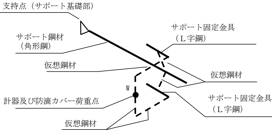
図4-1 解析モデル
