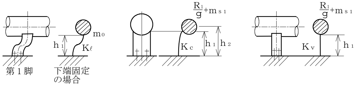
図4-5 長手方向の固有周期 計算モデル 図4-6 横方向の固有周期 計算モデル 図4-7 鉛直方向の固有周期 計算モデル
