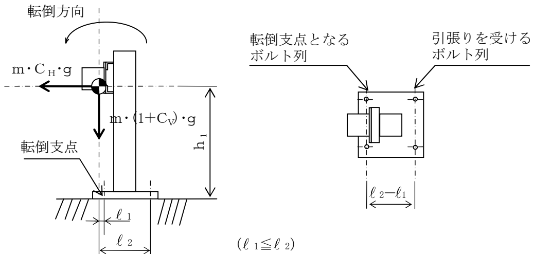
図5-4(3) 計算モデル
