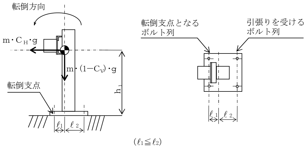
図5-4(1) 計算モデル
