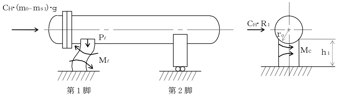
図4-3 長手方向荷重による胴の第1脚付け根部のモーメント及び鉛直荷重
