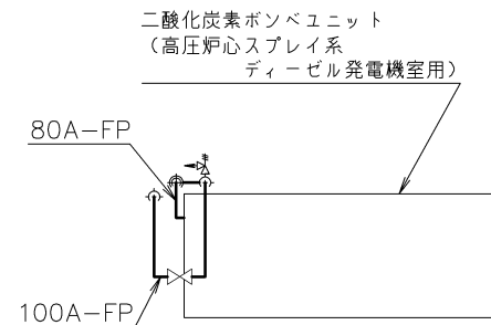
A~A矢视图
