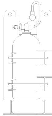
A~A矢视图
