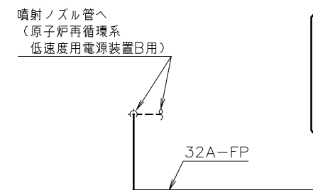
B~B矢視図
