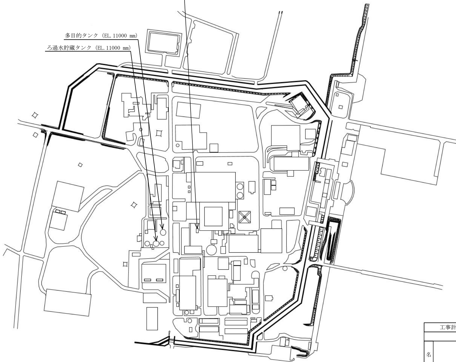
構内敷地図
