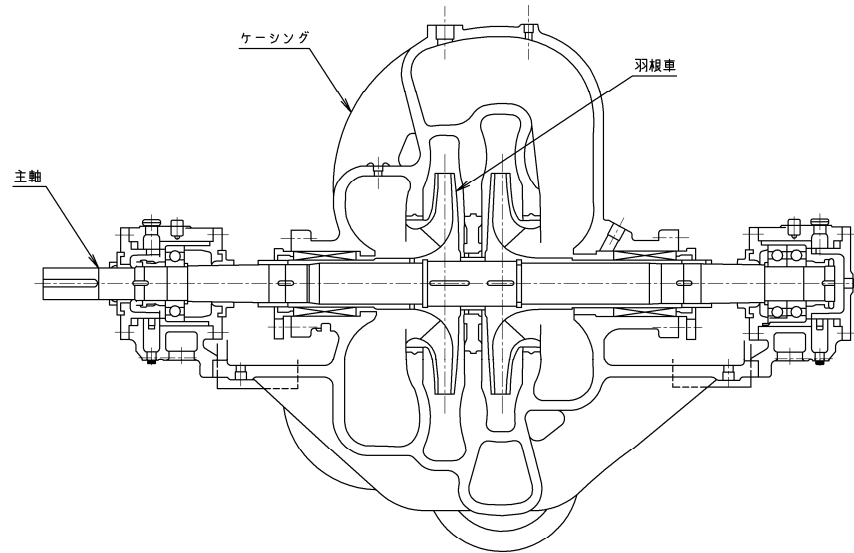
B~B断面図
