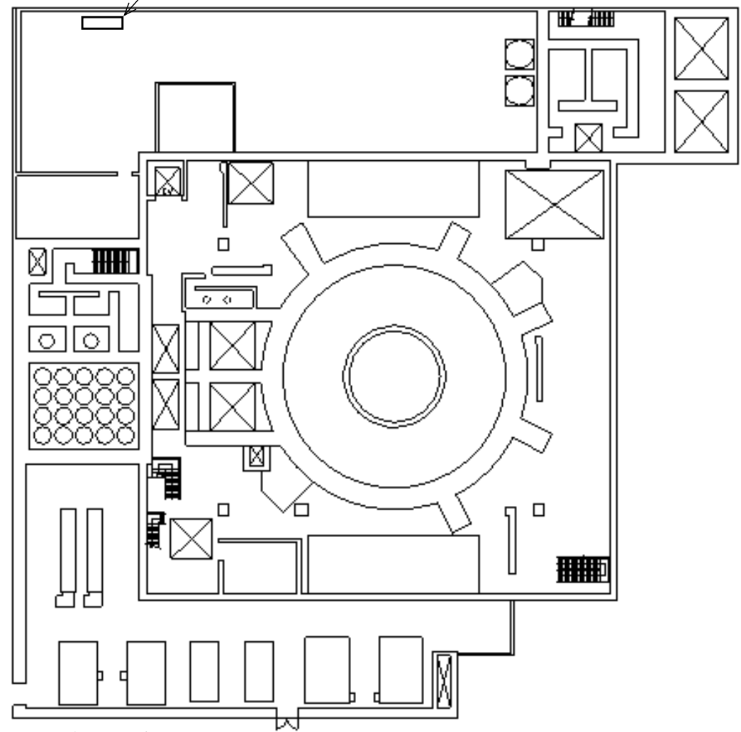
原子炉建屋原子炉棟 EL. 23000 mm
