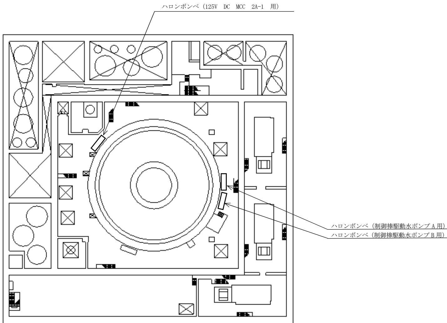
原子炉建屋原子炉棟 EL.2000 mm
