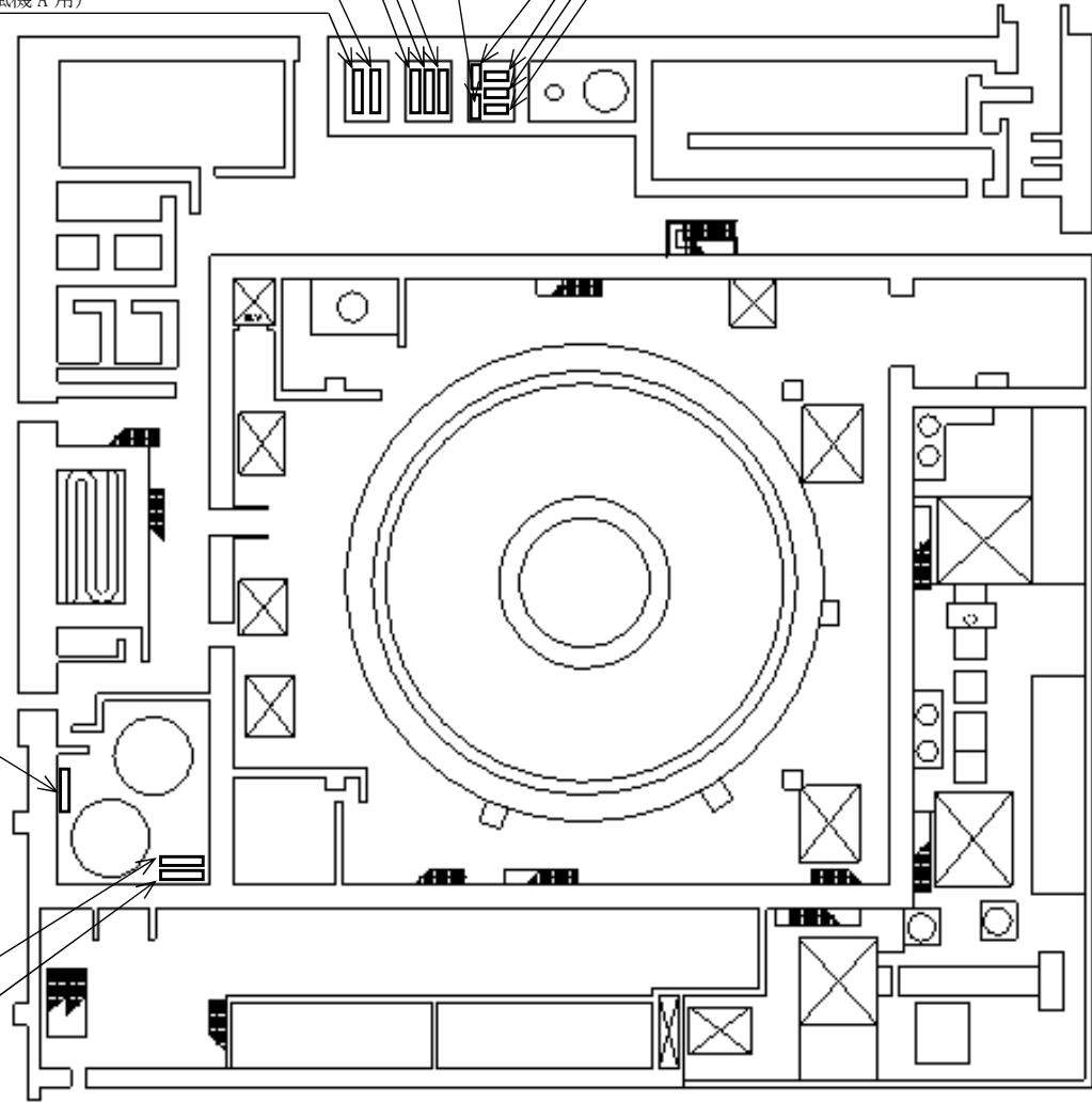
原子炉建屋付属棟 EL. 8200 mm
