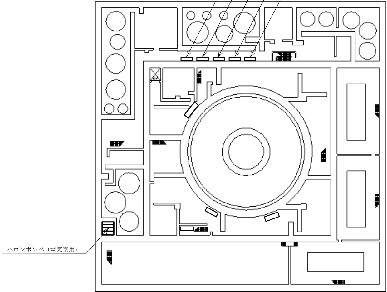
原子炉建屋付属棟 EL. -4000 mm
