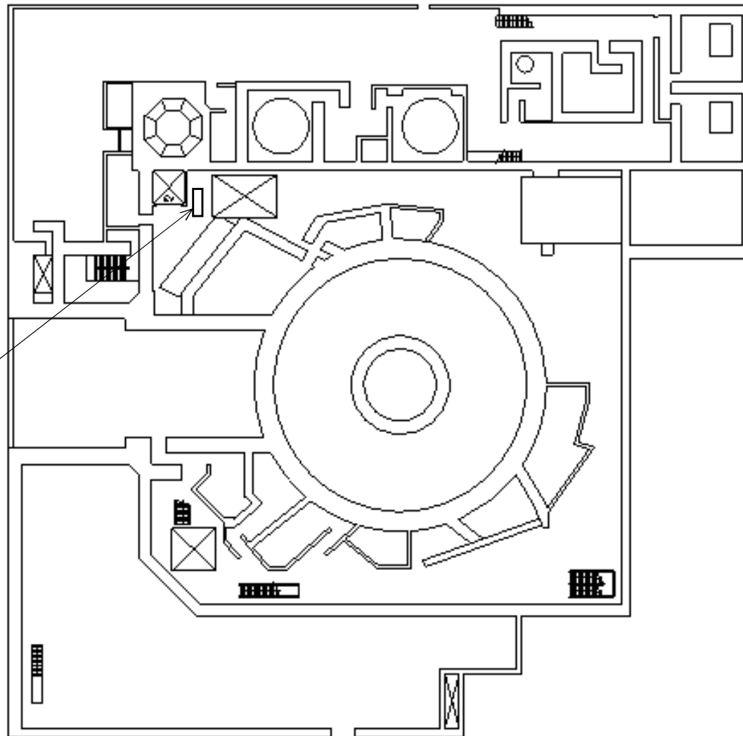
原子炉建屋原子炉棟 EL. 14000 mm
