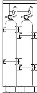
A~A 矢視図
