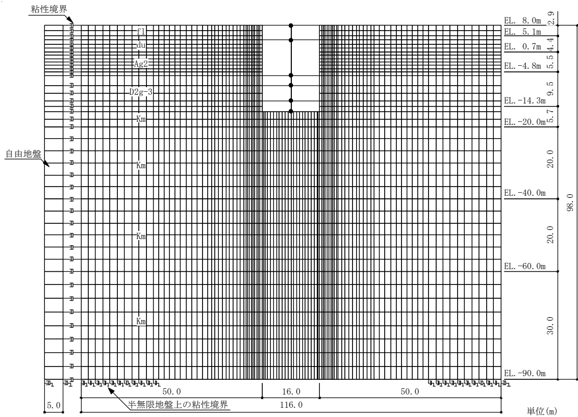
図3-4 地震応答解析モデル (UD方向全体)
