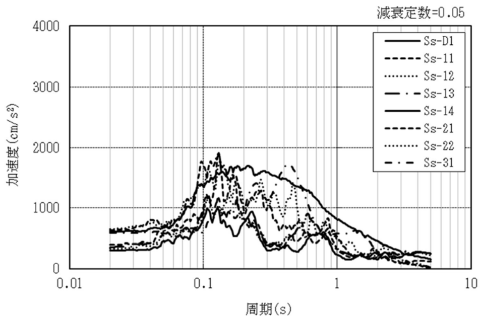
図3-7 (1/2) 入力地震動の加速度応答スペクトル ( S_s , EL. -90.0 m)
