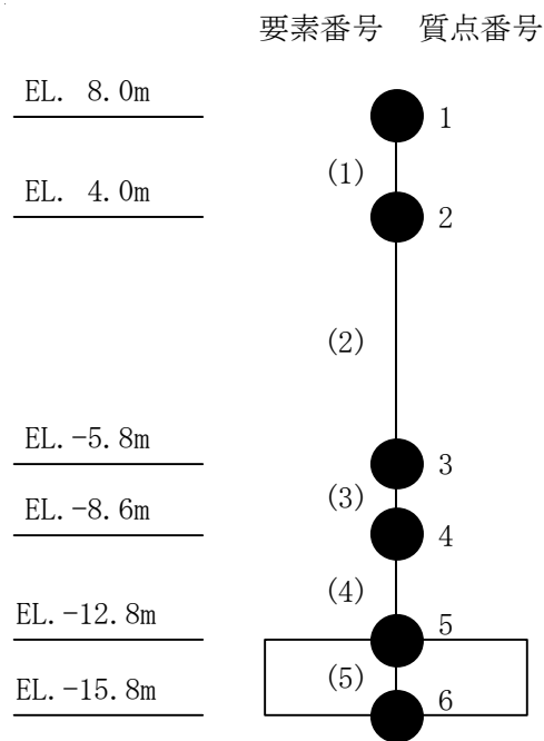
図3-5 地震応答解析モデル (UD方向構造物)
