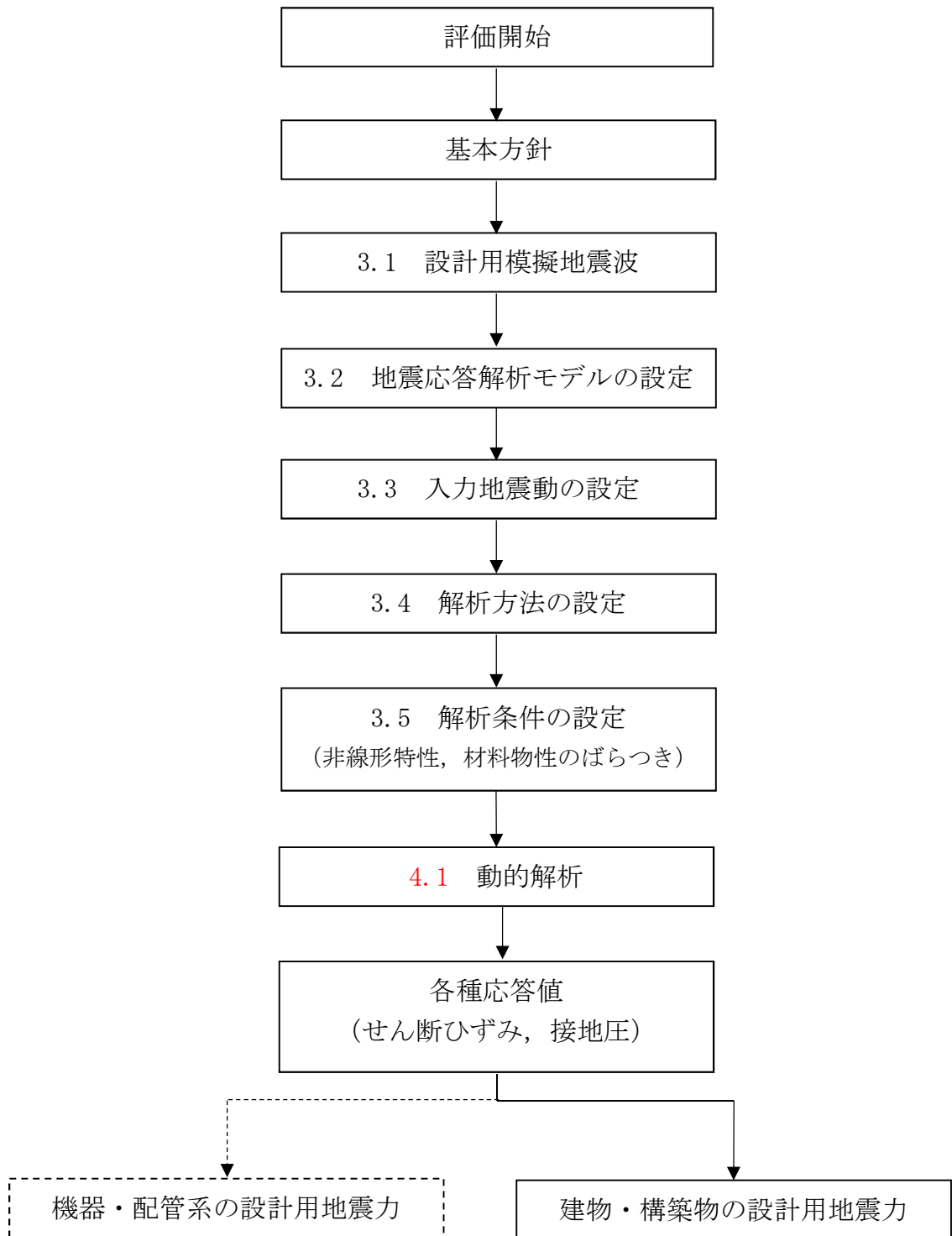
図2-4 格納容器圧力逃がし装置格納槽の地震応答解析フロー
