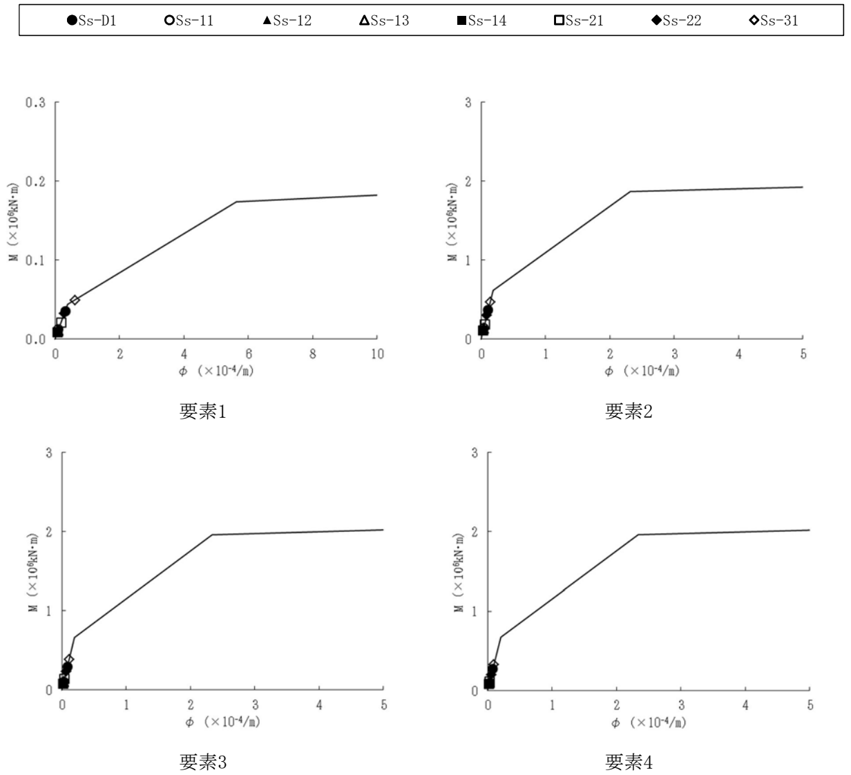
図4-15 曲げスケルトンカーブ上の最大応答値 ( S_s , EW方向)
