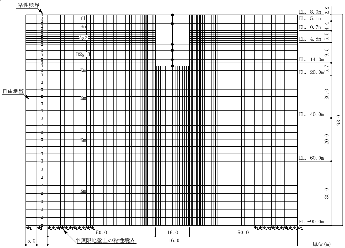
図3-1 地震応答解析モデル (NS方向全体)
