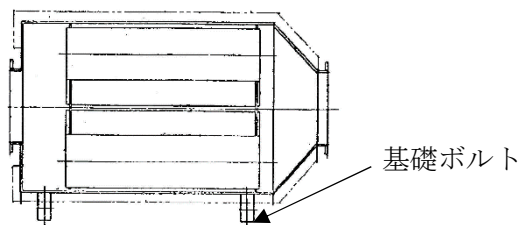
図3-3 ディーゼル発電機排気消音器（非常用ディーゼル発電機 2 D, 高圧炉心スプレイ系ディーゼル発電機）の評価対象部位（吸収部）
