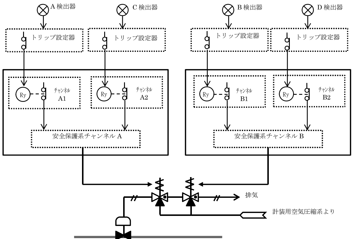
図 3-3-1 原子炉緊急停止系の構成例
