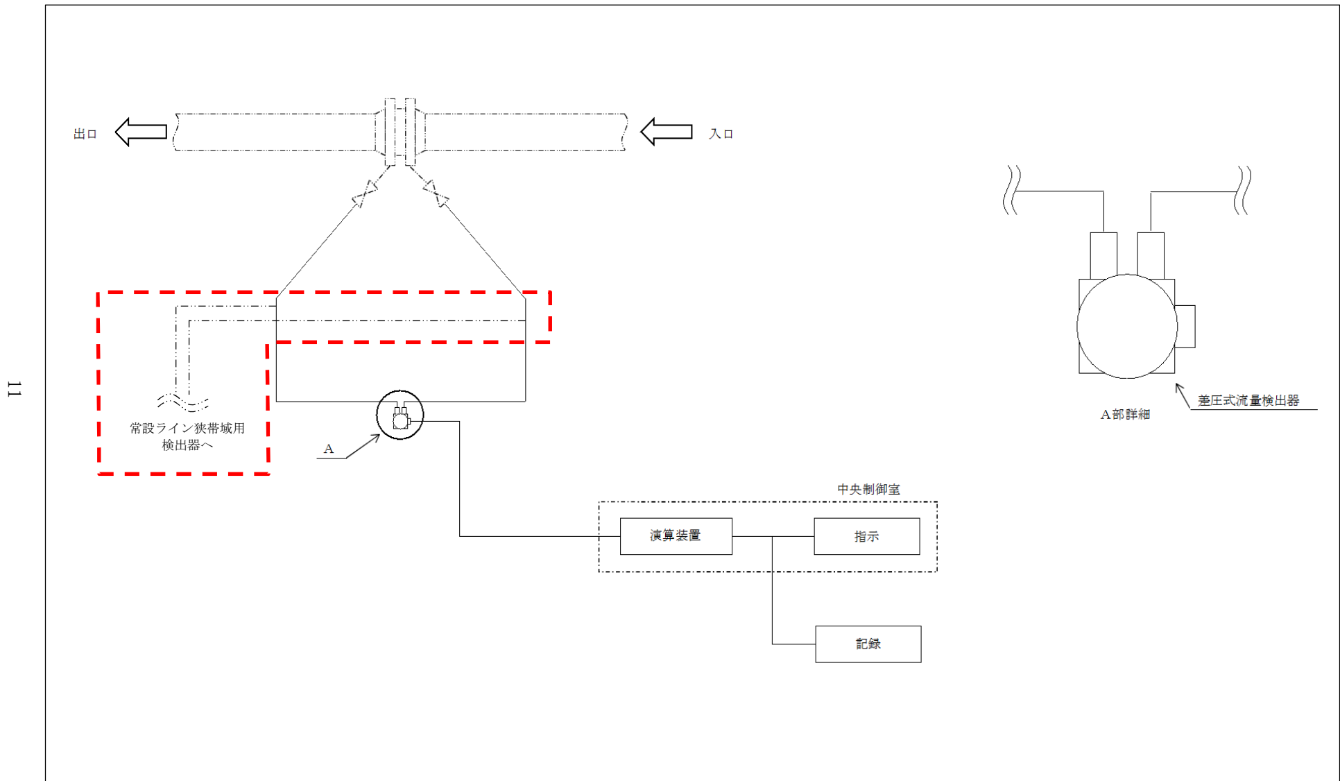
図 3-1-2-6 検出器の構造図 (低圧代替注水系原子炉注水流量 (常設ライン用))
