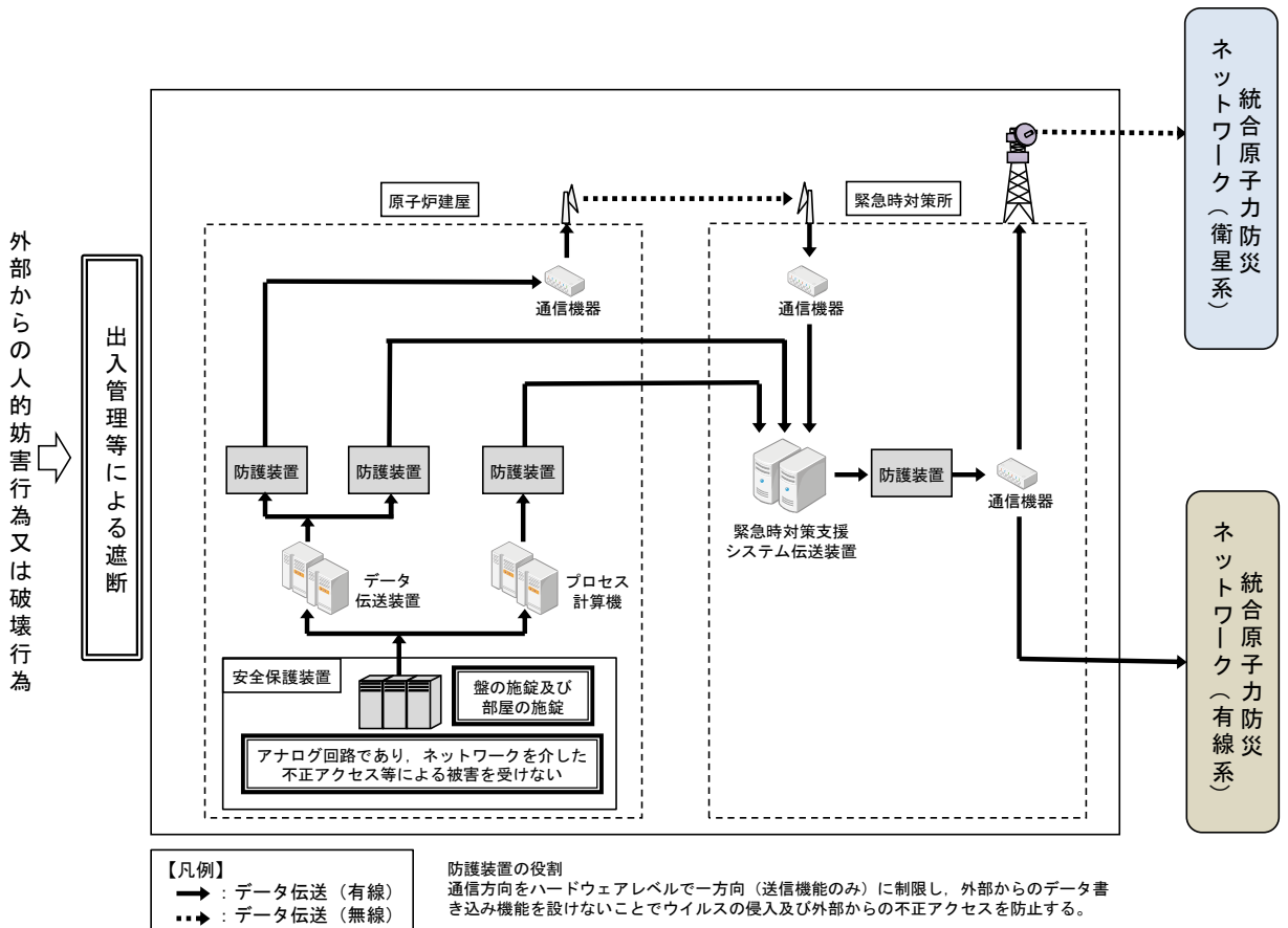
図 3-3-1-1 外部ネットワークと物理的又は機能的な分離概略図
