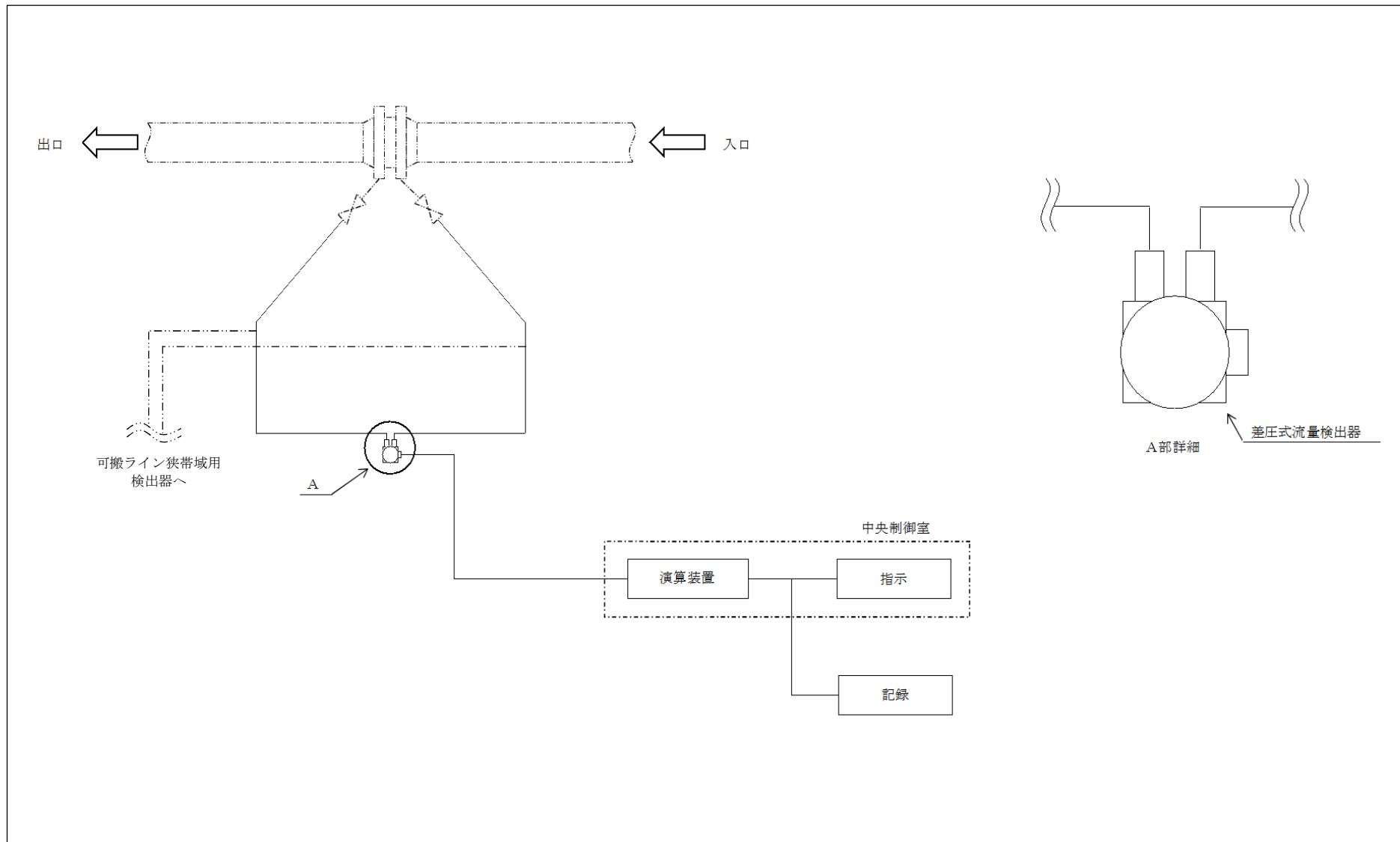
図 3-1-2-10 検出器の構造図（低圧代替注水系原子炉注水流量（可搬ライン用））
