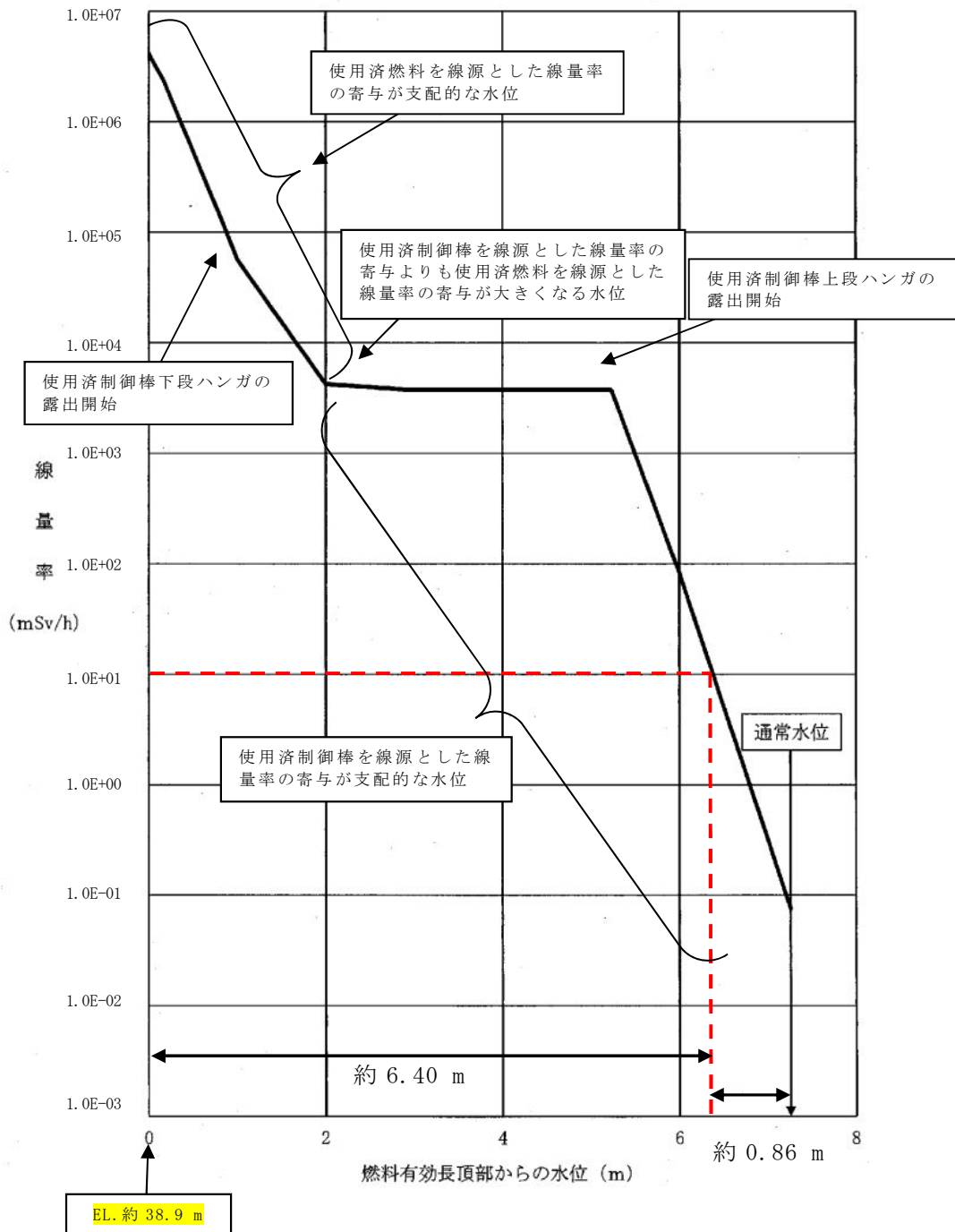
第4図 使用済燃料プールの線量率と水位の関係
