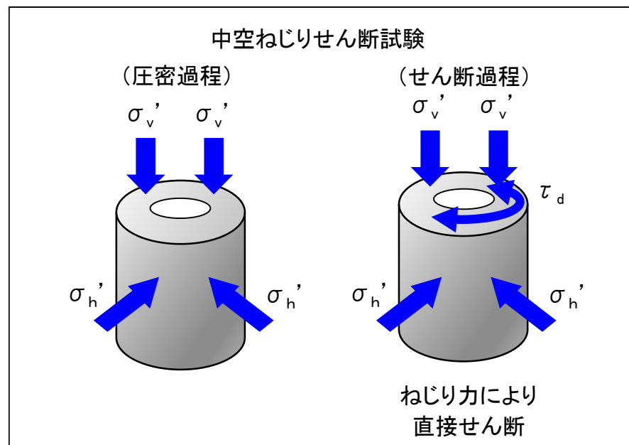
図 4.2-4 中空繰返しねじりせん断試験の概要
