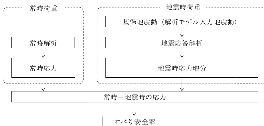
第13-1図 安定性評価フロー
