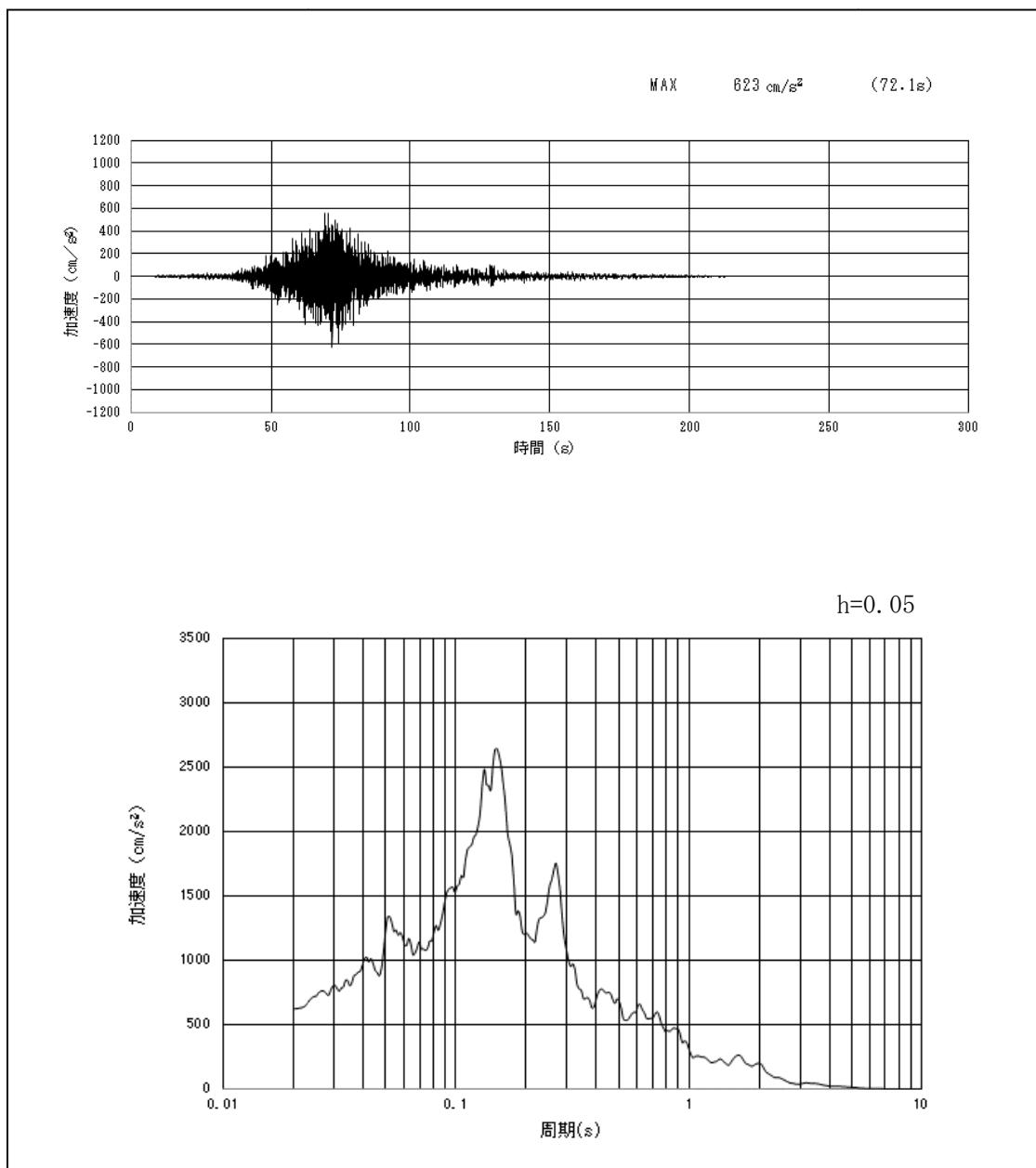
第2-7図 (25) 西側保管場所の入力地震動の加速度時刻歴波形及び加速度応答スペクトル (鉛直方向 東西 : S s -22)
