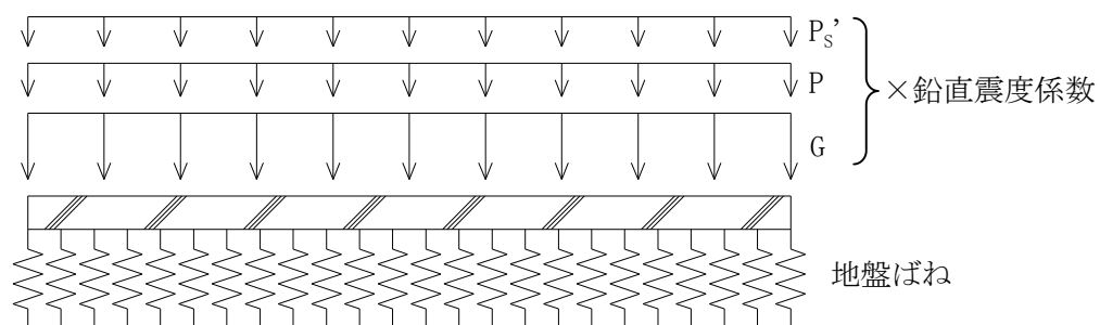
第3-2図 荷重条件
