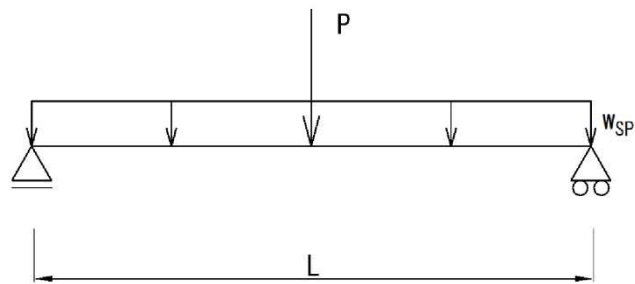
第 9-11 図 荷重図
