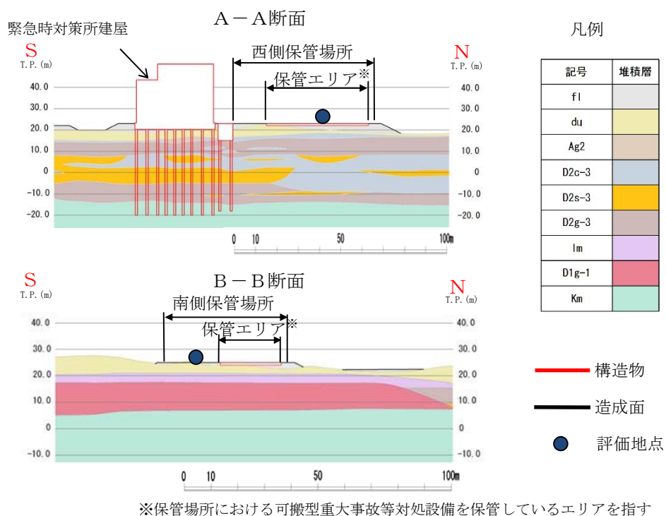
第2-5図 保管場所における液状化及び揺すり込み沈下による不等沈下に対する影響評価断面の位置図及び断面図
