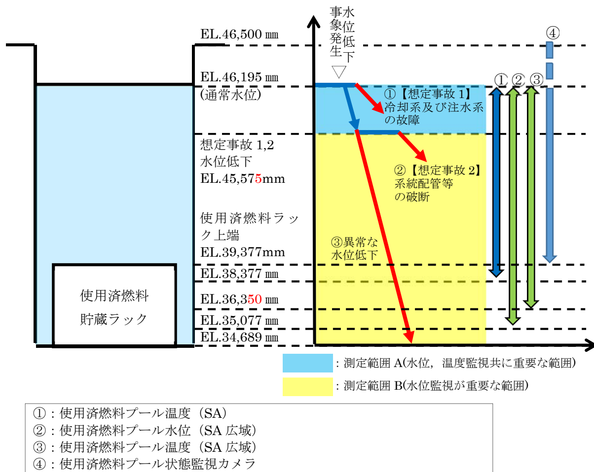
図 3-1 使用済燃料プールの水位が異常に低下した場合の監視設備概略図
