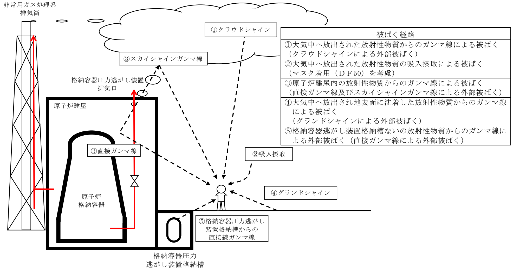
第1図 ベント操作に係る作業時及び水源補給・燃料補給作業の被ばく評価経路イメージ (屋外作業及び移動時)
