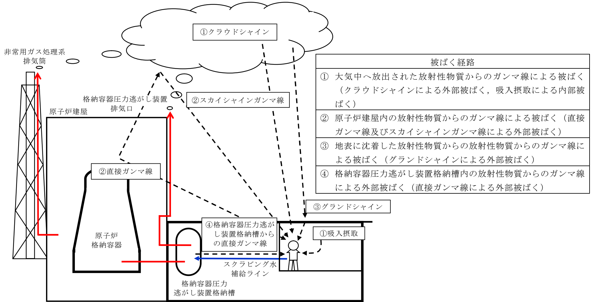
第1図 スクラビング水補給作業時の作業員の被ばく評価経路イメージ
