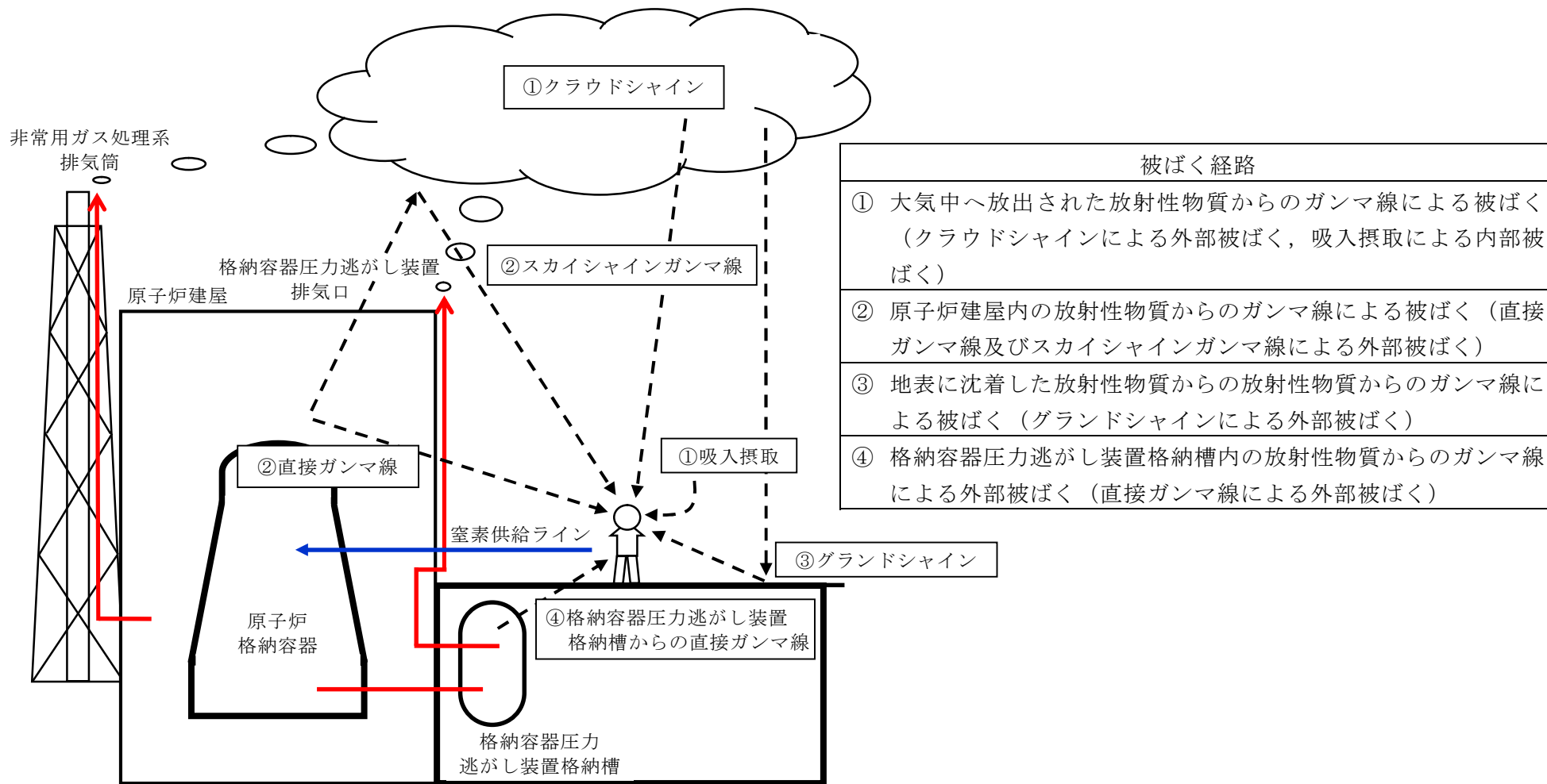
第2図 窒素供給作業時の作業員の被ばく評価経路イメージ
