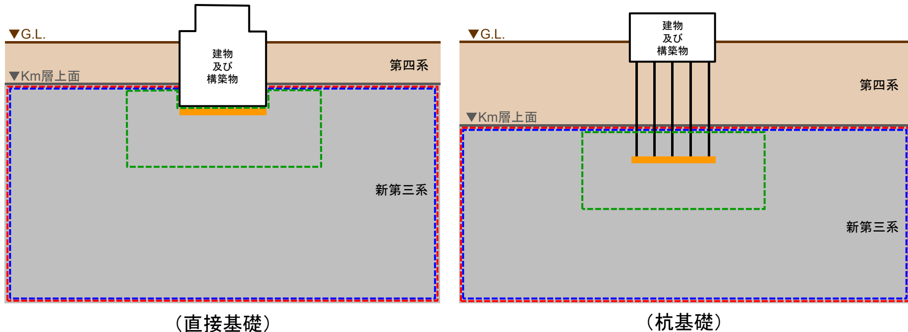
基礎地盤等のイメージ(東海第二の場合)
