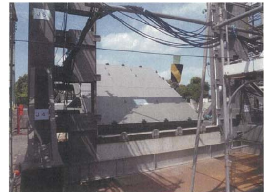
実機大ブローアウトパネル開放試験のイメージ (2012年 自主的安全性向上の一環として、原子炉建屋6階北側強制開放装置設置時の試験例)
