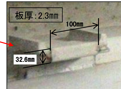
クリップ部拡大 (A-A' 矢視)
