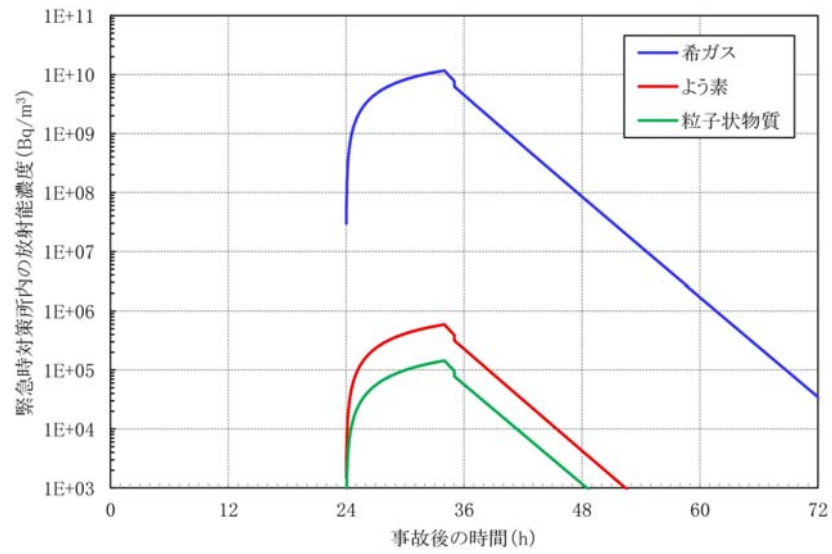
第9-1図 緊急時対策所内（浄化エリア）の放射性物質濃度の推移
