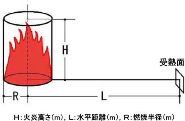
図 2.1.2-3 外部火災で想定する火災モデル
