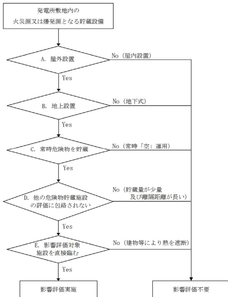
図 2.1.2-2 敷地内の評価対象抽出フロー
