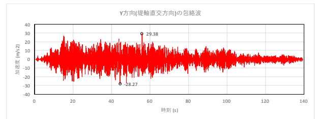
加速度応答スペクトルと時刻歴波形 (Y方向 (E W))
