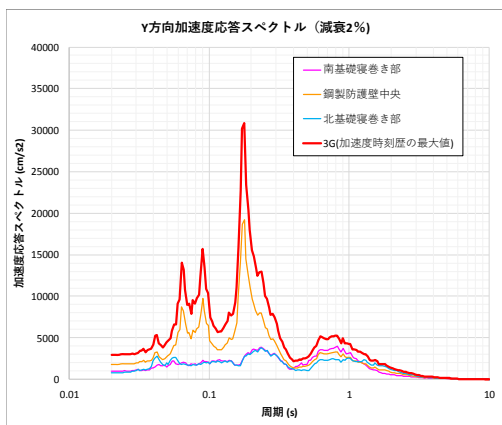
加速度応答スペクトルと時刻歴波形 (Y方向 (E W))
