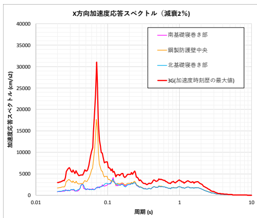
加速度応答スペクトルと時刻歴波形 (X方向 (N S))
