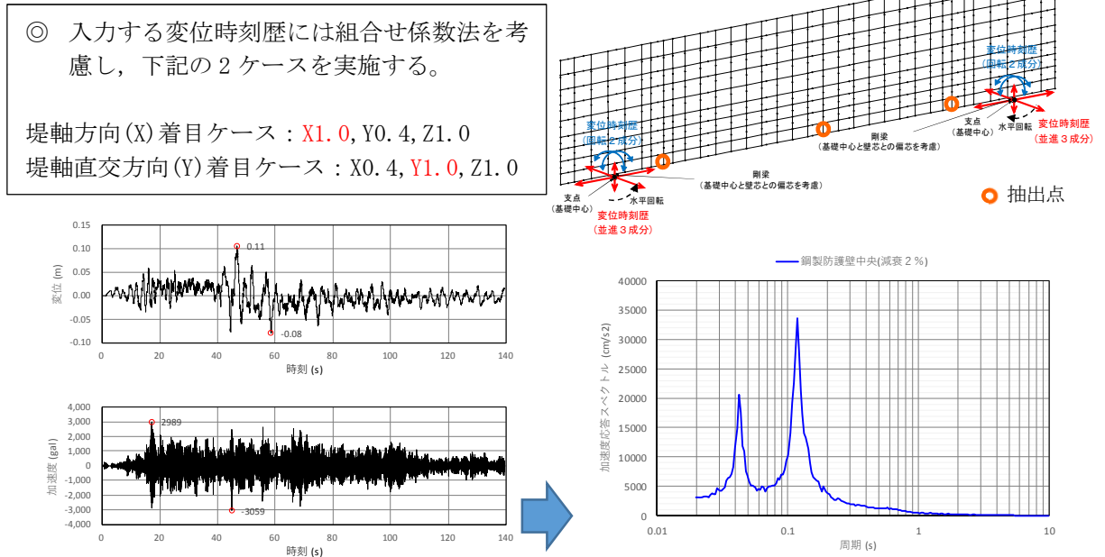
図 8 鋼製防護壁の三次元フレーム解析による中央部の応答時刻歴と応答スペクトル(鉛直方向)
