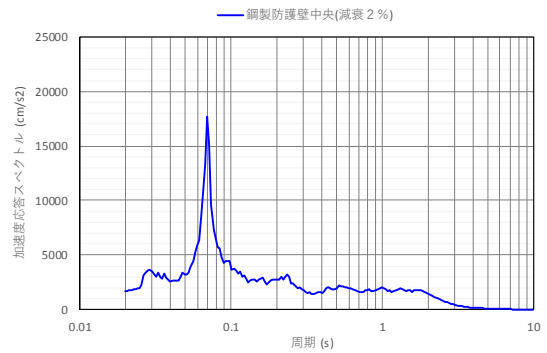
図8 鋼製防護壁の三次元フレーム解析による中央部の応答時刻歴と応答スペクトル(堤軸方向)
