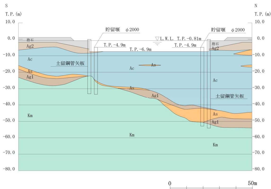
図 2.2-2 土留鋼管矢板の断面図 (NS-1)
