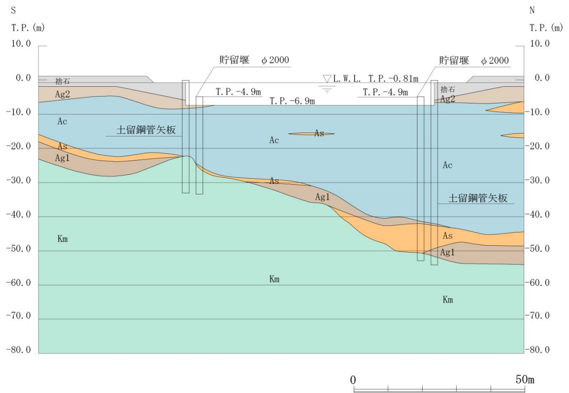
図 2.7-2 土留鋼管矢板の断面図 (NS-1)
