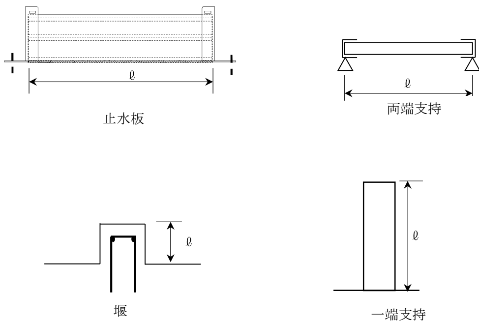
第3-1図 堰及び止水板の評価モデル図
