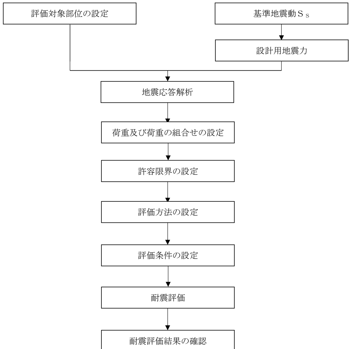
第2-9図 堰の耐震評価フロー
