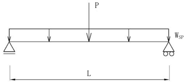
第9-13図 荷重図
