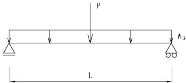
第 9-15 図 荷重図
