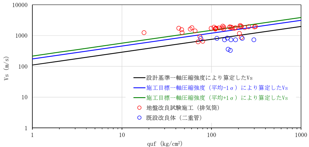
図2 地盤改良体の解析用地盤物性値 ( V_s ) と PS 検層の比較
