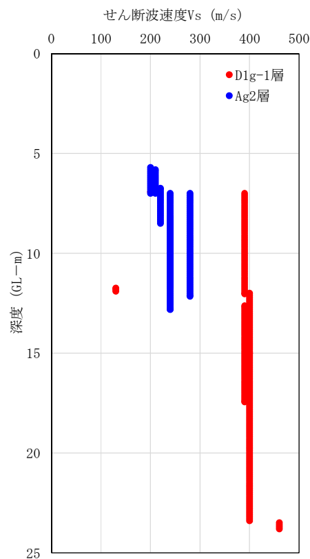
図 4 D1g-1 層と Ag2 層の PS 検層の比較
