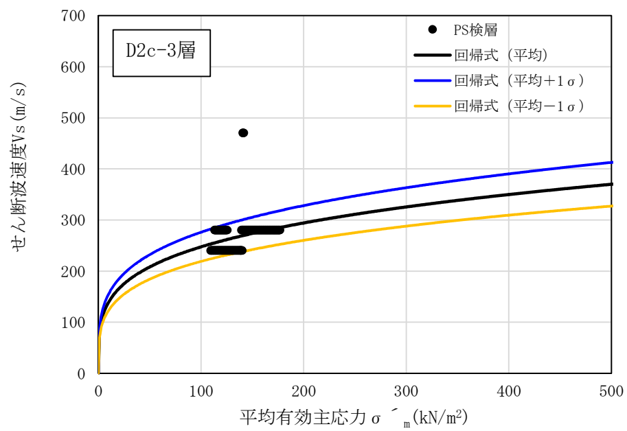
図 1.1-2 (8) V_s の \sigma'_m 依存式 (D2c-3 層)
