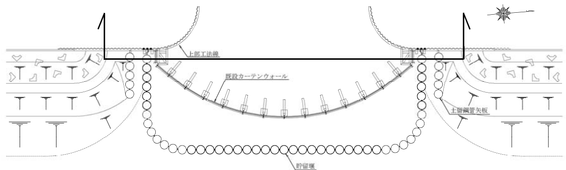
(平面図)
