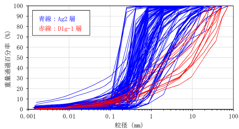
図 3 D1g-1 層と Ag2 層の粒度分布の比較
