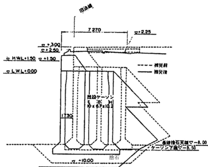
図 2 検討対象断面（神戸港第七防波堤）＊
