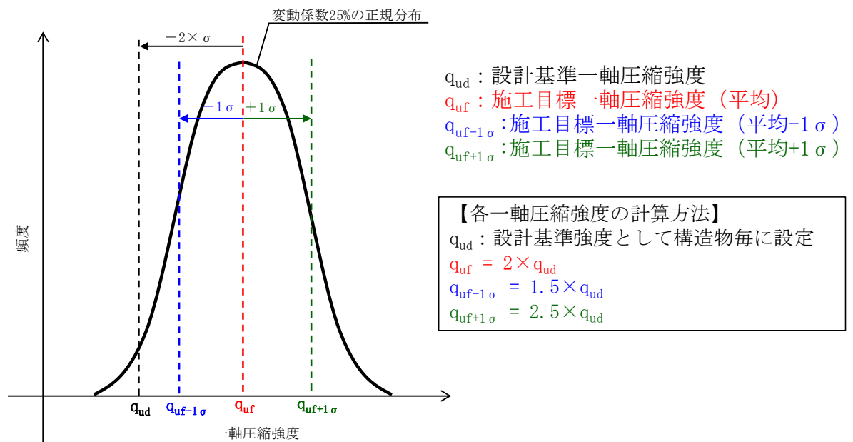
図 1 設計基準一軸圧縮強度と施工目標一軸圧縮強度及び標準偏差の関係
