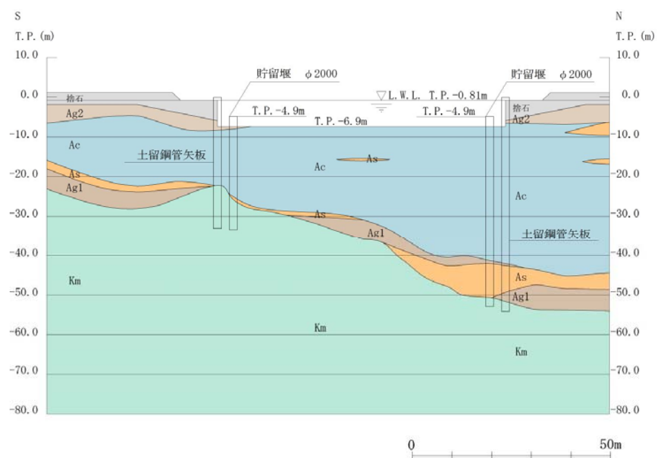
(断面図)
