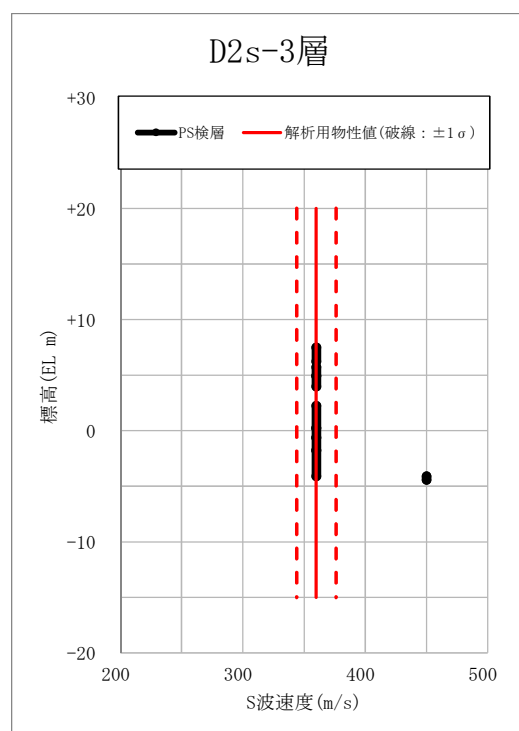
図 2-1 (4) PS 検層結果 (D2s-3 層)
