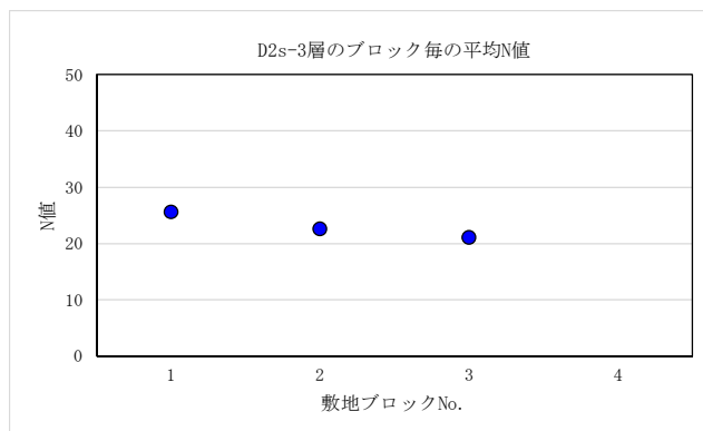
図 6.3-1 (6) 各ブロックにおける N 値の比較結果 (D2s-3 層)
