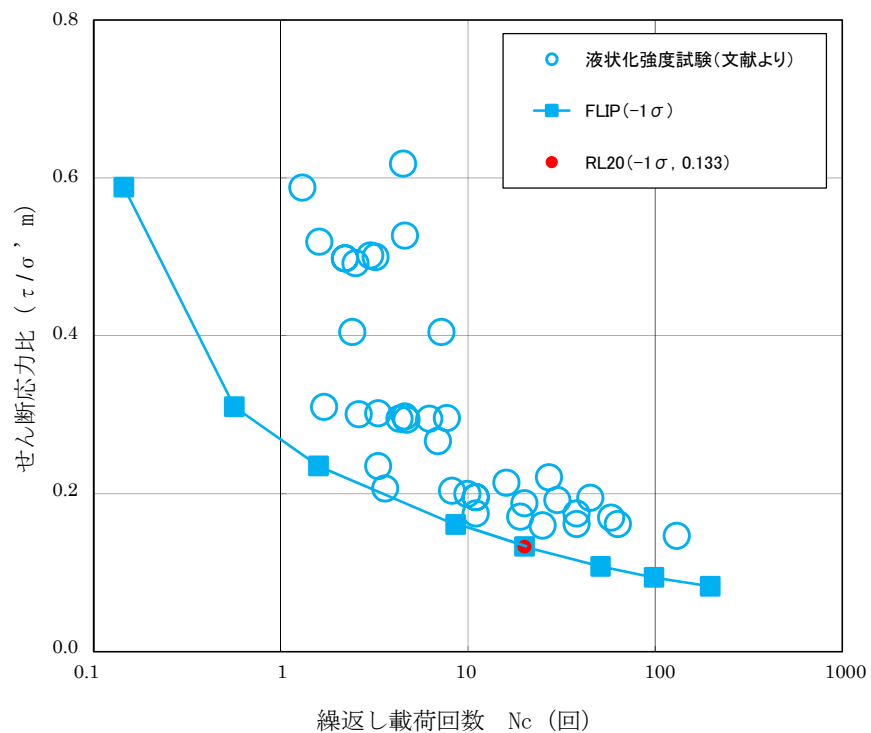
図 4.2-11 F L I P による豊浦標準砂の液状化強度特性 (-1 \sigma )
