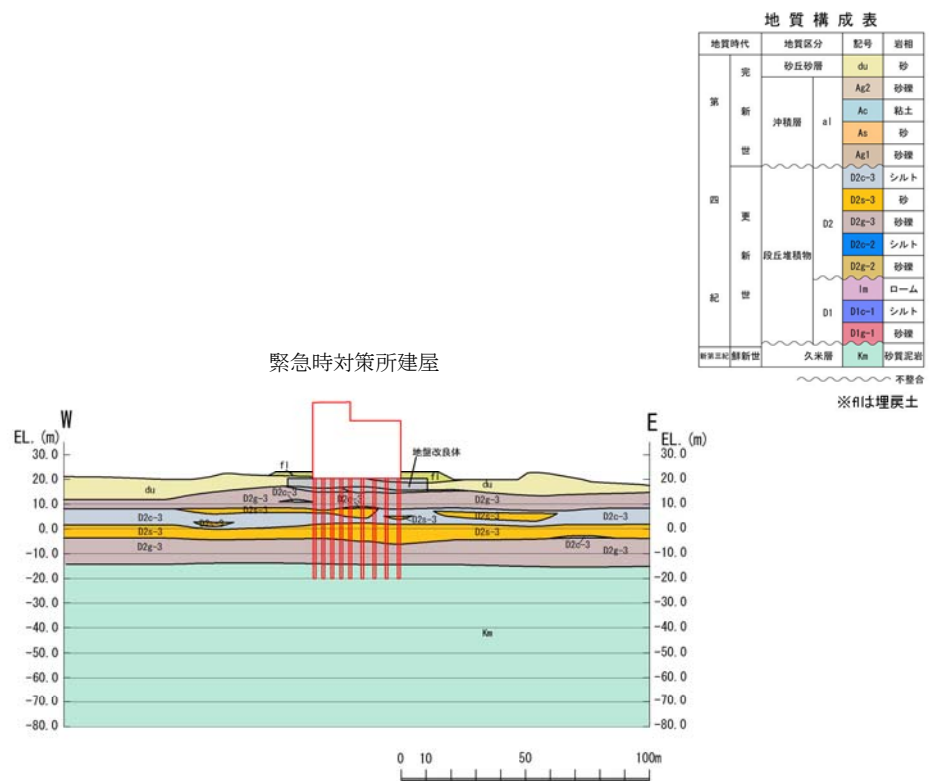
図 3.1-3 (2) 地質断面図 (2/6)
