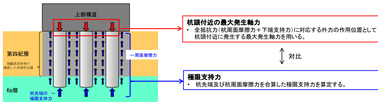
図2 杭周面摩擦力を支持力として考慮する評価の適用イメージ
