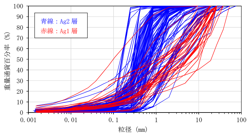
図 1 Ag1 層と Ag2 層の粒度分布の比較
