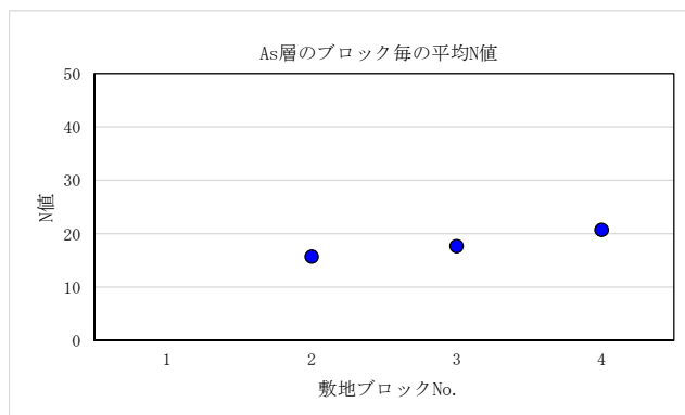
図 6.3-1 (3) 各ブロックにおける N 値の比較結果 (As 層)
