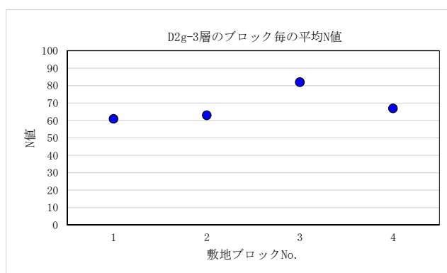
図 6.3-1 (7) 各ブロックにおける N 値の比較結果 (D2g-3 層)
