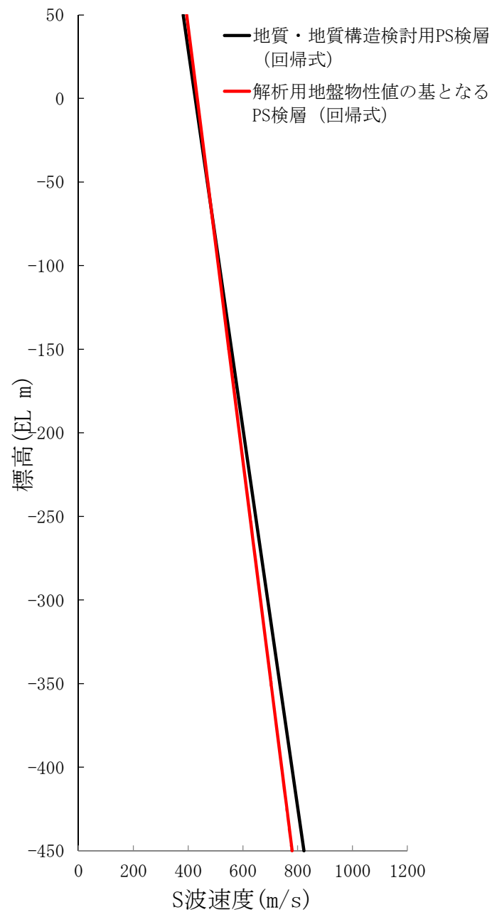
図 6.3-4 各 PS 検層の比較
