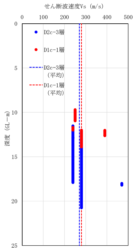
図 6 D1c-1 層と D2c-3 層の PS 検層の比較
