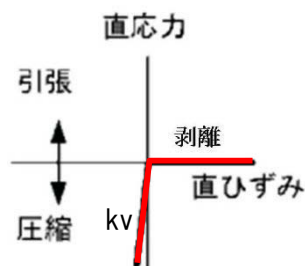
図 5 杭下端ジョイントばね設定の考え方
