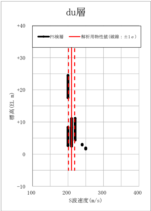
図 2-1 (1) PS 検層結果 (du 層)
