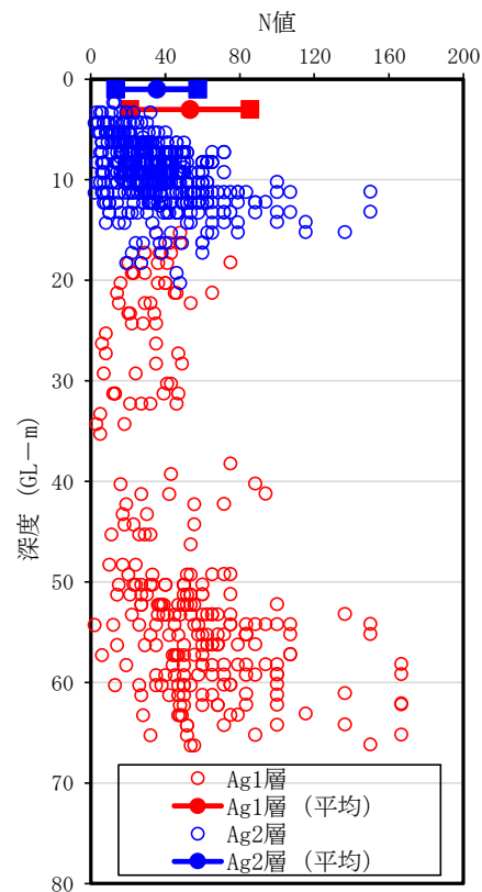
図 2 Ag1 層と Ag2 層の N 値の比較
