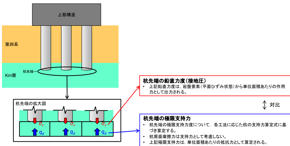
図1 杭先端の支持岩盤への接地圧算定方法
