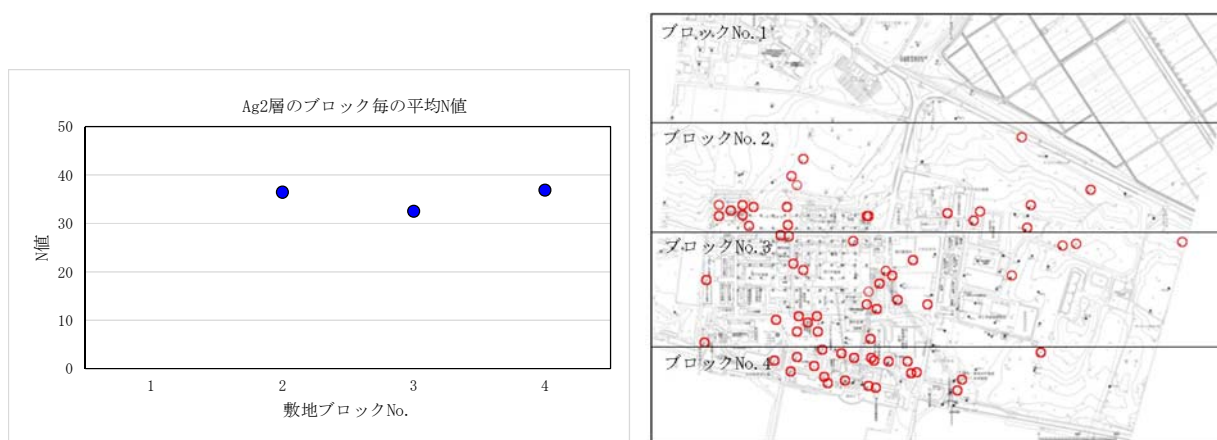
(ブロック区分と N 値の採取位置)
