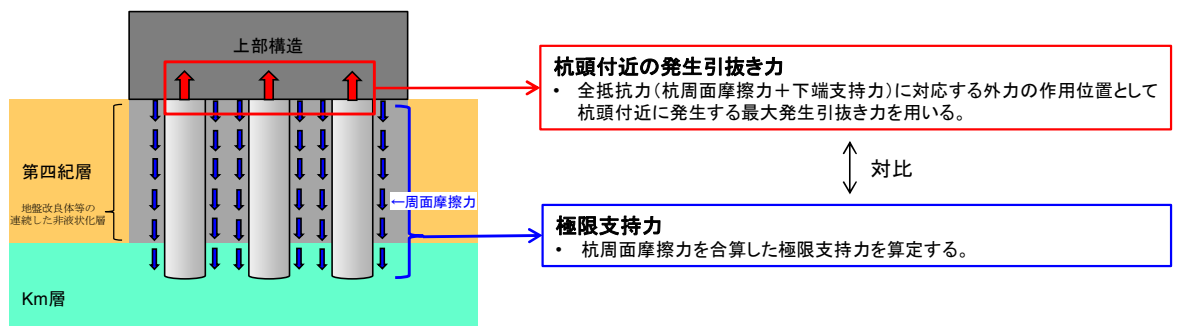
図3 引抜きに対する支持力評価のイメージ
