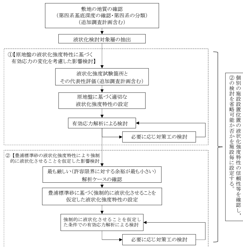
図 4.2-1 液状化影響評価のフロー
