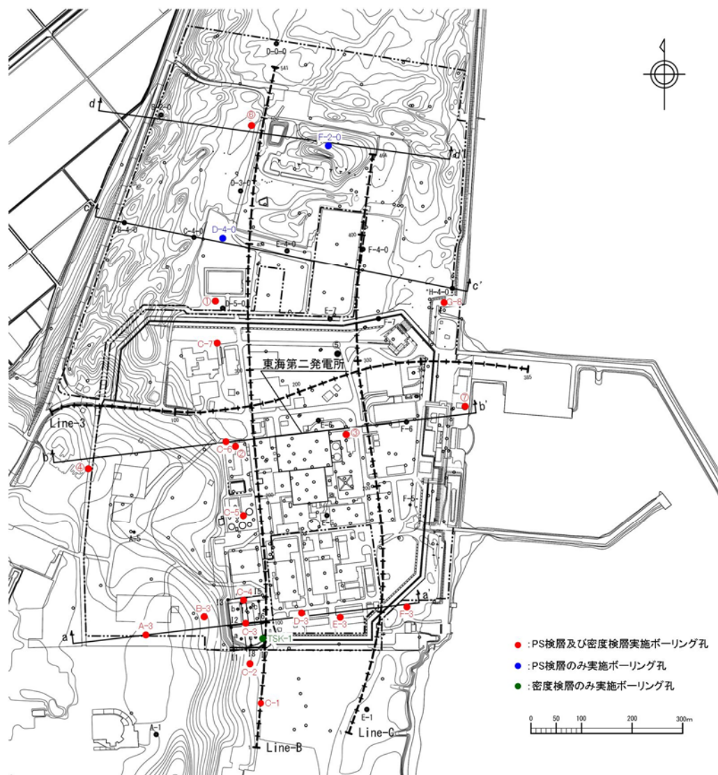
図 6.3-2 PS 検層実施位置図（敷地の地質・地質構造検討用）
