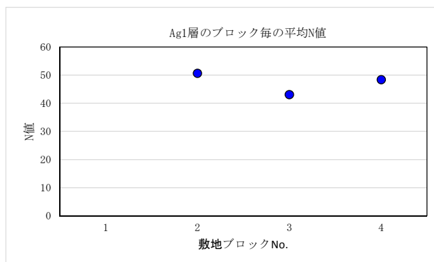
図 6.3-1 (5) 各ブロックにおける N 値の比較結果 (Ag1 層)
