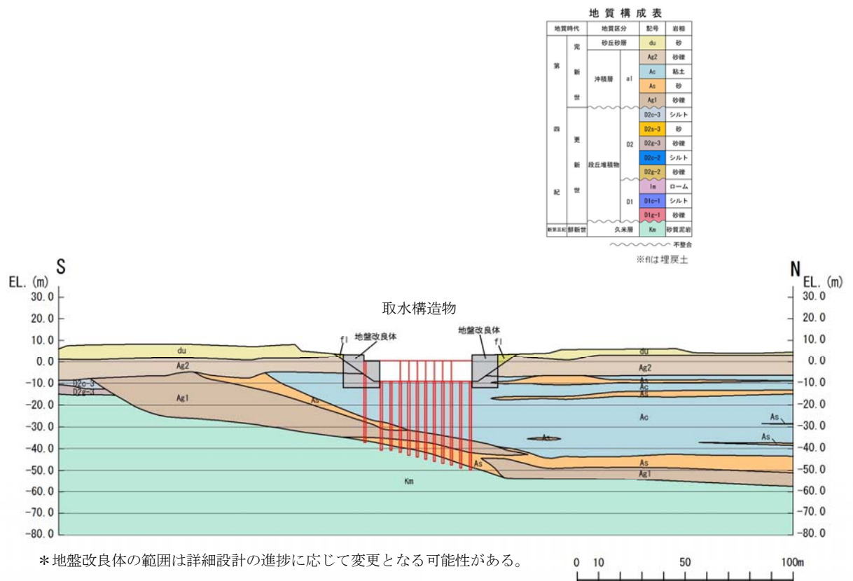
(5) 取水構造物周辺断面 (E-E 断面)
