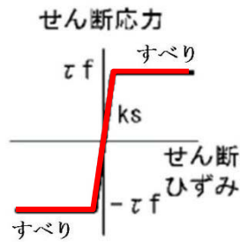
図 4 杭－地盤相互作用ばね設定の考え方
