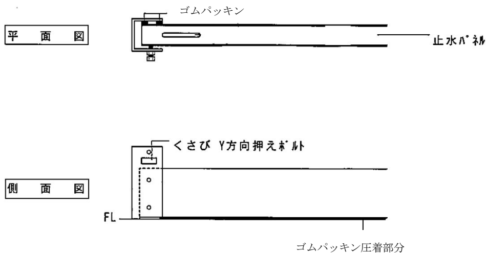
第4-4図 止水板の概要図
