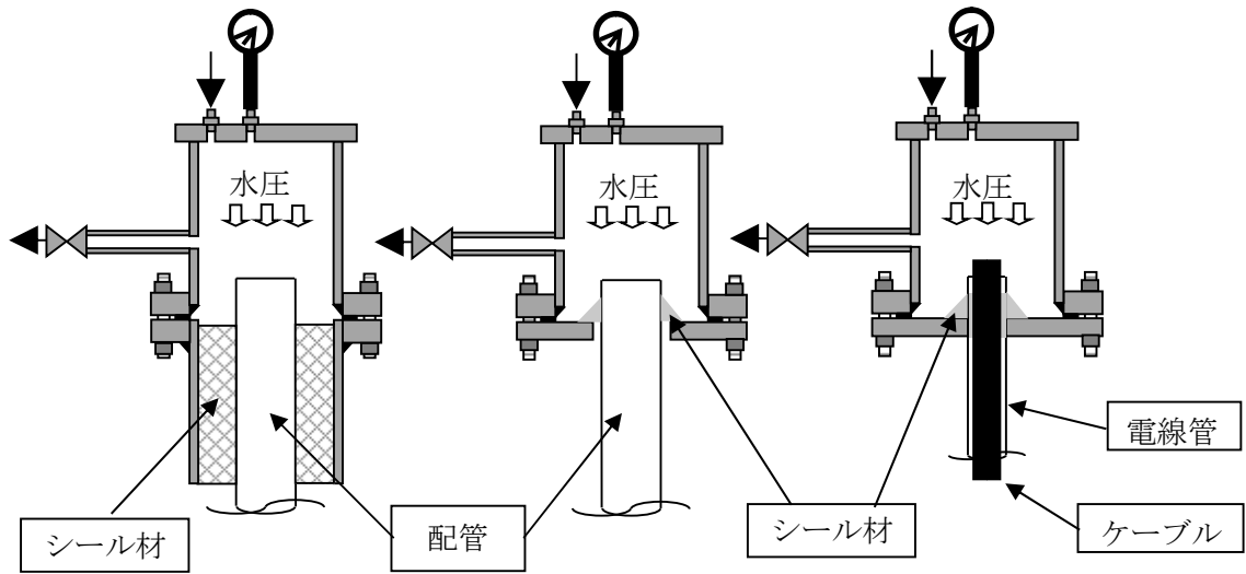
第4-9図 シール材の耐圧漏えい試験の概要
