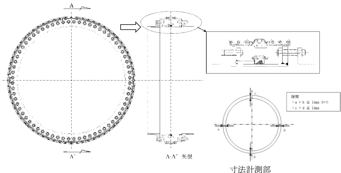
第4-14図 循環水管可撓継手設置時のすき間管理について
