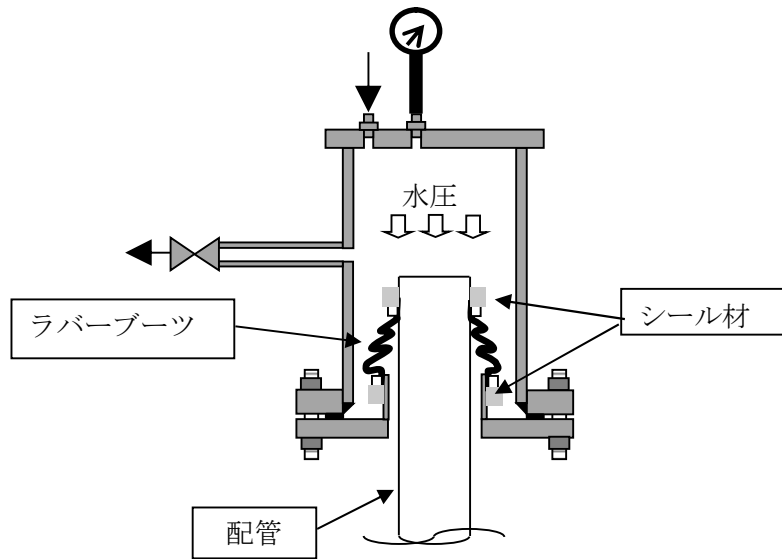
第4-9図 シール材の耐圧漏えい試験の概要
