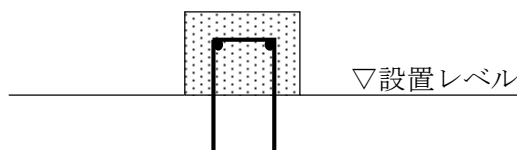
第4-2図 溢水拡大防止堰の概要図
