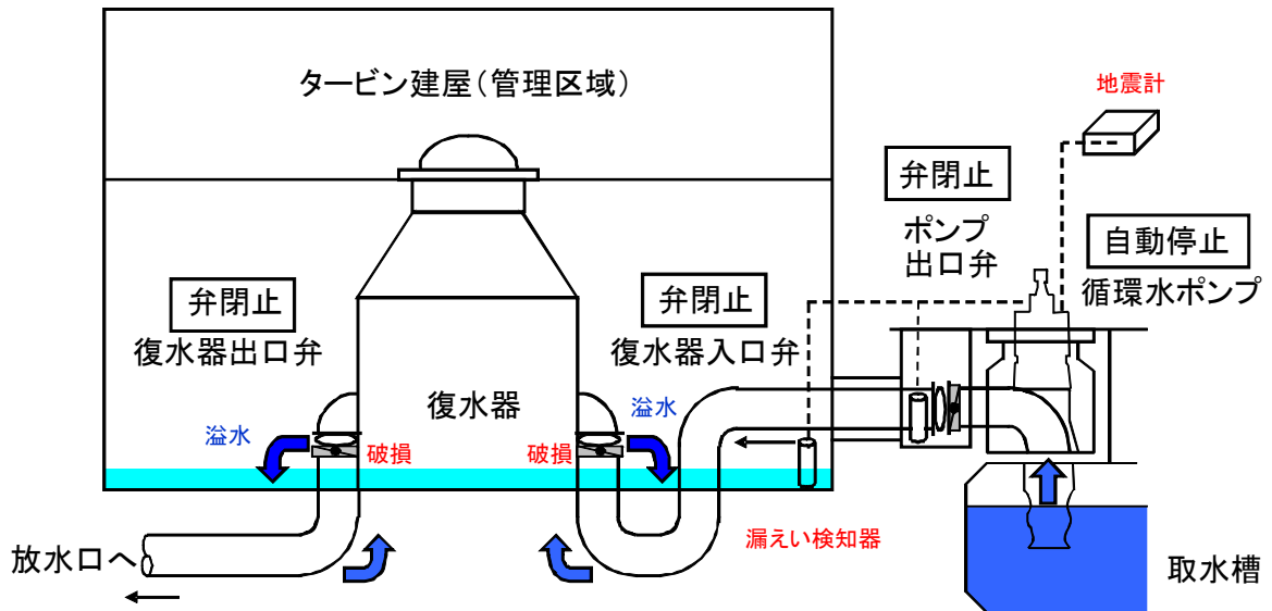
第4-12 図 設備概要
