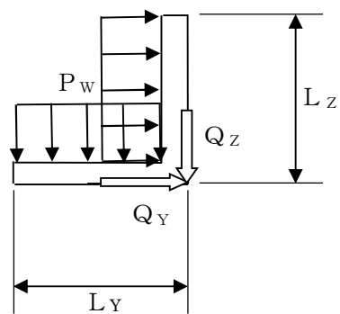
第3-9図 梁材に生じる力の模式図
