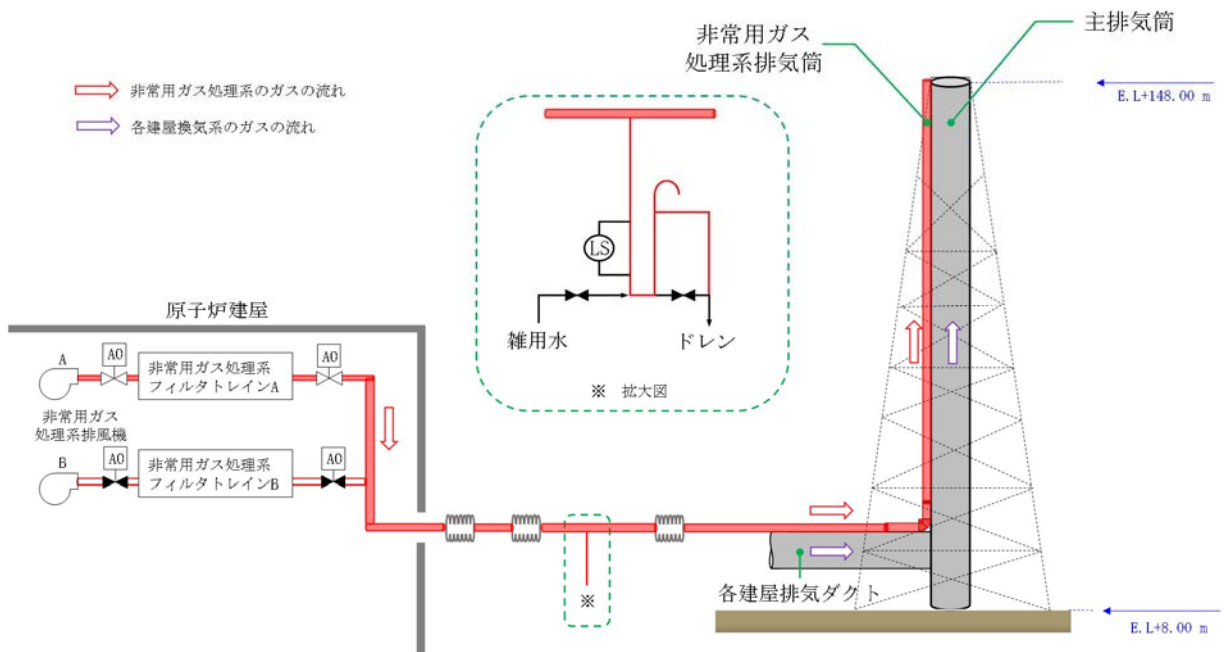
第 2. 2. 1-2 図 排気筒及び非常用ガス処理系排気筒の位置関係
