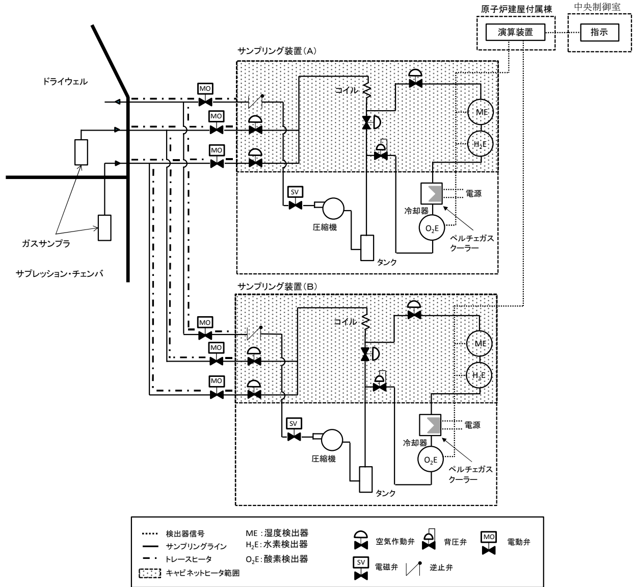
第 2-2 図 格納容器内水素濃度 (S A) 及び格納容器内酸素濃度 (S A) 系統概要図
