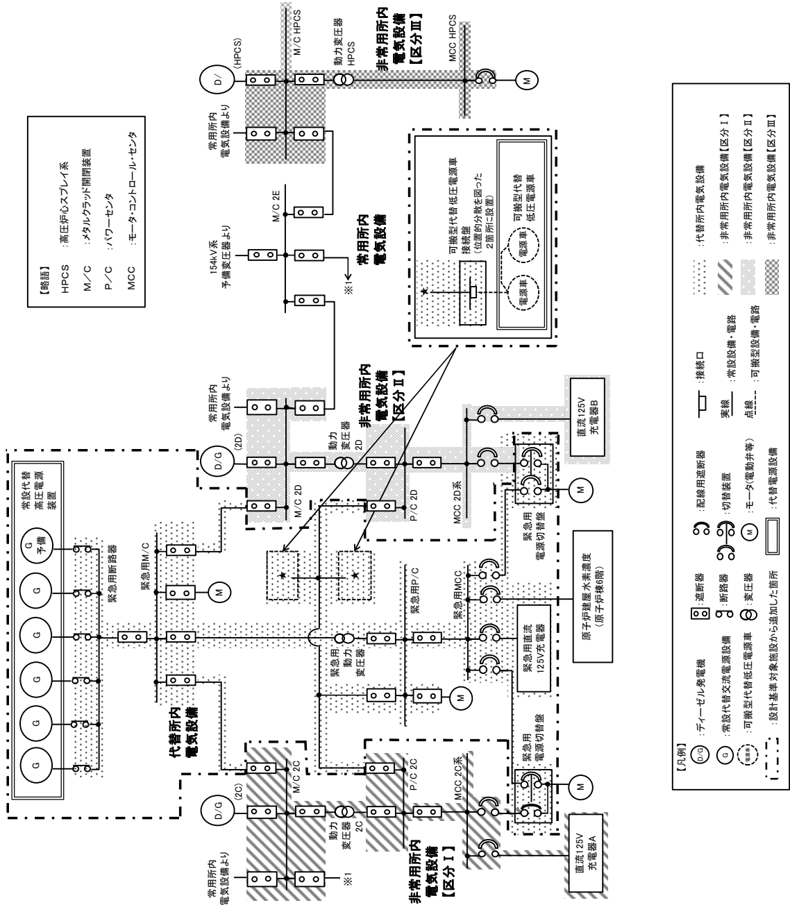
第3.4-5図 単線結線図 (交流電源設備)
