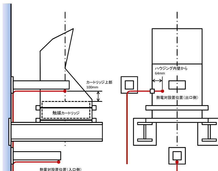
第4-4図 静的触媒式水素再結合器への熱電対取付位置概要図
