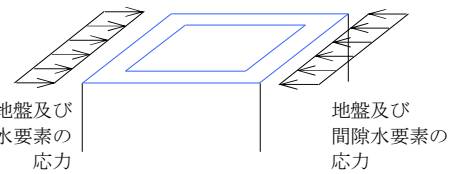
矩形立坑
