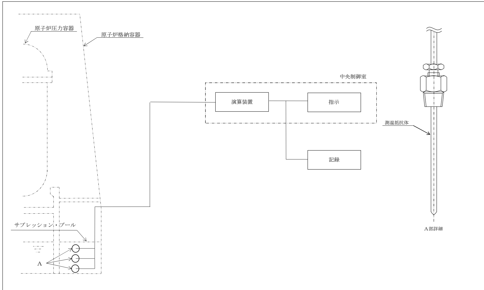
図 3-1-4-6 検出器の構造図（サブプレッション・プール水温度）
