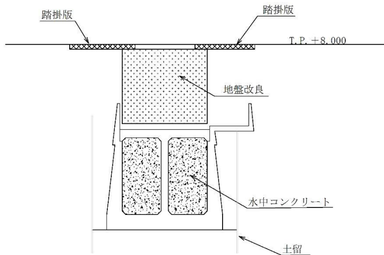
タイプD (踏掛版)
