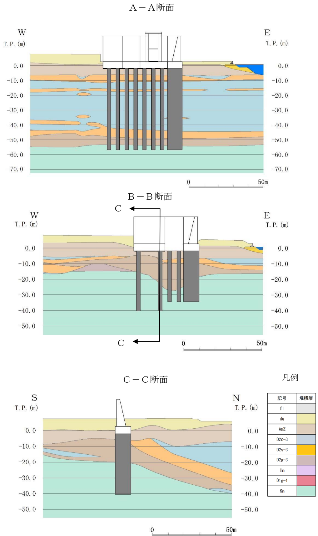
第3-9図 側方流動の評価範囲 (2/2)
