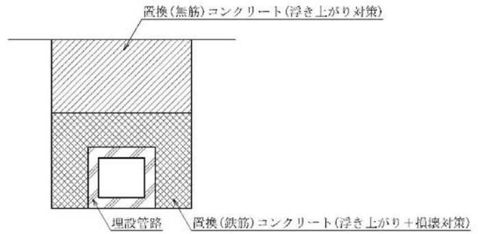
タイプA (置換コンクリート)
