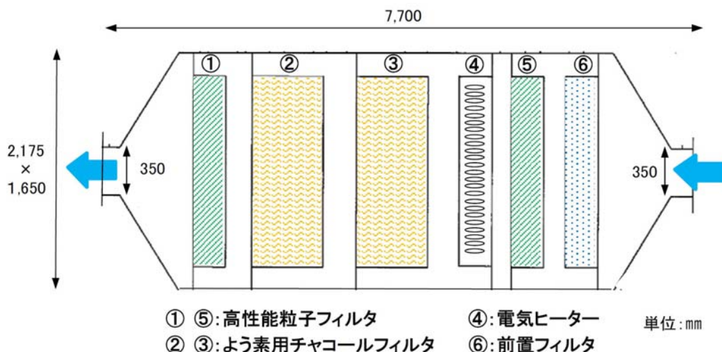
第3-3図 非常用フィルタ装置の概要図
