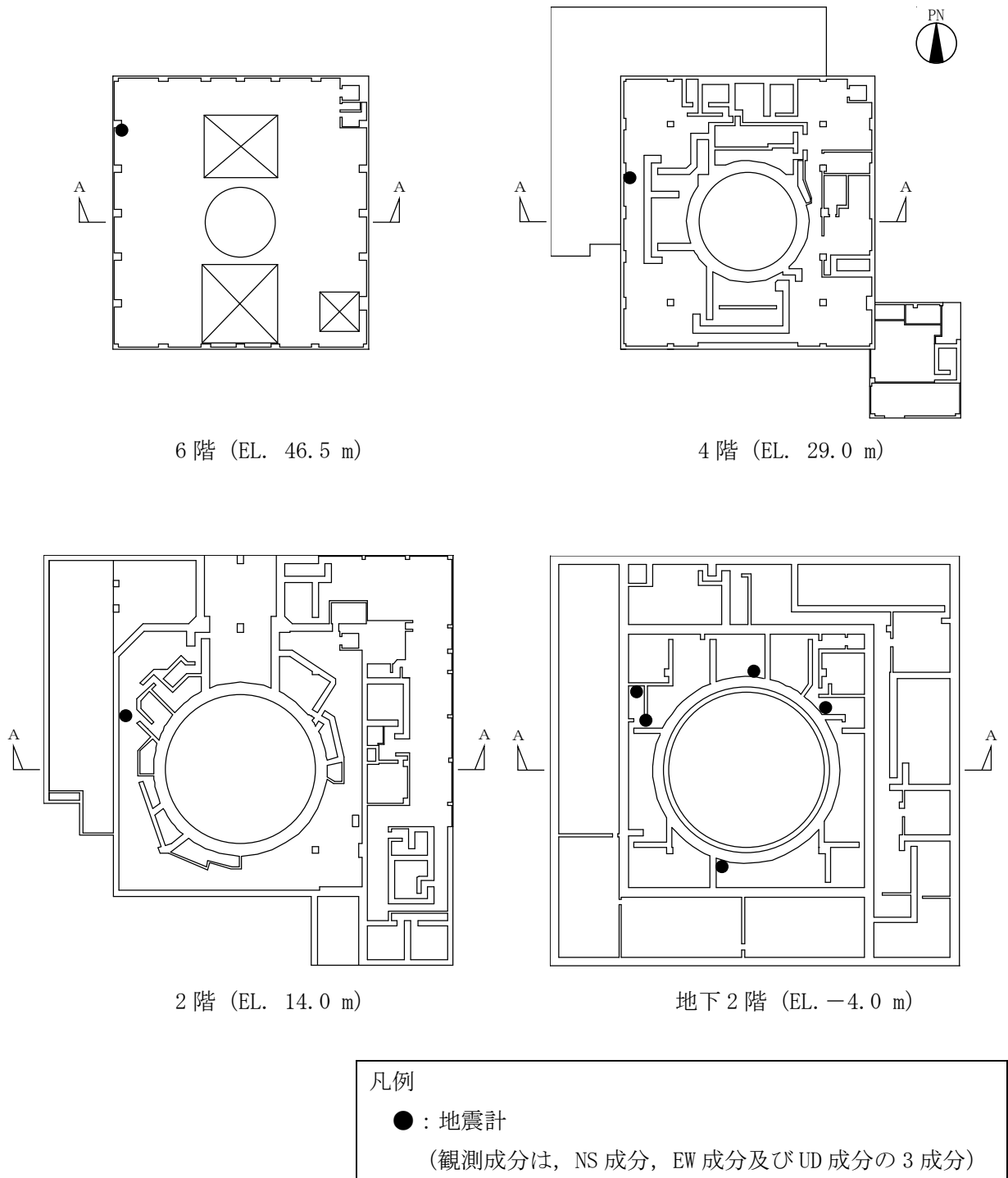
図 3-1 地震計配置図 (平面図) (原子炉建屋)
