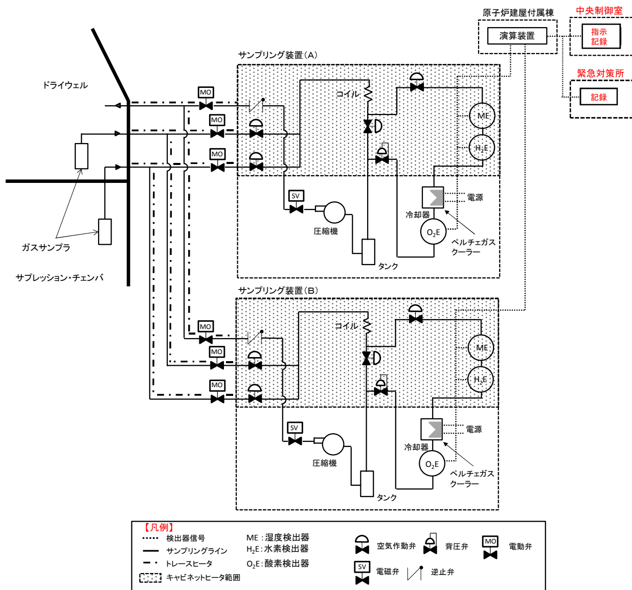
第 2-4 図 格納容器内水素濃度（S A）及び格納容器内酸素濃度（S A）系統概要図
