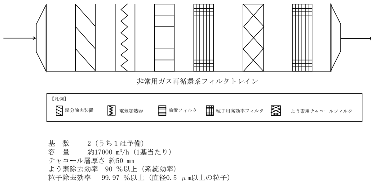
第 4-1 図 非常用ガス再循環系フィルタトレインの構成
