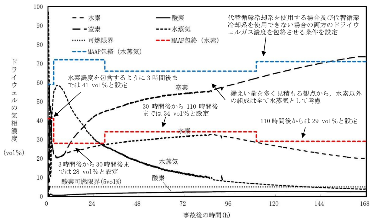
第 2.3.1-6 図 ドライウェルガス濃度（有効性評価シナリオ包絡条件） （代替循環冷却系を使用する場合）
