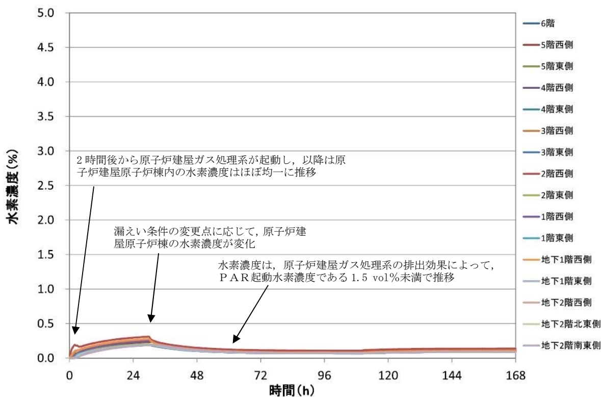
第 2.3.2-1 図 ケース 1 水素濃度の時間変化（原子炉建屋原子炉棟全域）
