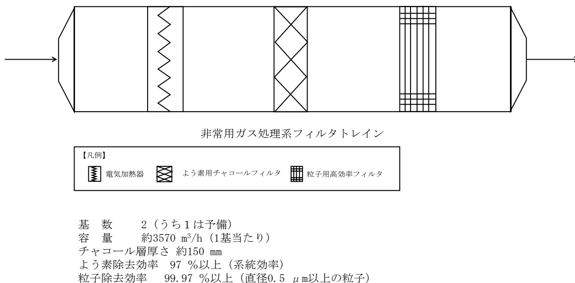
第 4-2 図 非常用ガス処理系フィルタトレインの構成
