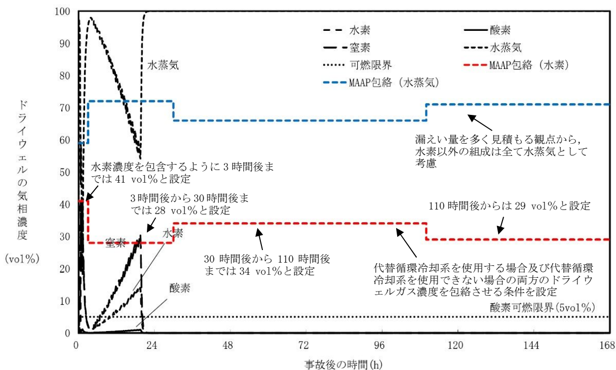
第 2.3.1-7 図 ドライウェルガス濃度（有効性評価シナリオ包絡条件） （代替循環冷却系を使用できない場合）
