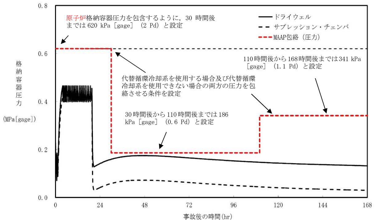
第 2.3.1-3 図 格納容器圧力（有効性評価シナリオ包絡条件） （代替循環冷却系を使用できない場合）
