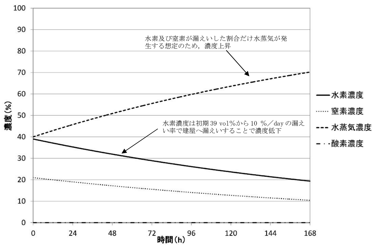
第 2.3.1-1 図 漏えいガス組成の時間変化（設計条件）
