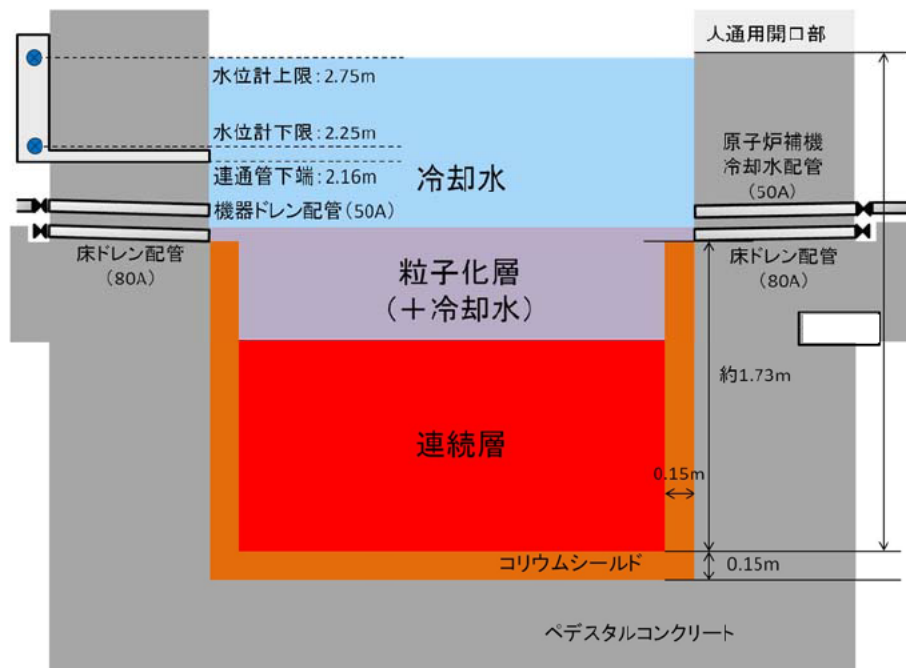
第1図 デブリ堆積イメージ図
