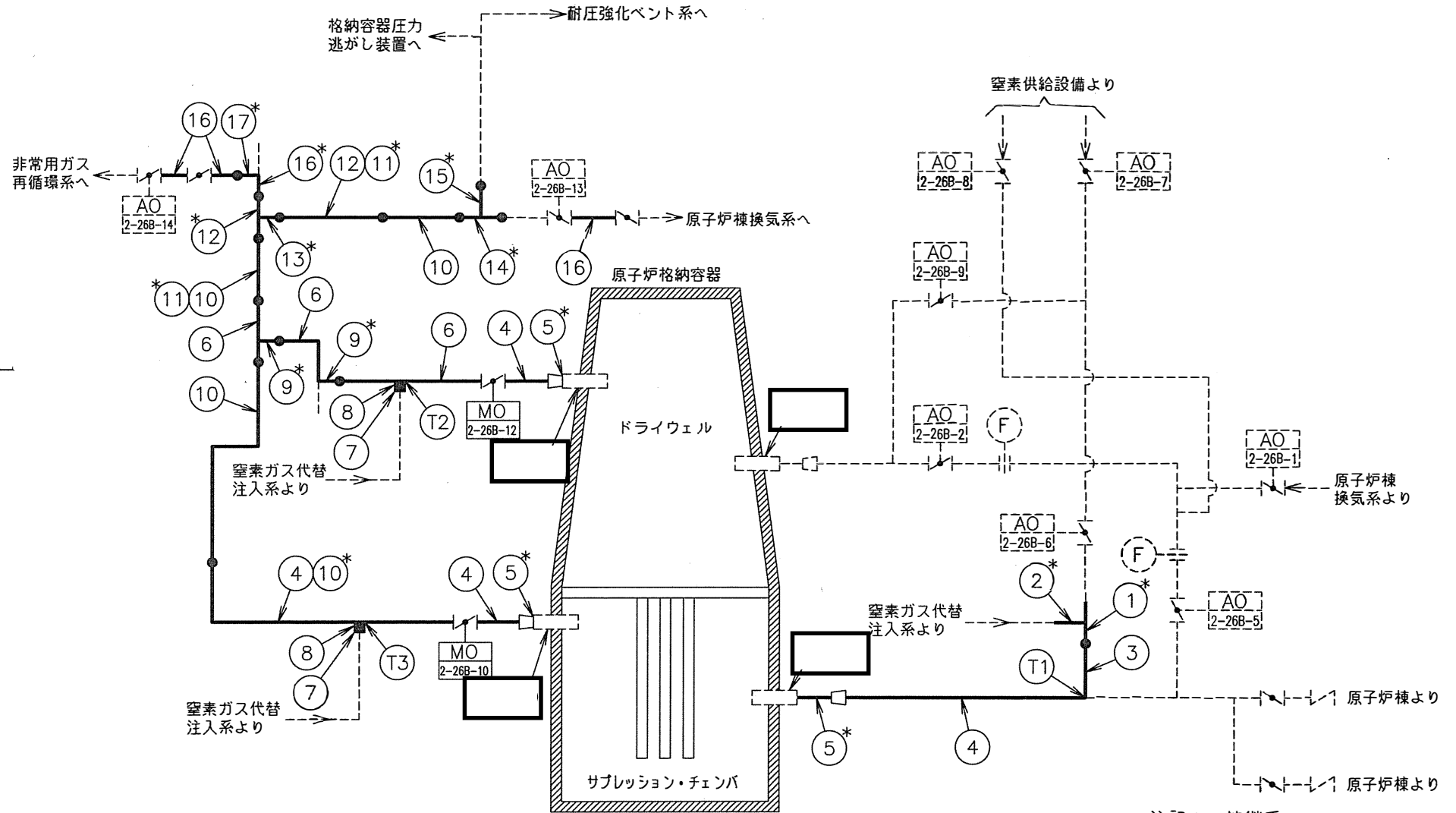
注記*：管継手 不活性ガス系概略系統図
