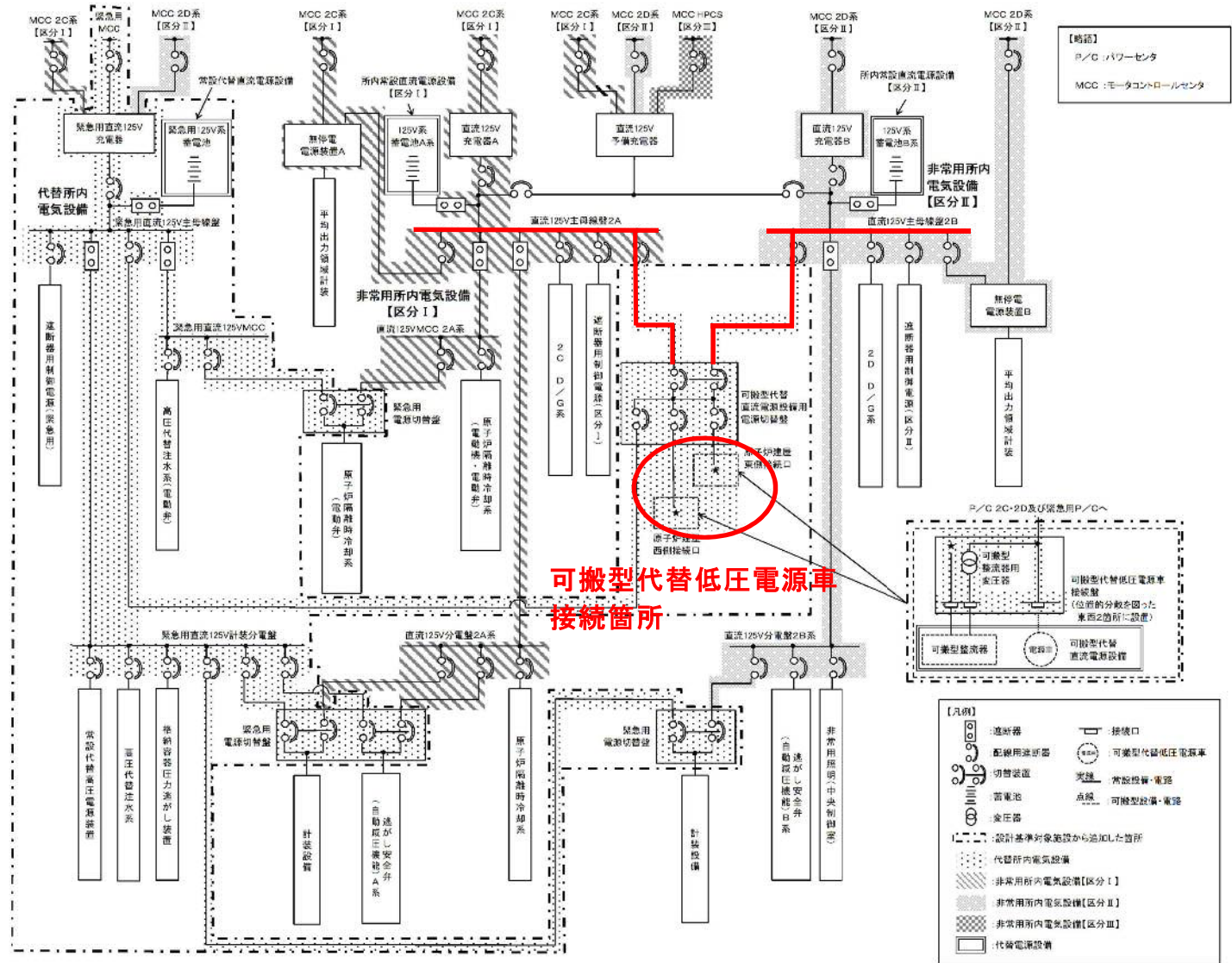
第 2 図 可搬型代替低圧電源車による非常用所内電気設備（125V 主母線盤）への電力供給経路図
