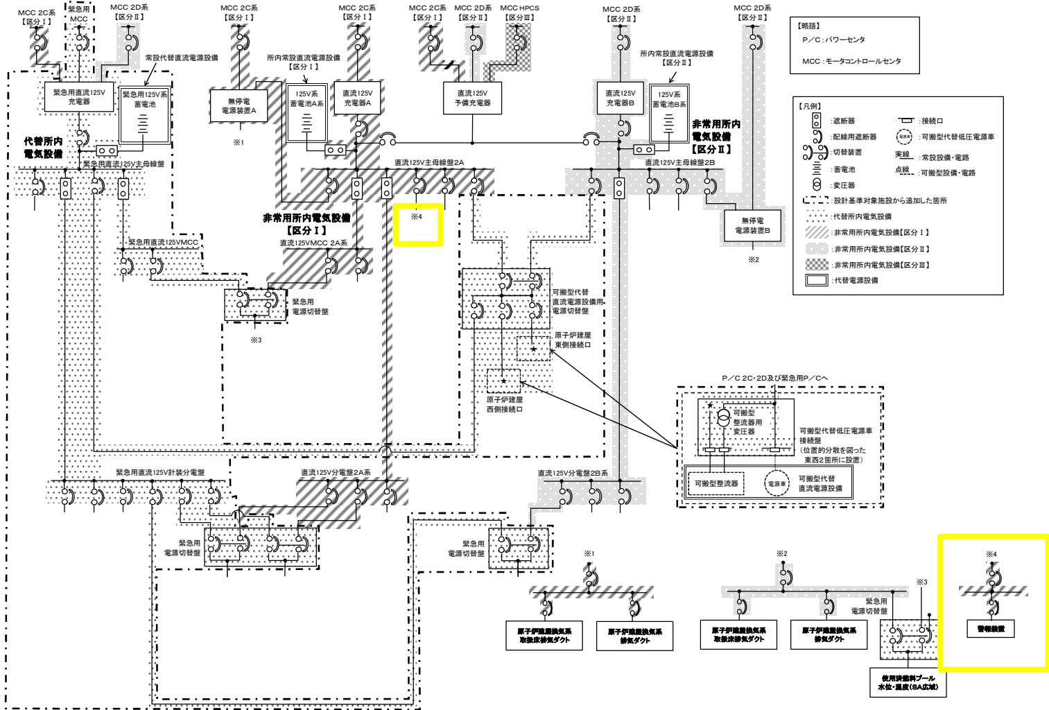
第 1.4-2 図 計測装置の電源構成概略図 (直流)
