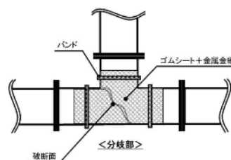
中央制御室空調ダクト分岐部における修復方法 ・ゴムシート+金属金網（メッシュ）により補強，バンドにて固定
