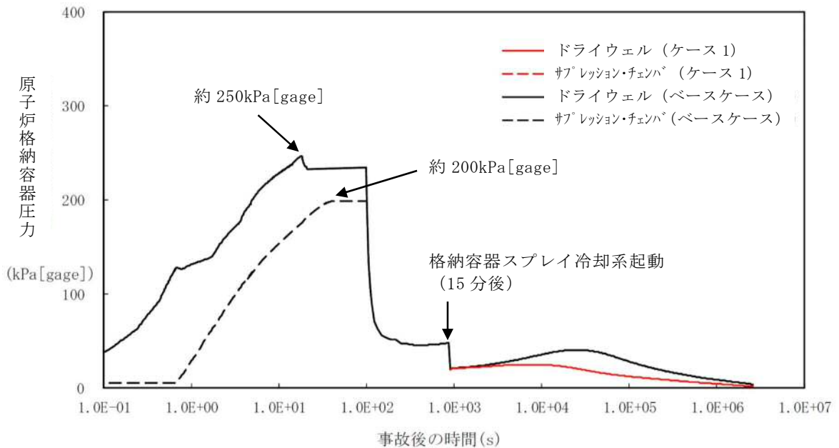
第2図 代替性確認評価ケース1とベースケースの 評価結果比較（原子炉格納容器圧力）
