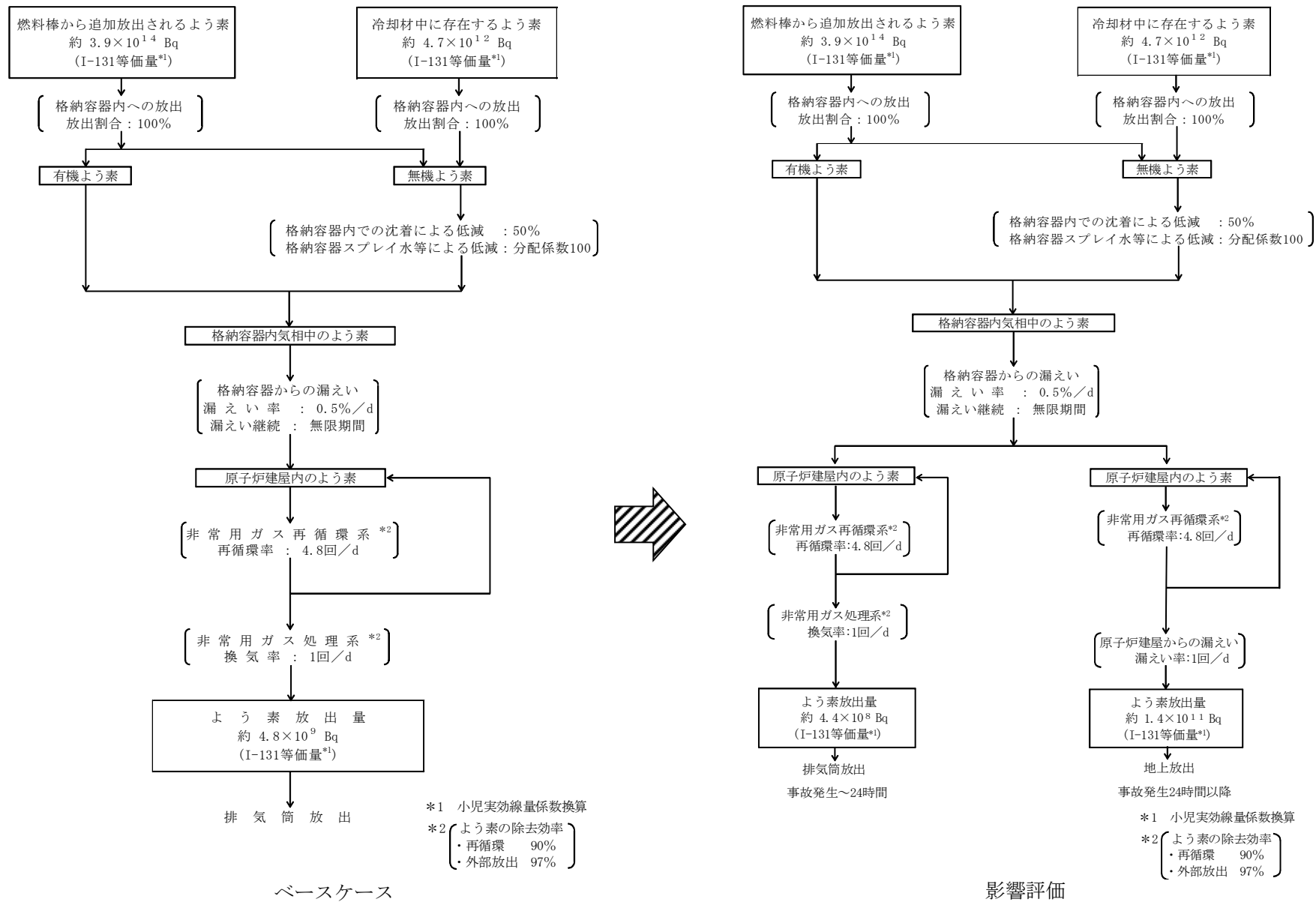
第3図 原子炉冷却材喪失時の放射性よう素の大気放出過程
