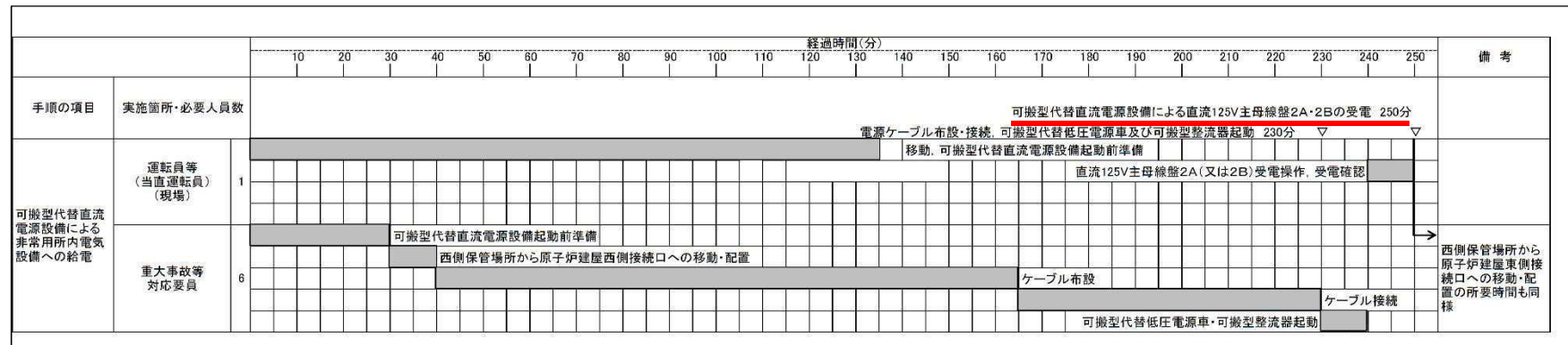
第4図 可搬型代替低圧電源車による非常用所内電気設備(直流125V主母線盤)への電力供給タイムチャート※1
