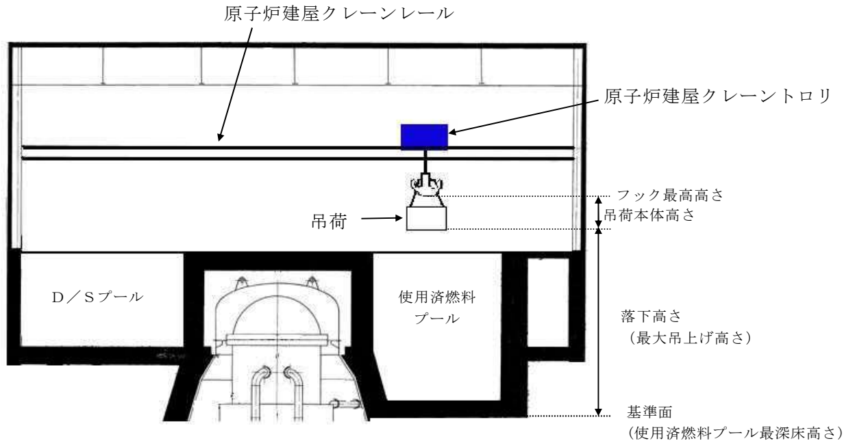
第 4.1-1 図 落下高さ算出概要
