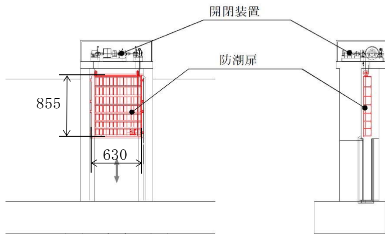
第 11 図 防潮扉の寸法図
