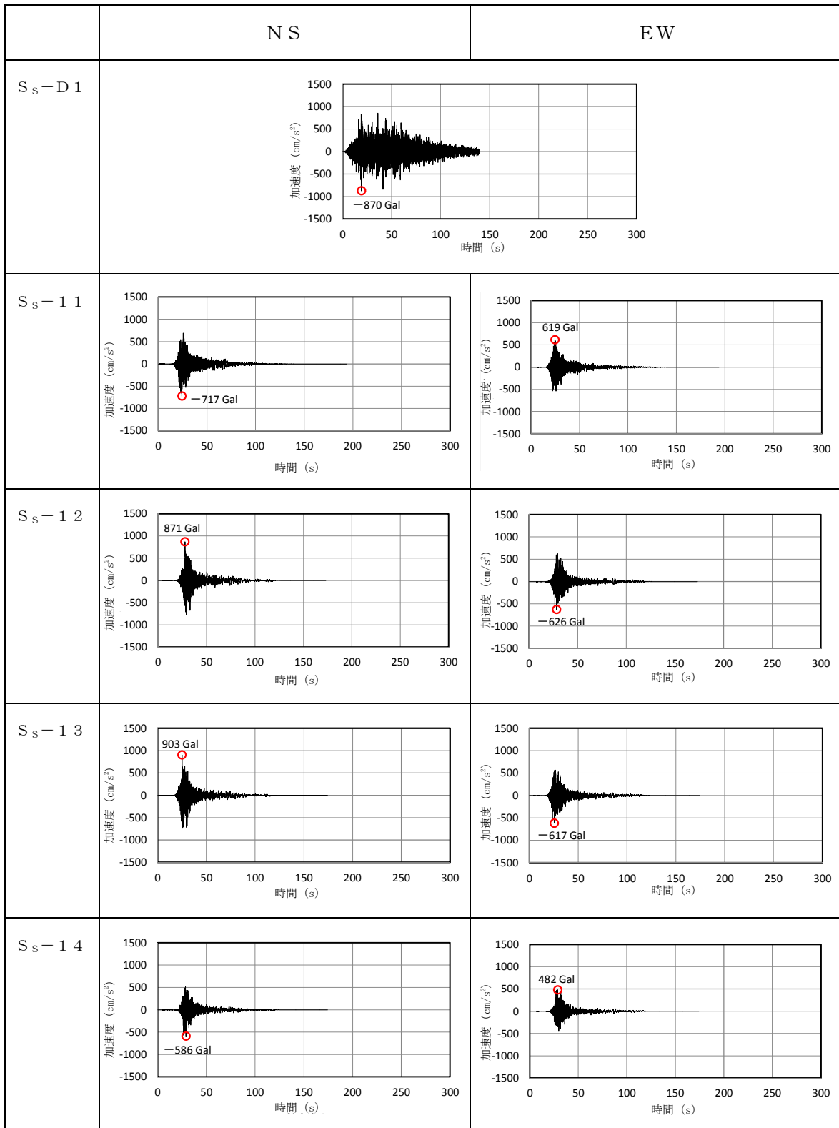
第 3-4 表 基準地震動 S_s の加速度時刻歴波形 (1/2)
