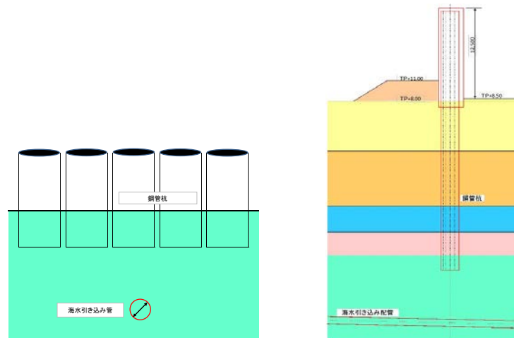
第 1-39 図 海水引込み管位置図
