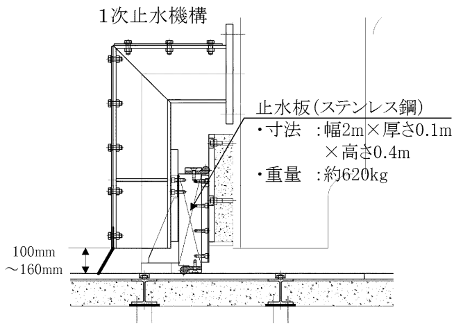
(1次止水機構拡大図)
