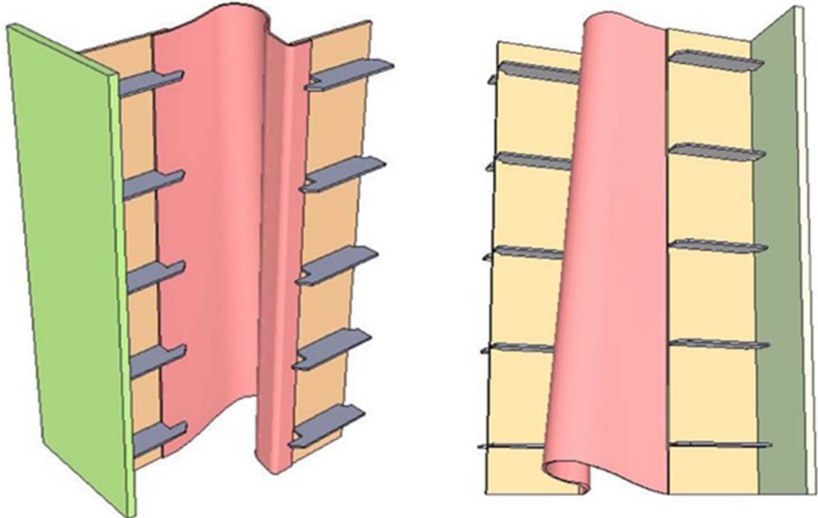
第 2-4.3 図 止水ジョイントの変形のイメージ (その 2)
