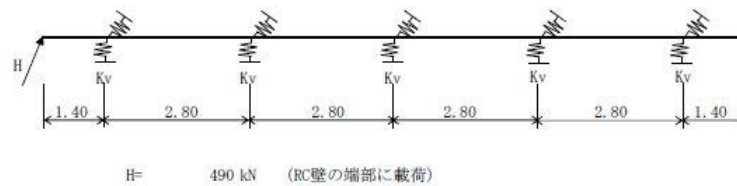
第 3-70 図 漂流物荷重 (水平)
