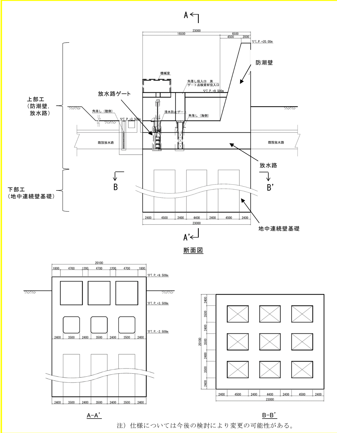
第3図 鉄筋コンクリート防潮壁（放水路エリア）構造図
