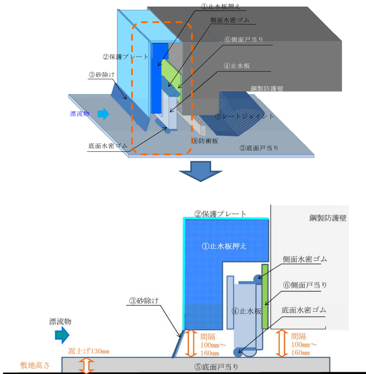
第 1-71 図 止水機構の構成部材の寸法
