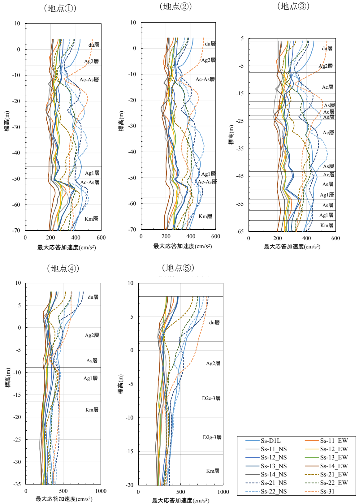
第 3-6 图 最大応答加速度分布
