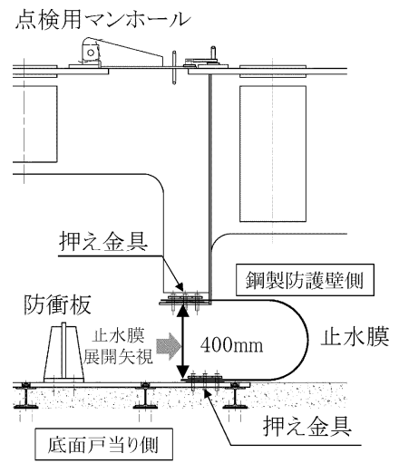
(点検用マンホール設置図)
