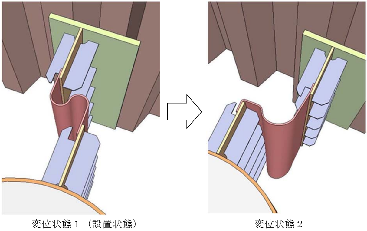
第 2-4.2 図 止水ジョイントの変位のイメージ (その 1)
