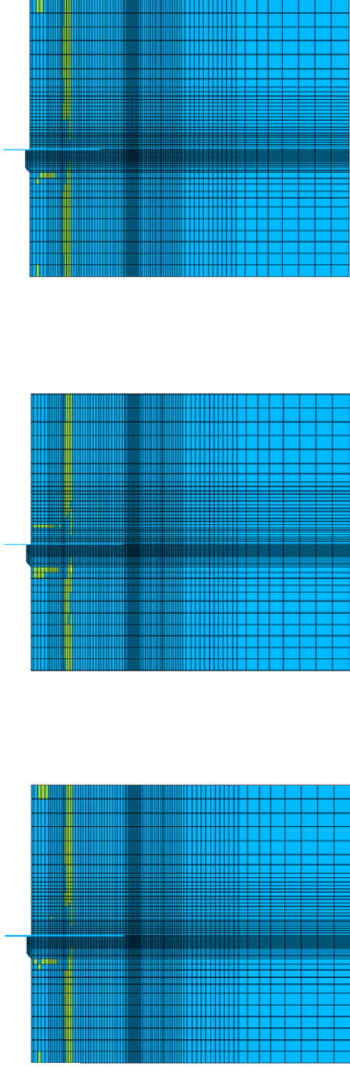
第 3-23 図 最大せん断ひずみ分布図 (岩盤傾斜部, 原地盤物性)
