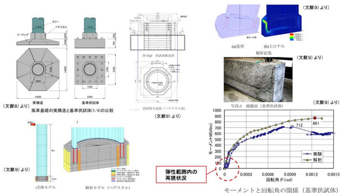
第 1-55 図 鋼製タワー基礎の载荷実験の再現解析結果
