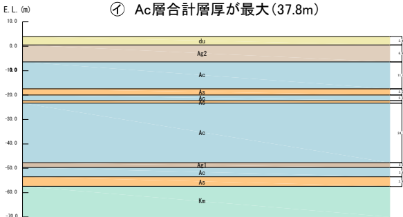
第 3-11 図 北側エリアにおける粘土層の層厚分布図
