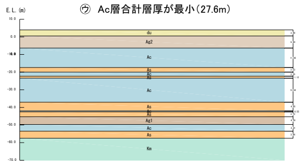
第 3-11 図 北側エリアにおける粘土層の層厚分布図
