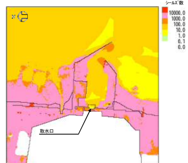
最大シールズ数分布
