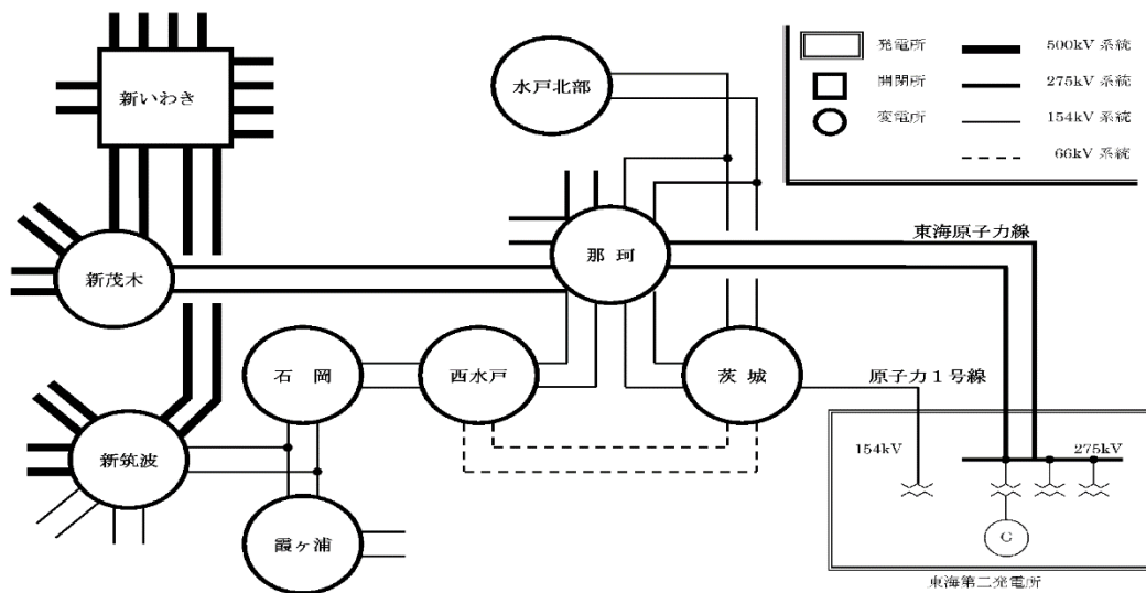
図 1 送電系統図
