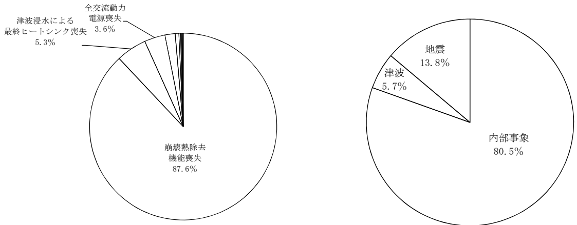
事故シーケンスグループ別 事象別 第1-7図 プラント全体の炉心損傷頻度
