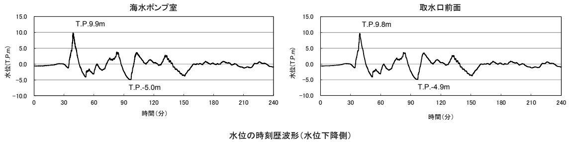
水位の時刻歴波形(水位下降側)
