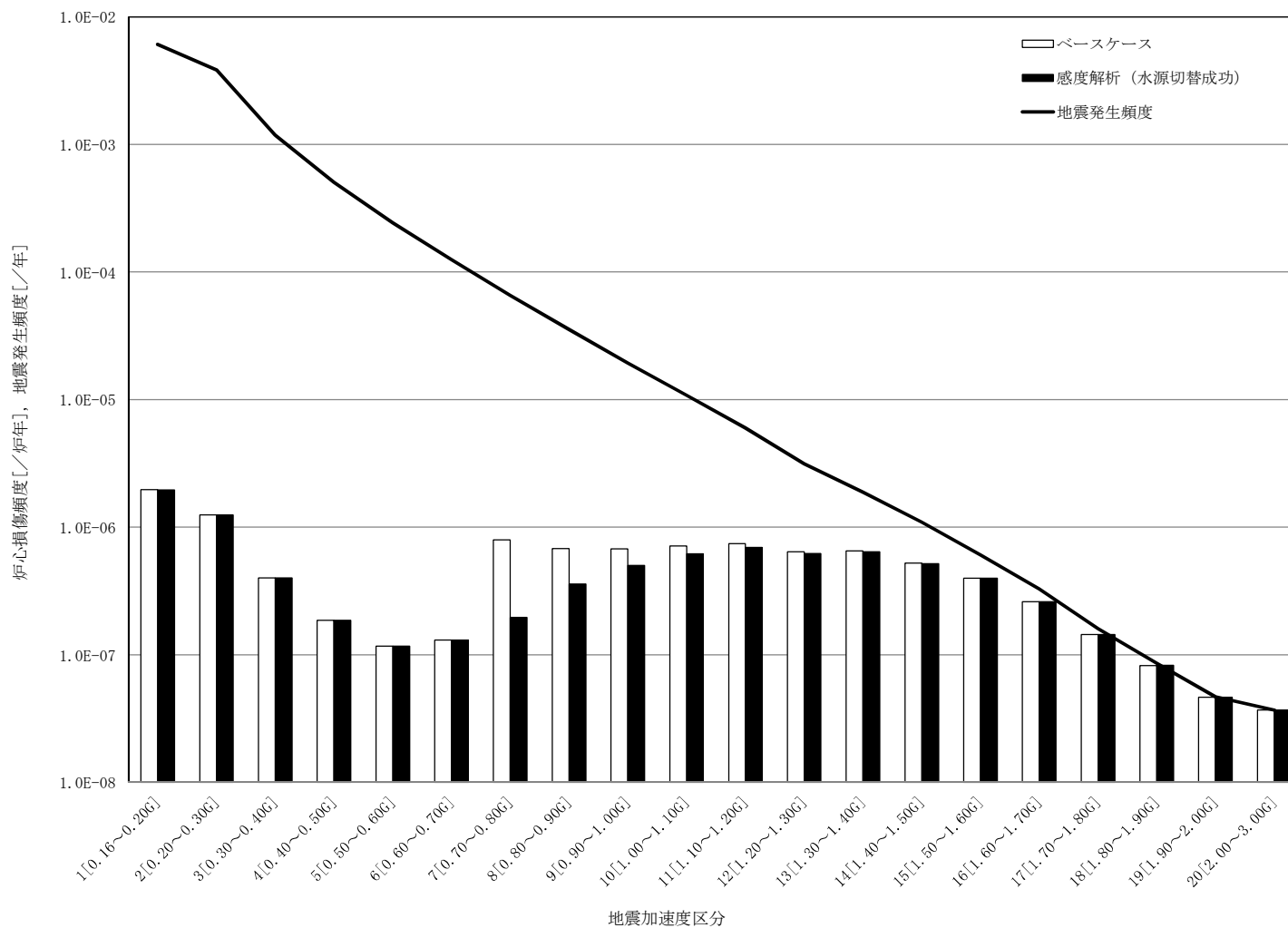
図3 地震加速度区別炉心損傷頻度（高圧注水系の水源切替のモデル化方法に関する感度解析）
