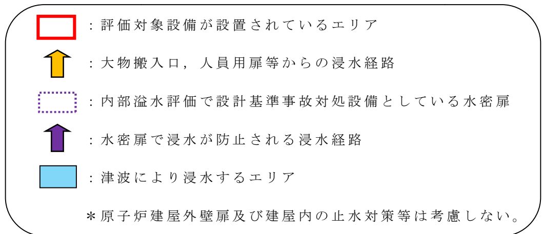
図 7 東海第二発電所 原子炉建屋地下 2 階 (EL. -4.0m)
