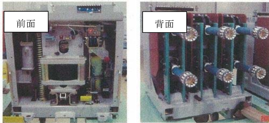
第41-1-13図 真空遮断器外観
