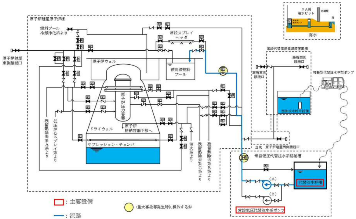
第10-1図 代替燃料プール注水系（注水ライン）の系統概略図（1/3）
