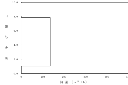
原子炉隔離時冷却系 ポンプによる注水特性
