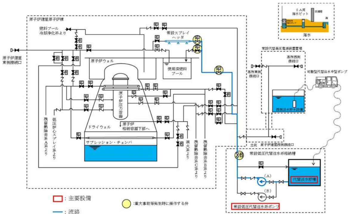
第10-2図 代替燃料プール注水系（常設スプレイヘッド）の系統概略図（2/3）
