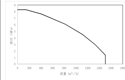
高圧炉心スプレイ系 ポンプによる注水特性
