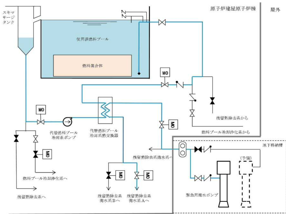
第 10-3 図 代替燃料プール冷却系，残留熱除去系及び燃料プール冷却浄化系の系統概略図 (3/3)
