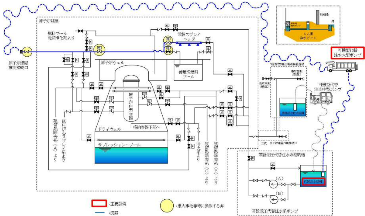
第25-2図 代替燃料プール注水系（常設スプレイヘッダ）の系統概略図
