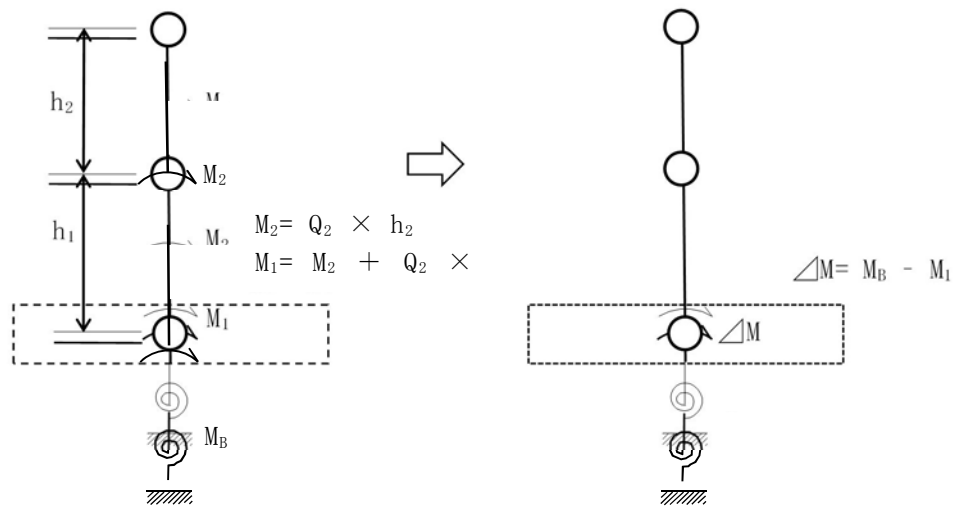
(b) 地盤の最大応答回転ばね反力 M_B と基礎スラブの補正モーメント \Delta M の関係
