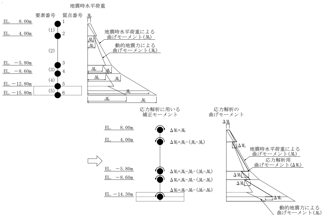
(b) 最大応答曲げモーメント iM_b と補正モーメント \Delta M_i の関係
