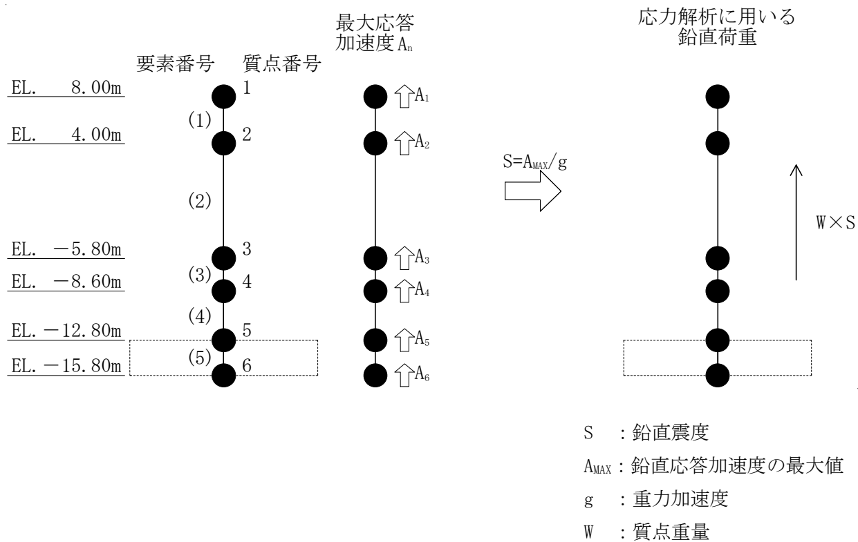
(c) 最大応答加速度 A_n と鉛直荷重 W \times S の関係
