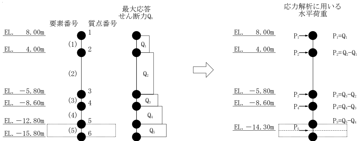
(a) 最大応答せん断力 Q_n と水平荷重 P_n の関係
