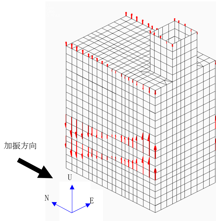
(c) 上部構造物の地震力 (補正モーメント)
